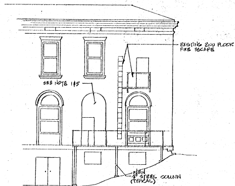
ELEVATION VIEW SCALE: 1/8" = 1'-0"
