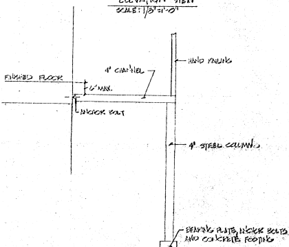
ELEVATION VIEW SCALE: 1/8" = 1'-0"
