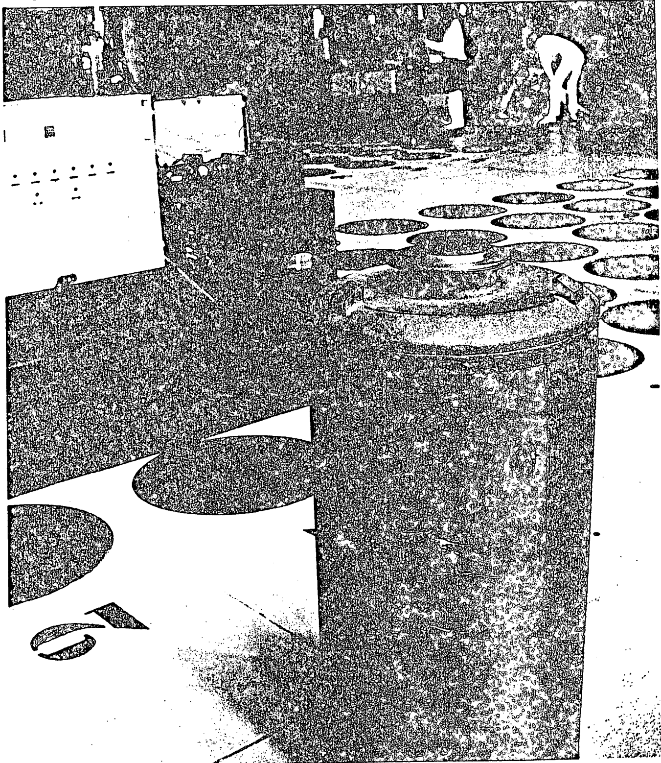
Dans ce hall de stockage sont entreposés les contenants renfermant les produits de la fusion vitrifiée. (A l'arrière-plan, l'opérateur).
