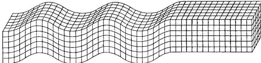
LOVE WAVE
