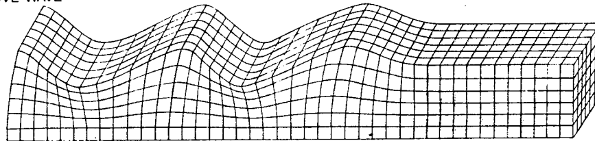
LOVE WAVE
