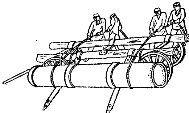
Figur 2 zeigt, wie mit Hilfe eines Hanfseiles schwere Bohr- und Futterrohre auf das Transportmittel aufgeladen werden
