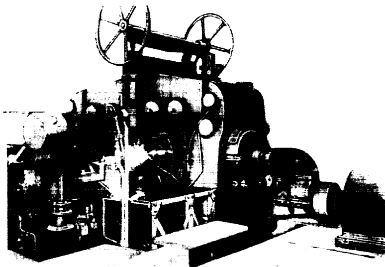
Рис. 3. Прошивной стан 5".
