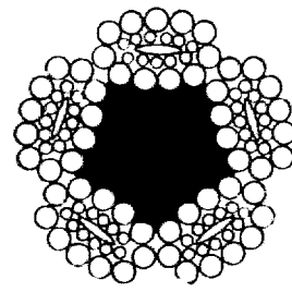
Рис. 13. Канаты овальнорядные
