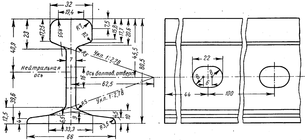
Рис. 9. Поперечный разрез и боковой вид конца узкоколейного рельса типа 11 кг/пог. м (ОСТ/ШКТП-7691/667)
