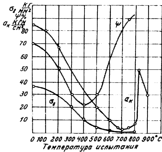
Рис. 11. Изменение механических свойств латуни Л68 в зависимости от температуры испытания.
