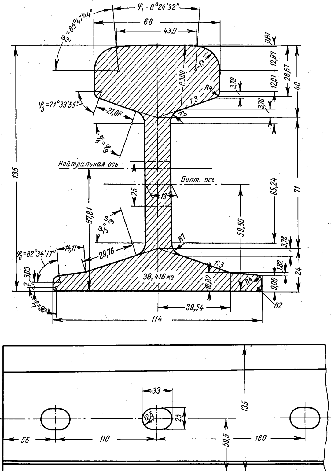
Рис. 4. Поперечный разрез и боковой вид конца рельса типа Р 38. Отверстия для болтов могут быть овальными, либо круглыми (ГОСТ 3542-47)
