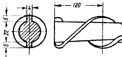
Рис. 28. Витая круглая с ребрами сталь
