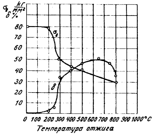
Рис. 9. Изменение механических свойств латуни Л59 в зависимости от температуры отжига.
