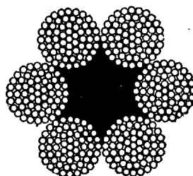
Рис. 10. Канаты круглопрядные
