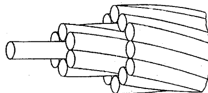
Рис. 30. Капаты с линейным касанием проволок (провода одного слоя касаются проволок смежных слоев по всей длине проволоки)
