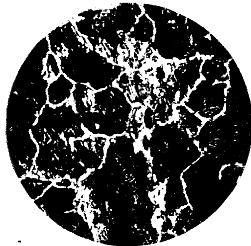
Рис. 5. Перлит и Цементит × 500
