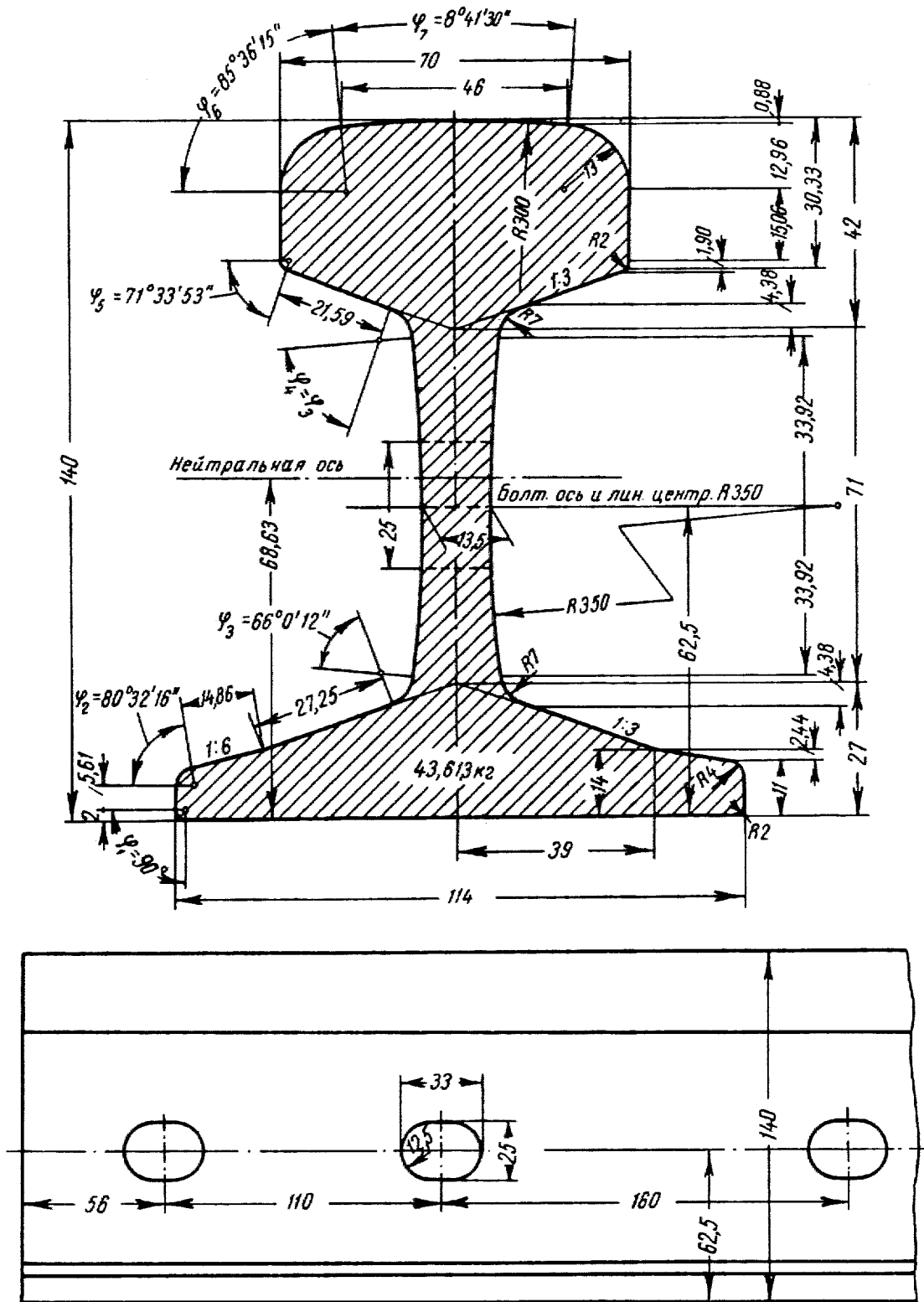
Рис. 3. Поперечный разрез и боковой вид конца рельса типа Р43. Отверстия для болтов могут быть овальными, либо круглыми (ГОСТ 3512-17)
