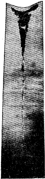
Рис. 8. Слиток обыкновенной стали торгового сорта
