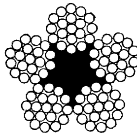
Рис. 16. Канаты пятирядные
