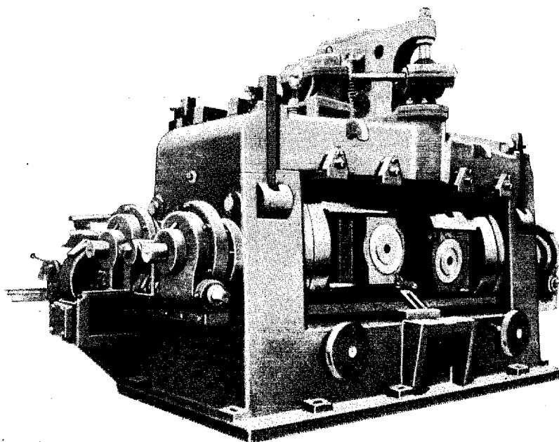
Рис. 5. Прошивной стан 8".
