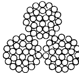
Рис. 15. Канаты трехрядные
