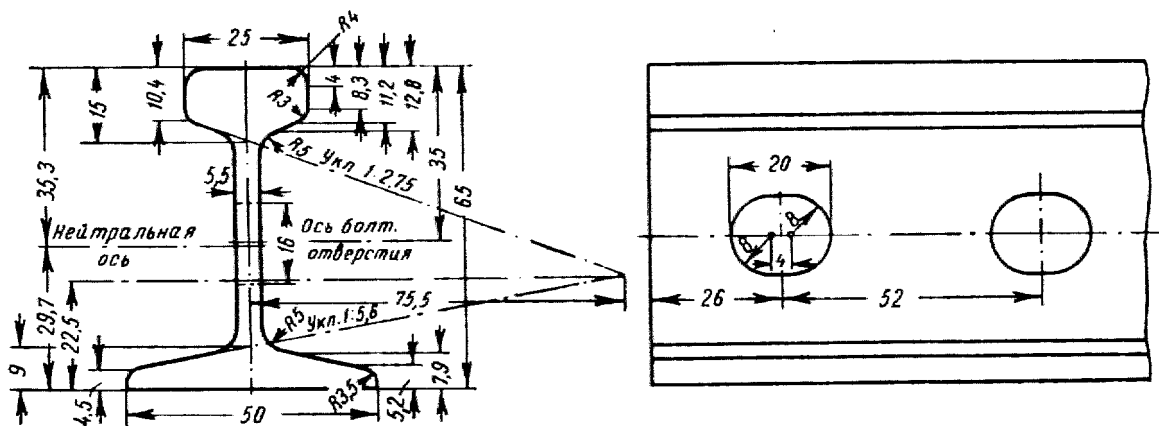
Рис. 7. Поперечный разрез и боковой вид конца узкоколейного рельса типа 7 кг/пог. м (ОСТ НКТП-7689/665)
