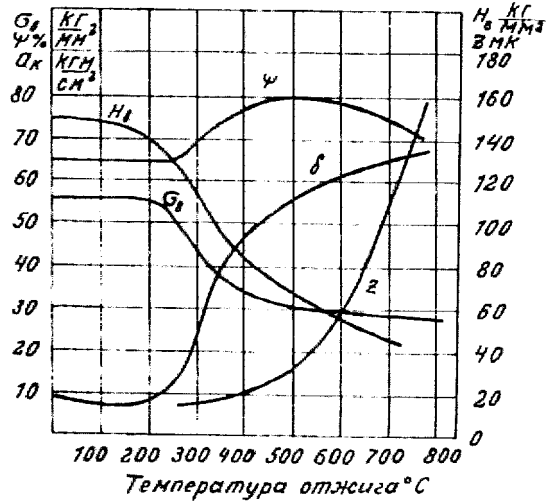
Рис. 10. Изменение механических свойств латуни Л68 в зависимости от температуры отжига (z — величина зерна в микронах).
