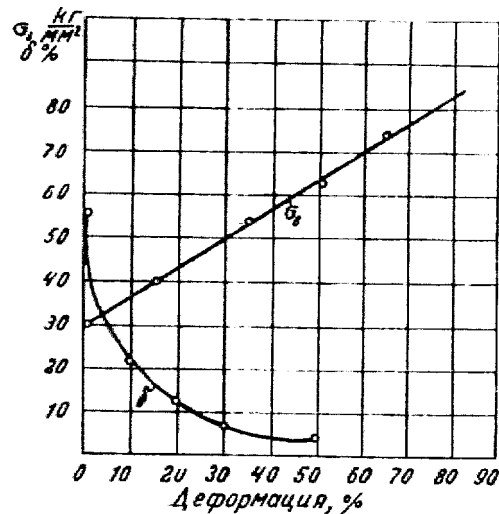
Рис. 5. Изменение механических свойств латуни Л68 в зависимости от деформации.
