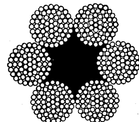
Рис. 10а. Канаты шестипрядные
