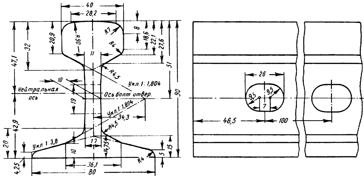
Рис. 11. Поперечный разрез и боковой вид конца узкоколейного рельса типа 18 кг/пог. м (ОСТ/НКТН-7693-669)
