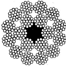
Рис. 22. Капаты с двумя слоями прядей (многослойные)
