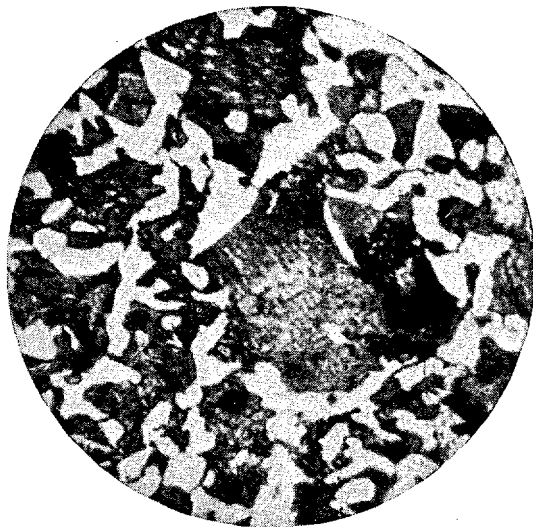
Рис. 7. Феррит и сорбит \times 500
