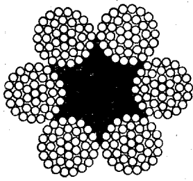
Рис. 21. Капаты с одним слоем прядей (однослойные)
