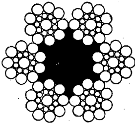
Рис. 4. Канаты из проволоки различного диаметра (компаунд)
