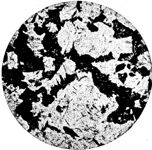
Рис. 6. Мартенсит и троостит \times 500
