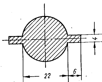
Рис. 30. Невитая круглая с ребрами сталь
