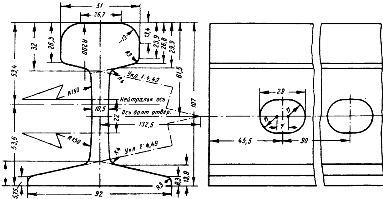
Рис. 12. Поперечный разрез и боковой вид конца узкоколейного рельса типа 24 кг/пог. м (ОСТ/НКТН-7694-670)
