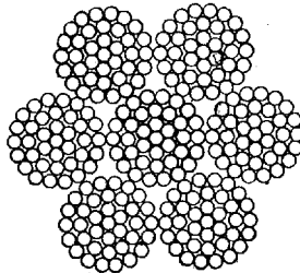
Рис. 5. Канаты с металлическим сердечником (цельнометаллически)
