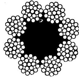
Рис. 5а. Канаты восьмипрядные
