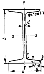
Основной сортмент двутавровых балок (ОСТ 10016-89)
