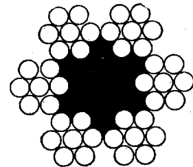
Рис. 8. Канаты с одним (центральным) сердечником
