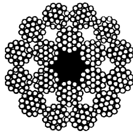
Рис. 17. Канаты восемнадцати-рядные
