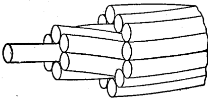
Рис. 29. Капаты с точечным касанием проволок (провода одного слоя касаются проволок смежных слоев в одной точке)
