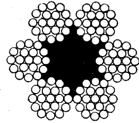
Рис. 3. Канаты из проволоки одинакового диаметра
