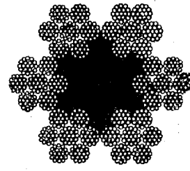
Рис. 23. Капаты тройной свивки (кабели)
