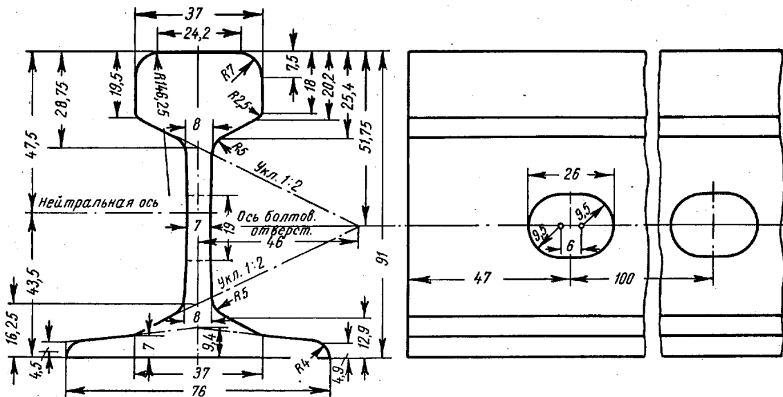
Рис. 10. Поперечный разрез и боковой вид конца узкоколейного рельса типа 15 кг/пог. м (ОСТ/ШКТП-7692/668)
