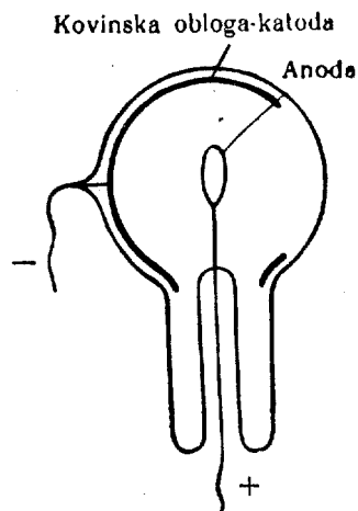
Konstrukcija fotocelice.
