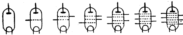
Razni tipi elektronk: dioda, trioda, tetroda, pentoda, heksoda, pentagrid in oktoda.
