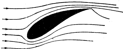
Sl. 51. — Strujanje okoli krila pri vpadnem kotu -4^\circ
