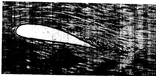
Sl. 45. — Strujanje se pričinja vrtinčiti
