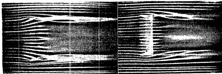
SI 54. — Robni vrtilnec krila, pogled od zgoraj
