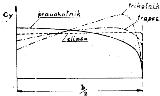
Sl. 66. — Porazdelitev [ C_y ] vzdolž razpetine za razne tlorisne oblike
