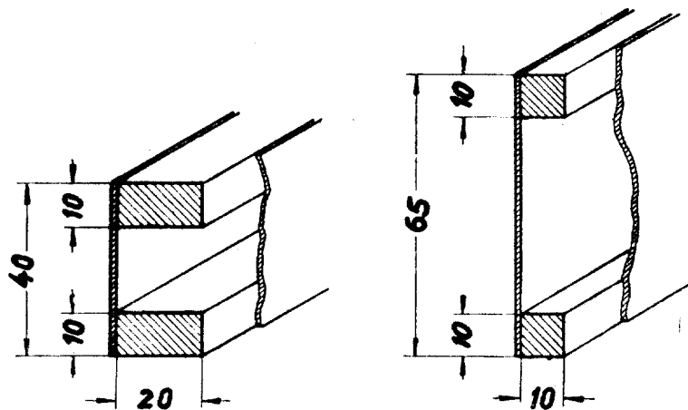
Sl. 82. — Nosilec krila: Prvi nosilec je nižji. Zato mora biti širina letev večja kot pri drugem, ki ima večjo višino
