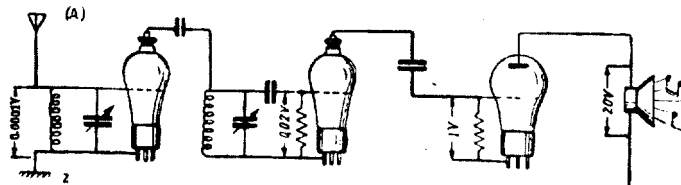
Shema radiosprejemnika SI-235.
