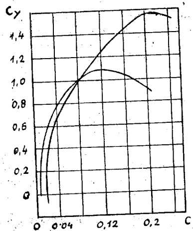
Sl. 42. Primerjava polar vzbočenega in plosimetričnega profila
