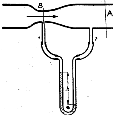
Sl. 4. — Bernollijev poskus Tok v zoženi cevi
