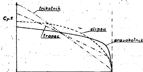
Sl. 65. — Porazdelitev ( C_y \cdot t ) vzdolž razpetine krila za razne tlorisne oblike
