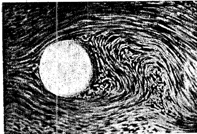
Sl. 12. — Strujanje okoli krogle
