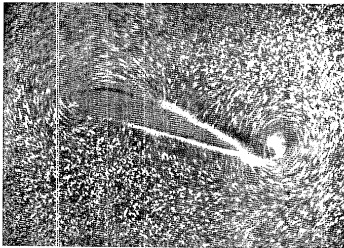
Sl. 31. — Vrtinca na krilu ob pričetku gibanja
