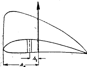
Sl. 50. — Prijemališče vzgona in nosilec krila
