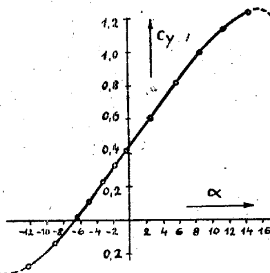
Sl. 38. — Krivulja kaže, kako se spreminja vzgonski koeficient v odvisnosti vpadnega kota
