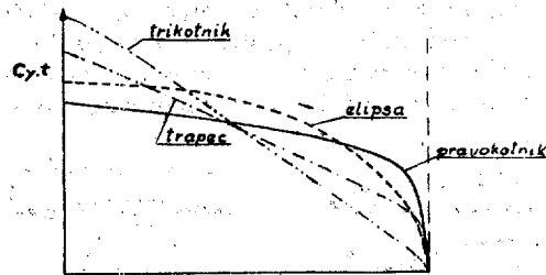
Sl. 65. — Porazdelitev ( C_y ) vzdolž razpetine krila za razne tlorisne oblike
