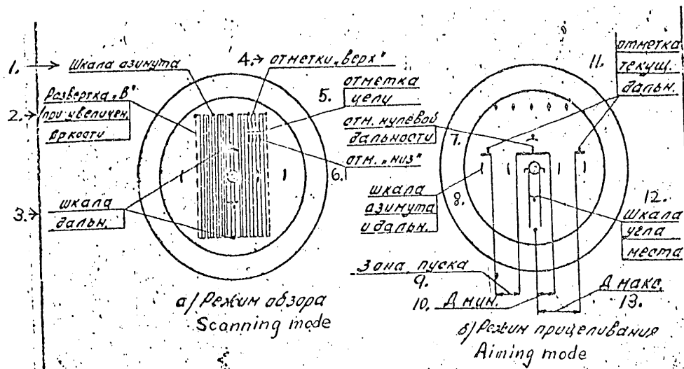
Фиг. 12 Вид экрана индикатора в режимах обзора и прицеливания.
