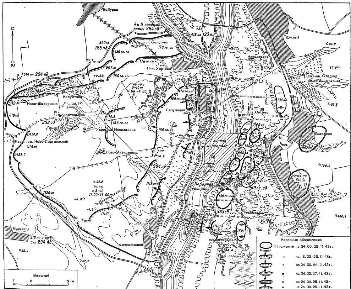
Схема 15. Боевые действия 185-го гвардейского стрелкового полка 26-29.11.43 г.
