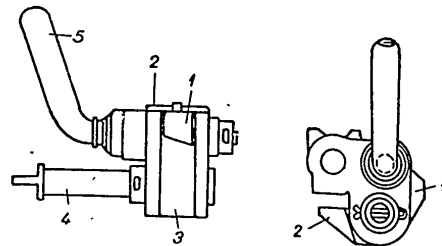
Рис. 28. Страничен механизъм: 1 — затегач, 2 — плъзгач; 3 — съединител; 4 — спиралка; 5 — ръчка
