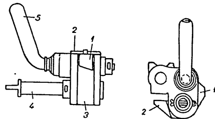
Рис. 28. Страничен механизъм: 1 — затегач; 2 — пружина; 3 — съединителя; 4 — спиралка; 5 — ръчка
