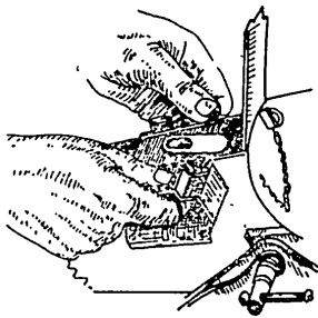
Рис. 7. Изваждане на водителя на патроните
