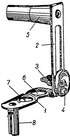
Рис. 2. Универсална диафрагма: 1 — основание; 2 — стойка, 3 — перста ключалка; 4 — подвижен окуляр; 5 — тръбичка за закрепване към пушката; 6, 7 — кръгли отвори за закрепване към картчницата; 8 — шип за закрепване на диафрагмата към старите образни тежки картчници
