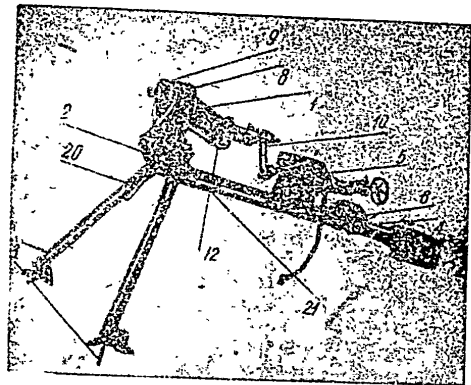
Рис. 29. Лафет-тринога на тежка картечница система Максим обр. 1908, 1909 г.: 1 — вилка; 2 — глава; 3 — предни крака; 4 — заден подвижен крак; 5 — повдигателен механизъм и лостове; 6 — възглавничка; 7 — седалнице; 8 — цапфа; 9 — кръгова чашкообразна цапфа; 10 — дъгова площадка; 11 — кутия за запасния затвор; 12 — ключалки на страничните крака; 13 — тръба
