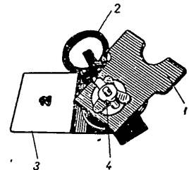
Рис. 1. Показна мушка: 1 — горна пластинка с прорез; 2 — средна пластинка с мушка; 3 — долна пластинка с мерни точки; 4 — винт
