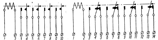
Abb. 1. Innenschaltung des Relais RUo-700 mit 4 Arbeitskontakten (Ausführung als RUo-704)
