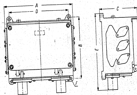
Abb. 2 Verteilungsschränke Typen KVA 8012-13
