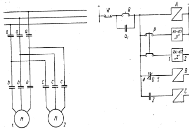
Schaltbild 3
