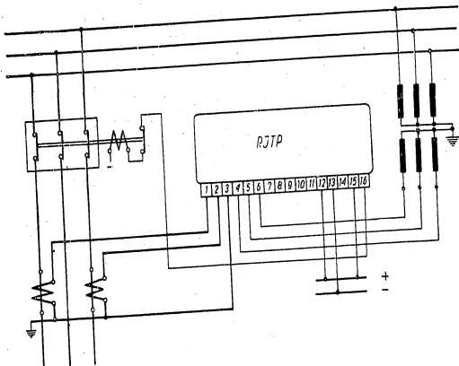
Abb. 1. Anschliessen des Relais der Typ RITP als Überstrom-Richtungsschutz einer Leitung.
