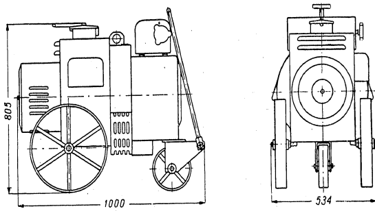
Abb. 4. Massbild des Schweissumformers EW-21u
