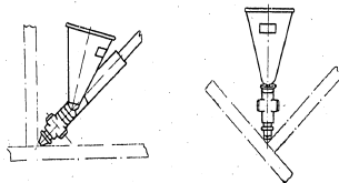
Abb. 4 Schweissung von Winkelnähten
