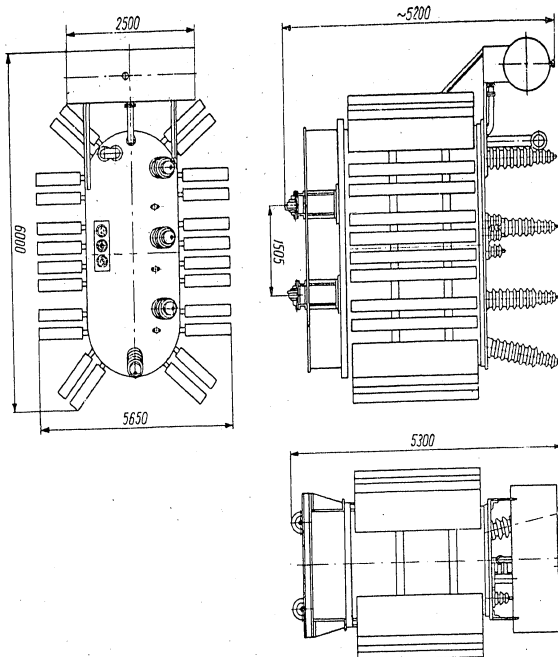
Masskizze
