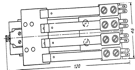
Abb. 5. Abmessungen des Relais RUo-700
