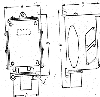
Abb. 1 Verteilungsschränke Typen KVA 8001-11
