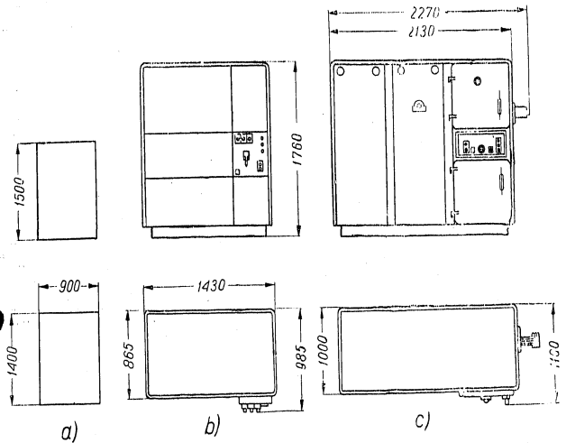
Abb. 3. Aussenmasse des Mittelfrequenz-Induktionsofens Type PIS-20: a — Transformator, b — Gleichrichter, c — Generator
