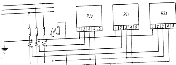
Abb. 1. Anwendungsbeispiel des Relais R1z zum Schutz einer Dreiphasen-Hochspannungsleitung.
