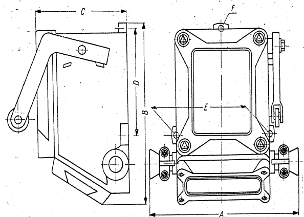
Abb. 5. Signalgeber Typ KFS 1252. Masszeichnung.
