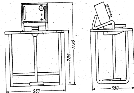
Massbild
