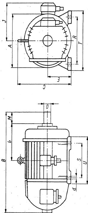
MASSBILD
