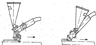
Abb. 3 Auftragschweissung
