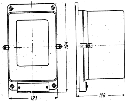
Abmessungen des Relais GSM
