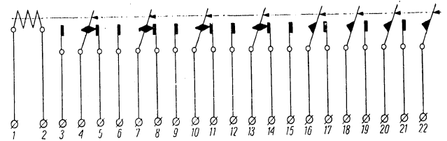
Abb. 3. Innenschaltung des Relais RUo-700 mit dem Kontaktsatz "4 p + 4 z" (Ausführung als RUo-708)
