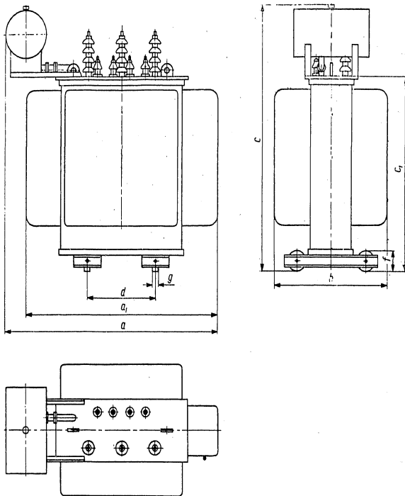
Masskizze
