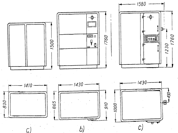
Abb. 4. Aussenmasse des Mittelfrequenz-Induktionsofens Type PIS-50: a — Transformator, b — Gleichrichter, c — Generator
