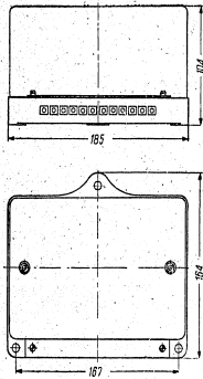
Bild 5 Masszeichnung des Relais RA-411/421
