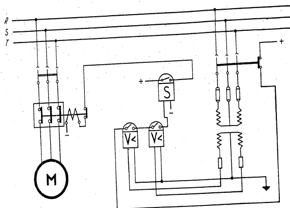
Abb. 1 Schaltsystem mit zwei Relais REp-4 plus Zeitrelais S.
