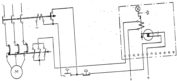
Abb. 1. Anwendungsbeispiel für das Relais RA-412/422.
