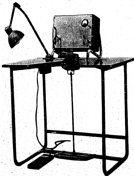
Abb. 2. Hochfrequenz-Schweißgerät Typ ZDK-01-C.
