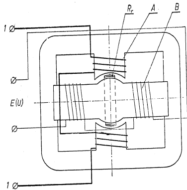
Abb. 1 Konstruktions-Schema des Relais RP-1
