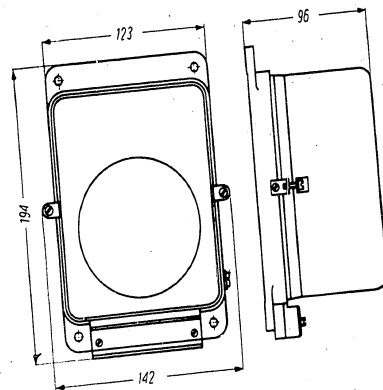
Abb. 4 Massbild des Relais Typ RI-4
