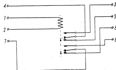
Abb. 2. Schaltbild des Relais RU-500
