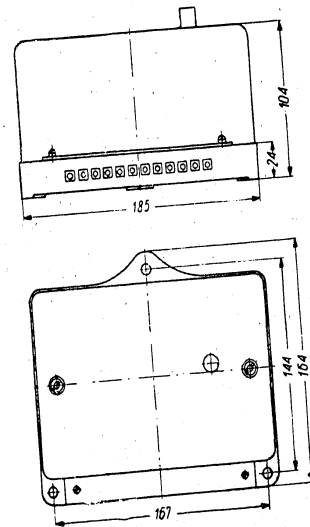
Abb. 3. Masskizze des Relais
