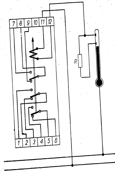
Abb. 1 Elektrisches Schema des RES Relais
