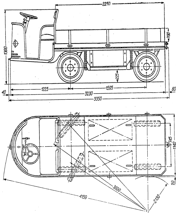
Masszeichnung
