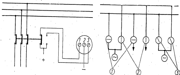
Abb. 1. Anschluss des Anzeigers Typ WP zum Anzeigen der Stellung des zugeordneten Schalters.
