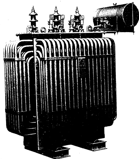
Transformator mit Rohrkasten
