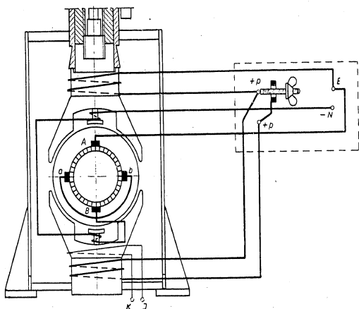
Abb. 2. Aufbauskinne des Schweissgenerators
