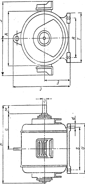
MASSBILD
