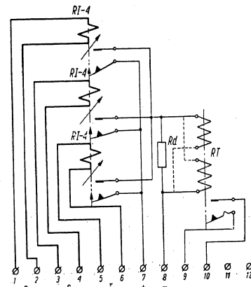
Abb. 4. Schaltschema des Relais RI-3
