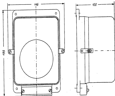
Abb. 3 Masse des Relais REp-4
