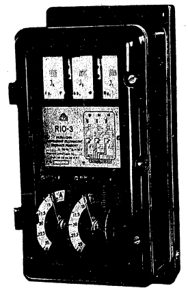
Überstromrelais mit unverzüglicher Auslösung Type Rio
