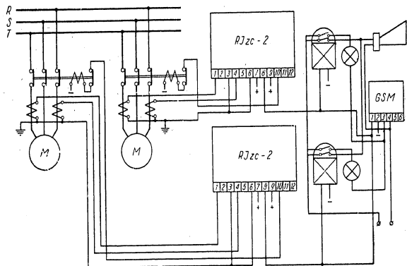
Abb. 1. Anwendung des Blinkrelais zur Leuchtsignalisation beim Überstromschutz zweier Motoren
