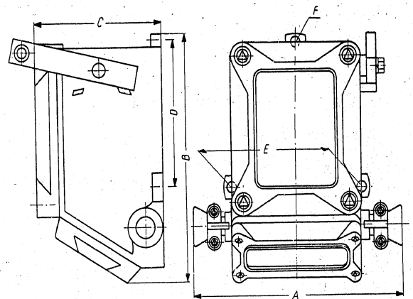
Abb. 1. Signalgeber Typ KFS 1212. Masszeichnung
