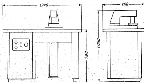
Massbild
