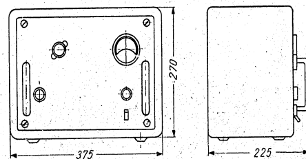
Massbild
