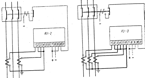
Abb. 1. Sicherungs-Schema bei Anwendung des Relais RI-2
