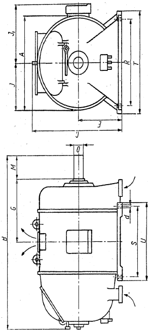
Motoren der Typenreihe SYUf (Grösse 18 - 20) Betriebsspannung 3000 V und 6000 V, 2 und 4 - polig
