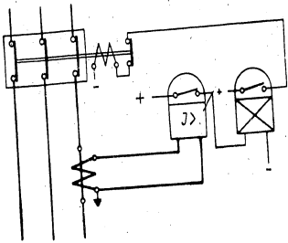
Abb. 1. Anwendungsbeispiel des Relais RI-4 als unverzögerter Überstromschutz.
