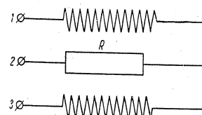
Abb. 4. Schaltung des Schalterstellungsanzeigers WP mit Vorwiderstand.
