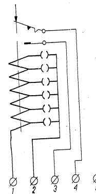
Abb. 2. Schaltschema des Relais R1z
