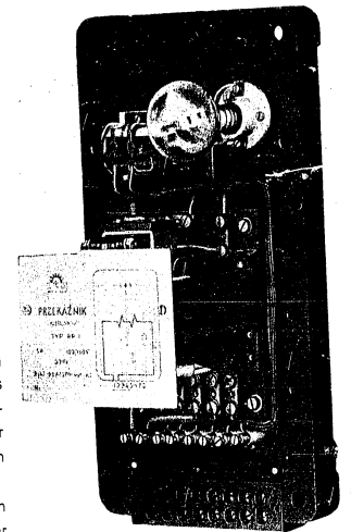
Relais RP-1 ohne Gehäuse
