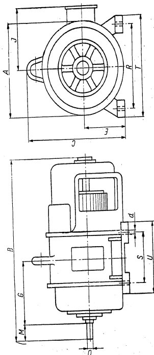
MASSBILD
