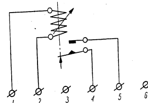
Abb. 2 Elektrische Schaltung des Relais REp-4
