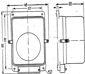
Abb. 2 Abmessungen des Relais REn-4
