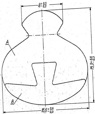
Zeichn. 2. Stahl-Aluminium-Fahrdraht Type S-80/175 A-Aluminiumteil B-Stahlteil
