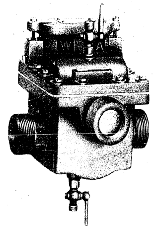
Buchholzrelais Type RB-1, RB-2, RB-3
