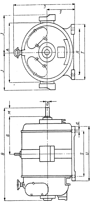
MASSBILD
