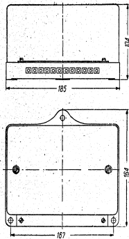
Bild 5 Masszeichnung des Relais RA-411/421
