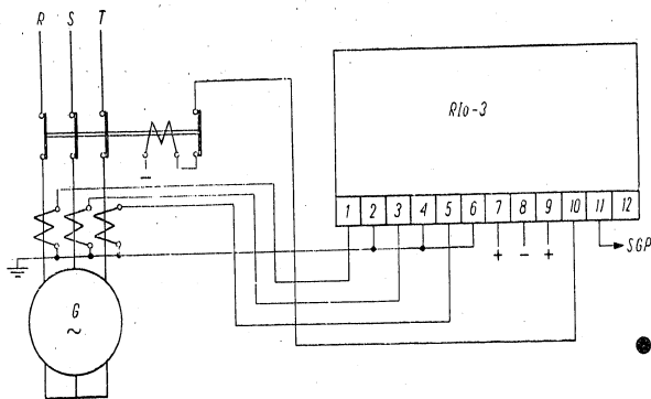
Abb. 1. Beispiel der Anwendung des Relais Rlo
