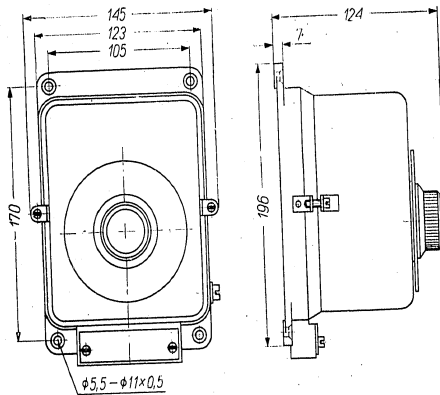
MASSZEICHNUNG
