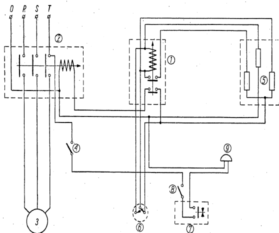
Abb. 1. Verwendung des Relais RU-520 zur automatischen Steuerung einer hydraulischen Presse
