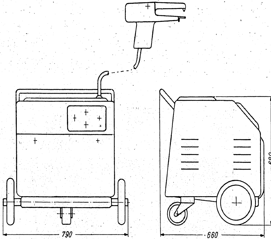
Massbild
