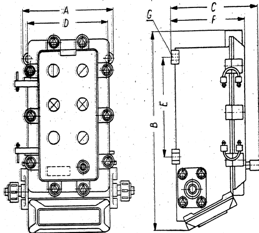
Abb. 3 - Leuchttafel Type KDA 3263 Masszeichnung
