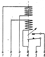
Abb. 1. Überspannungsrelais REn-4 Innenschaltung
