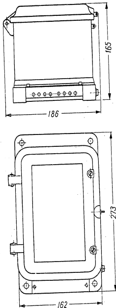
Abb. 5 Massbild des Relais mit Gehäuse
