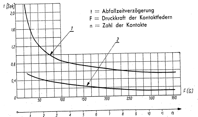
Abb. 4. Kennlinien des Relais RUo-700 1 t (F) bei \delta 0,1 mm (Kurve 1) und \delta 0,2 mm (Kurve 2).
