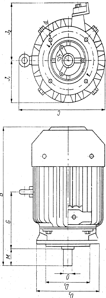
MASSBILD
