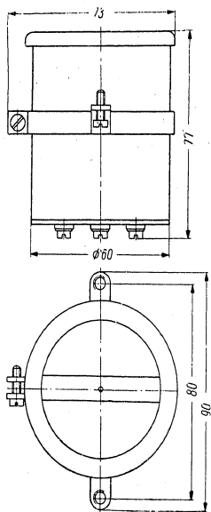
Abb. 5. Massskizze
