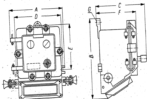
Abb. 1 - Leuchttafel Type KDA 3223 Masszeichnung
