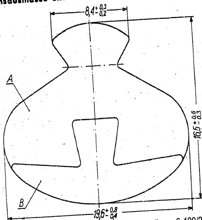
Zeichn. 1. Stahl-Aluminium-Fahrdraht Type S-100/215 A-Aluminiumteil B-Stahlteil
