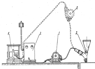
Abb. 2. Schemazeichnung der Schweißanlage
