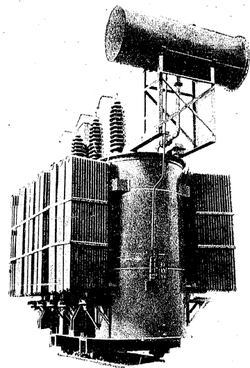
Drehstrom-Öltransformator in Freiluftausführung Type TON-16000/110
