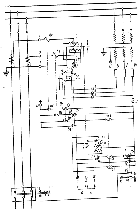
Abb. 3. Erweitertes Prinzipschaltbild; Sicherungsschutz mittels Relais Typ RITP.
