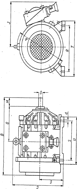
MASSBILD
