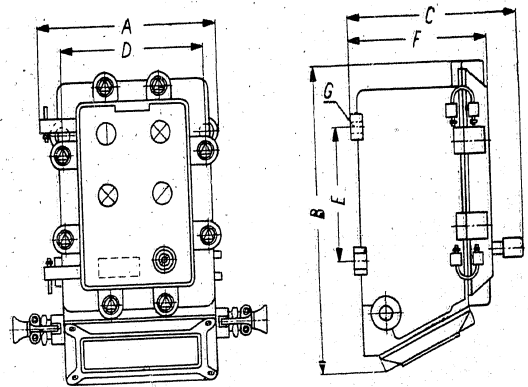
Abb. 2 - Leuchttafel Type KDA 3243 Masszeichnung
