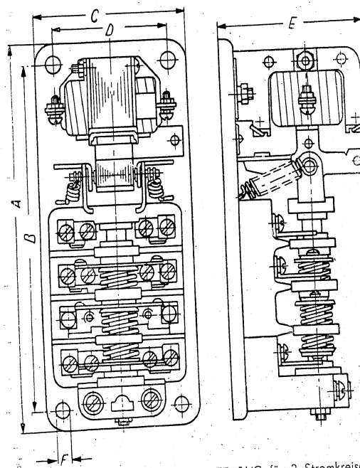
Abb. 1. Massbild des Relais PEZ 54/C für 3 Stromkreise
