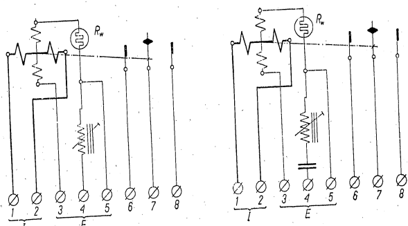
Abb. 3 Prinzipschaltung des Relais RPb-1 und RPM-1
