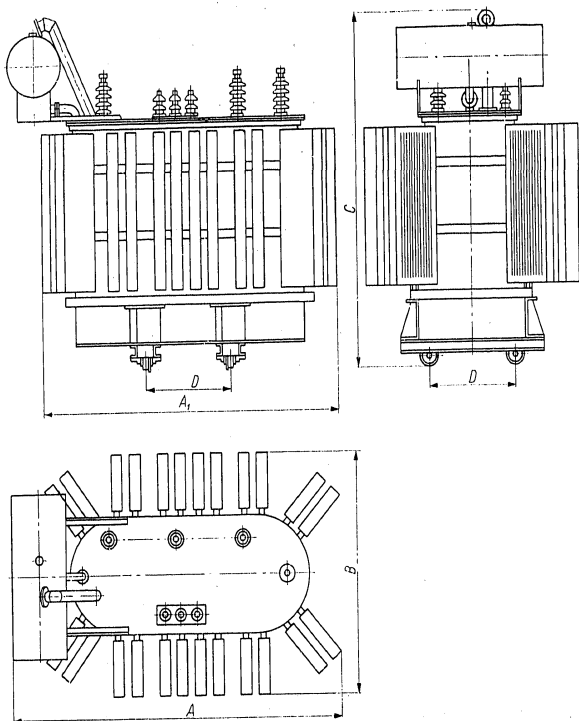
Masskizze
