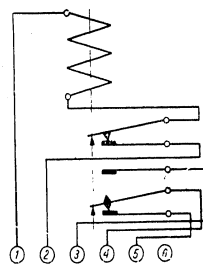
Abb. 2. Innenschaltung des Relais GSM
