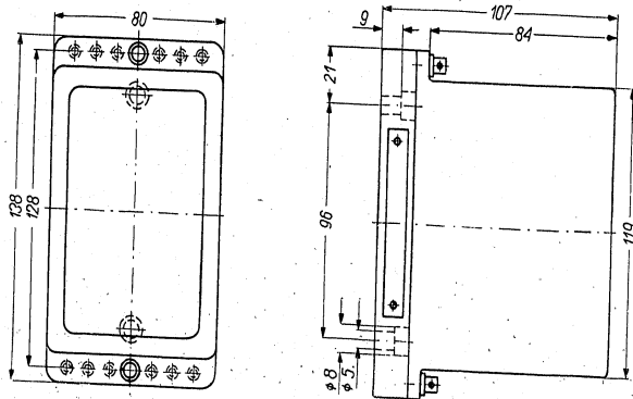
Abb. 2 Maßzeichnung
