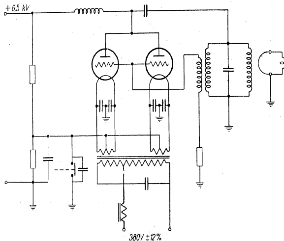
Abb. 2. Schaltschema des Mittelfrequenz-Induktionsofens
