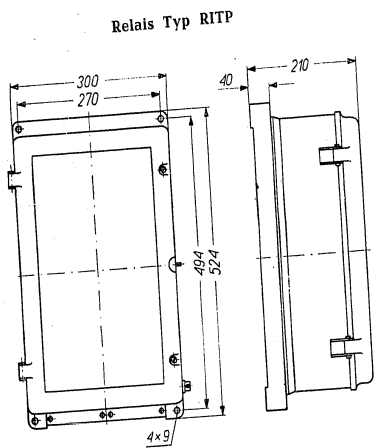
Abb. Nr. 4. Ausmasse des Relais
