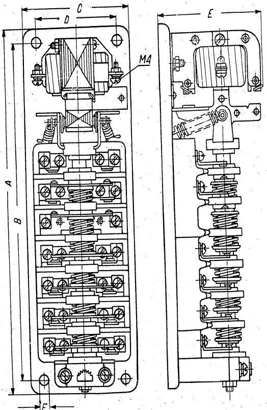
Abb. 2: Massbild des Relais PEZ 54/C für 6 Stromkreise
