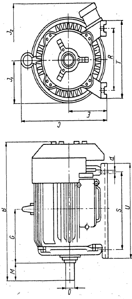
MASSBILD
