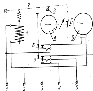
Schaltbild des Relais
