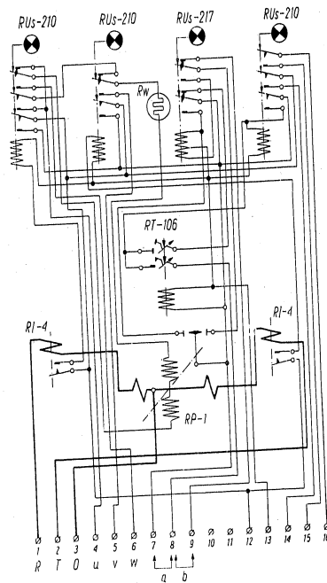
Abb. 2. Schaltschema des Relais Type RITP.
