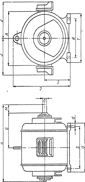
MASSBILD
