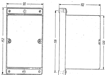
Massbild
