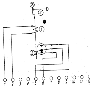
Abb. 2. Prinzipschaltbild des Relais RA-412/422.
