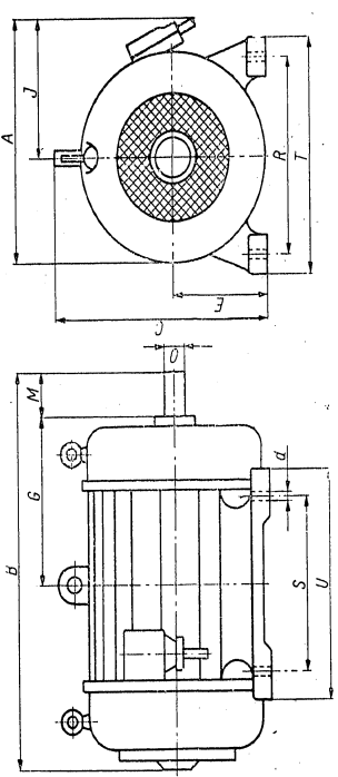
MASSBILD
