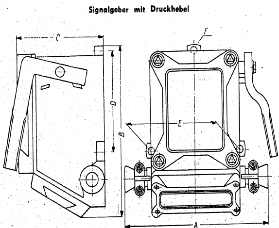
Abb. 4. Signalgeber Typ KFS 1232. Masszeichnung.
