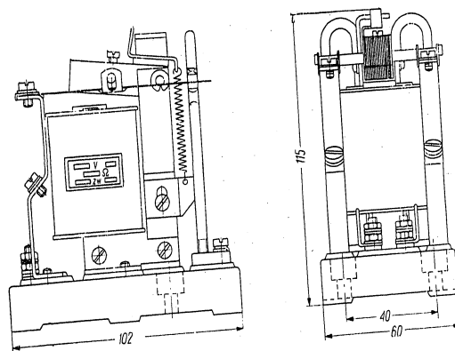
Abb. 3. Masskizze des Relais RU-500
