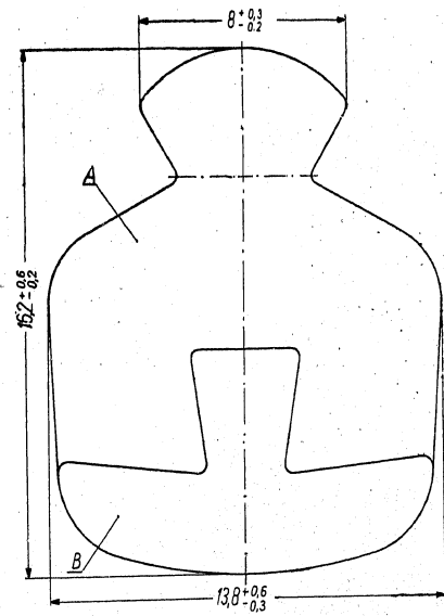
Zeichn. 3. Stahl-Aluminium-Fahrdraht Type T-80/175 A-Aluminiumteil B-Stahlteil
