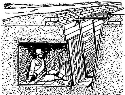
Фиг. 46. Подбрустерна ниша
