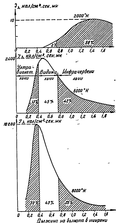
Фиг. 29. Спектрално разпределение на енергията за различни повърхностни температури на огненото кълбо
