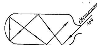
Фиг. 24. Модел на абсолютно черно тяло
