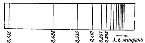
Фиг. 22. Линейен спектър на водорода във видимата и в близката до ултравиолетовата част на спектъра
