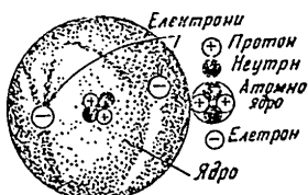
Фиг. 1. Строеж на хелиевия атом (схема)
