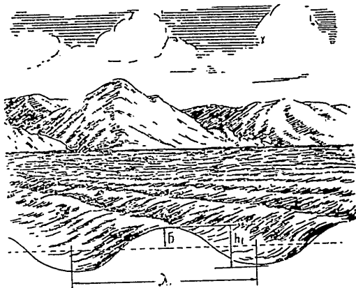
Фиг. 14. Вълни по повърхността на водата : \lambda — дължина на вълната, h_1 — височина на вълната, B — амплитуда
