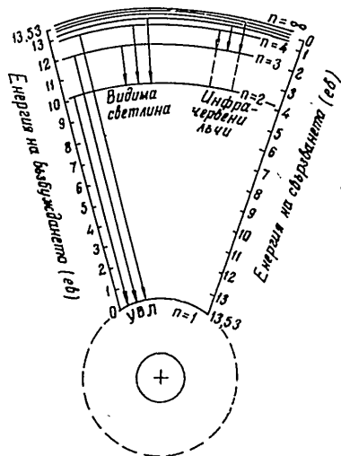
Фиг. 23. Схема на енергичните нива на водородния атом
