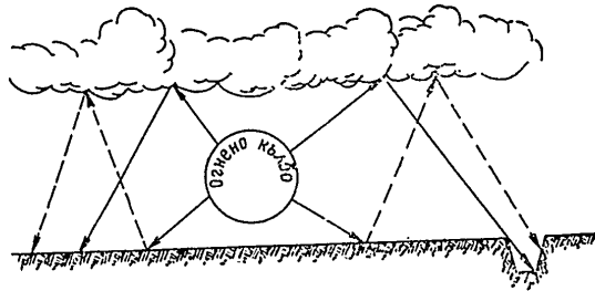
Фиг. 34. Схема за отразяване на светлинното излъчване от облаците
