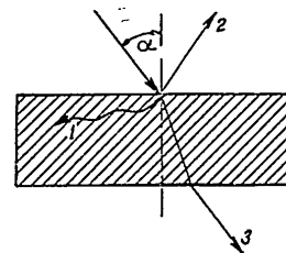
Фиг. 36. Схема за разпределение на светлинната енергия (светлинния импулс), падаща върху тялото: 1 — погълната от тялото; 2 — отразена; 3 — преминала през тялото
