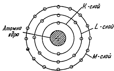
Фиг. 20. Схема за строежа на електронната обвивка на атома
