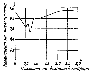
Фиг. 37. Изменение коефициента на поглъщането за човешката кожа в зависимост от дължината на светлинната вълна
