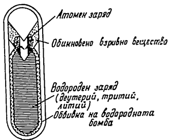
Фиг. 3. Принципна схема на водородната бомба
