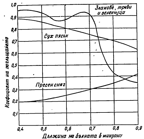
Фиг. 38. Изменение на коефициентите на поглъщане за различните земни покривки в зависимост от дължината на вълната
