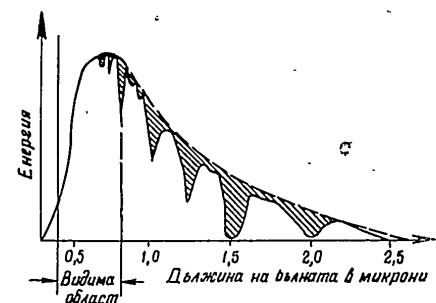
Фиг. 26. Излъчвателен спектър на слънцето. В местата, означени с шрихи, слънчевата енергия се поглъща в атмосферата.
