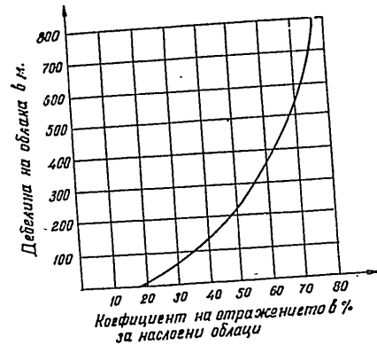
Фиг. 35. Зависимост между отразените светлинни излъчки и дебелината на облаците
