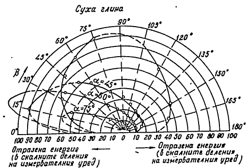
Фиг. 43. Разпределение на отразената енергия в пространството при различни ъгли на падане ( \alpha ) и ъгли на отражение ( \beta ) на лъчите
