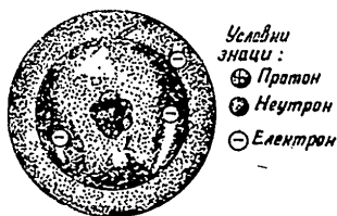
Фиг. 19. Схема за строежа на литиевия атом
