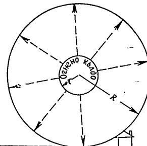
Фиг. 30. Ако имаме загуба на енергия в атмосферата, цялата излъчена от огненото кълбо енергия ще премине през сфера с радиус R .
