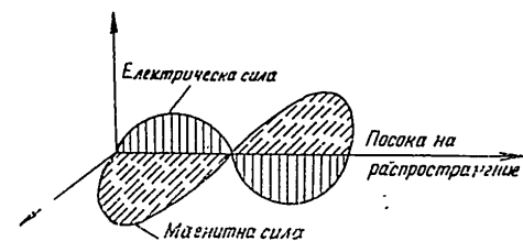
Фиг. 16. Електромагнитна вълна
