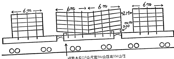
原本成組連裝法裝載略圖
