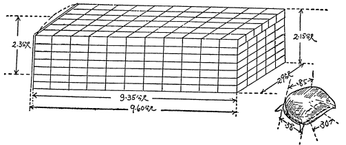
濟南局巢縣站敞車裝稻子 (增載 33 噸) 略圖 (乙)
