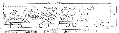
十九、衡陽局黃埔站用平車二輛裝汽車五輛的圖
