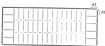
第7層兩端縱置平放 5 \times 2 = 10 件，中間五層平放 15 \times 3 = 45 件，共計55件，互相擠壓，長度尚長收縮。
