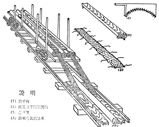
雨天裝原木略圖
