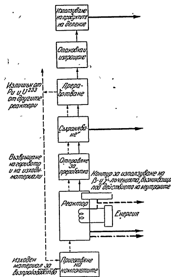
Фиг. 1. Схема на проектирания енергичен реактор с твърдо гориво, предназначено също за използване като източник на лъчение
