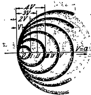
Фиг. 15. Разпространение на смущения при скорост на източника, произвеждащи смущенията, V равна на скоростта на звука a ( V=a )
