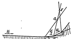
Фиг. 18. Обтичане на вътрешен тъл ъгъл от свръхзвуков въздушен поток
