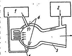
Фиг. 137. Принципа схема на атомни реактивен двигател без реактор:
