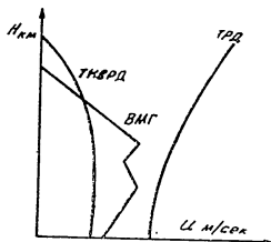
Фиг. 125 Изменение на максималната вертикална скорост на самолети с бутални (ВМГ), турбо-реактивни (ТРД) и течно-ракетни (ТРД) двигатели в зависимост от височината на полета
