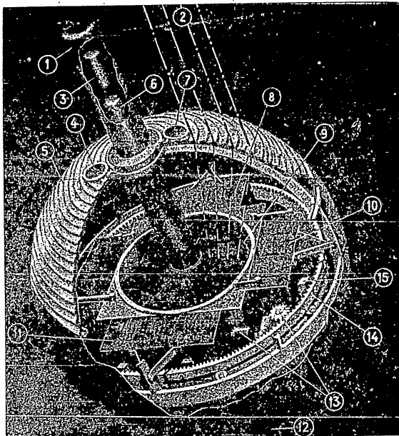
Фиг. 134. Принципа схема на изкуствен спътник на земята:
