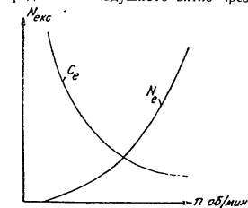
Фиг. 114. Оборотна характеристика на турбовитловия двигател
