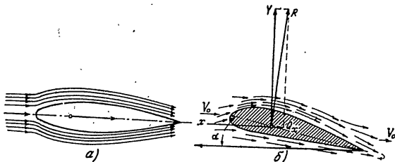
Фиг. 29. Сили, действащи на крилото
