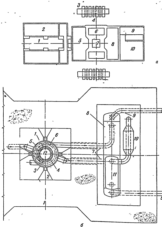
Фиг. 4. Схема на реактор с двойно предназначение:
