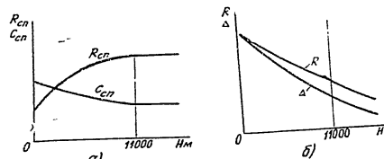
Фиг. 110. Височинна характеристика на турбо-реактивния двигател
