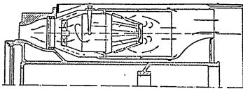
Фиг. 102. Блоквата горивна камера
