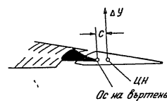
Фиг. 41. Осева компенсация
