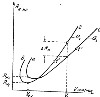
Фиг. 121. Влияние на изменението на полетното тегло на самолет с реактивен двигател върху необходимата теглителна сила за хоризонтално летене
