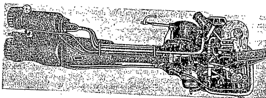
Фиг. 85. Течно-ракетен двигател с две горивни камери
