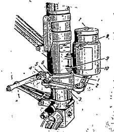
Фиг. 68. Общ вид на демперен апарат. 1) пръстен с лост; 2) лост; 3) промехдулционно звено; 4 и 6) болтове; 5) прорез; 7) инертен за зареждане на компресирана течност; 8) индикатор; 9) кронштейн; 10) демпер
