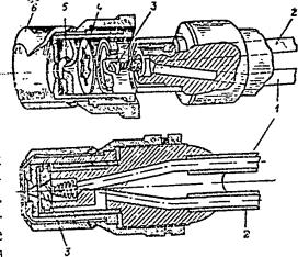
Фиг. 105. Двуканална горивна форсунка: 1 — пускова тръбичка, 2 — основна тръбичка, 3 — завихрител, 4 — пластинчат завихрител, 5 — сопло, 6 — въздушен капачок
