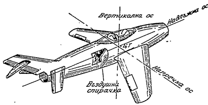
Фиг. 48. Въздушна спирачка и оси на самолета
