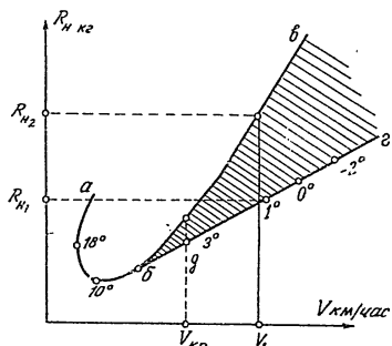
Фиг. 119. Влияние на свиваемостта на въздуха и ъвълновото съпротивление върху необходимата теглителна сила R_H за хоризонтален полет
