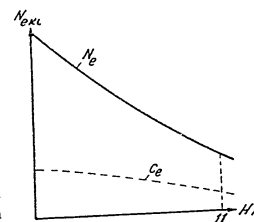
Фиг. 116. Височинна характеристика на турбовитловия двигател
