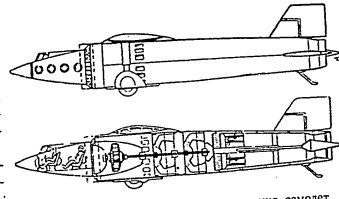
Фиг. 92. Принципа схема на реактивния самолет „Капрони-Кампини“
