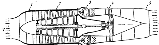
Фиг. 93. Принципа схема на турбо-реактивен двигател с осев компресор: 1 — входящ канал; 2 — осев компресор; 3 — горивна камера; 4 — газова турбина; 5 — реактивно сопло
