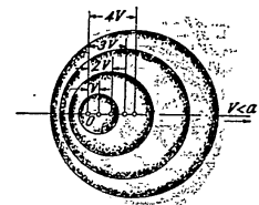
Фиг. 14. Разпространение на звукови вълни при скорост на източника, по-малка от скоростта на звука (V < a)
