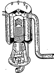
Фиг. 5. Резервоар на активната зона на реактор с бързи неутрони с натриево охлаждане
