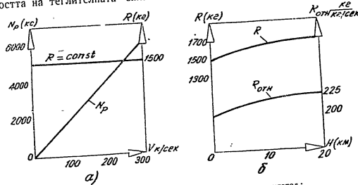
Фиг. 81. Характеристики на течен ракетен двигател: а — скоростна характеристика; б — височинна характеристика
