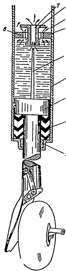
Фиг. 65. Принципно устройство на амортизационна стойка
