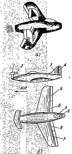
Фиг. 25. Особени схеми на самолети: а — самолет „без опашка“; б — самолет тип „патница“.
