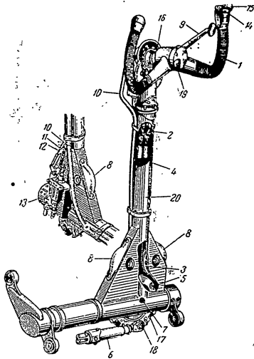
Фиг. 52. Волан:
