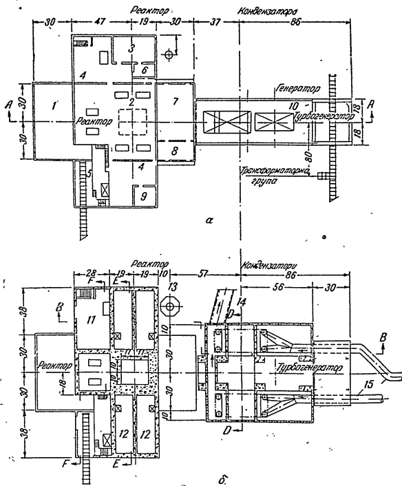
Фиг. 2. Горизонтални разрези на сградата за реактор с топлинни неутрони с водно охлаждане (всички размери на фигурата са дадени във футове): а — разрез по етажа, в който се намира звъната за управление; б — разрез по нивото на земята; в) разрез под нивото на земята 1 — защитни люкове, водещи към спомагателните съоръжения; 2 — защитни люкове, водещи към помпите и вентилите; 3 — склад за дозиметричните и ремонтните съоръжения; 4 — преградка; 5 — помещение за пълнене; 6 — лаборатория; 7 — помещение за управление; 8 — помещение на обслужващия персонал; 9 — хранилище за пресните топлоотдаващи елементи; 10 — релси на порталния кран; 11 — ремонтна работилница за електрическите съоръжения; 12 — парогенератори; 13 — тръба; 14 — тръба с вътрешен диаметър 10 фута; 15 — стоманена тръба с вътрешен диаметър 6 фута;
