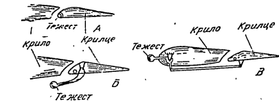
Фиг. 45. Тегловна компенсация : А — тежестта е поставена в крилото; Б и В — тежестта е извън крилцето
