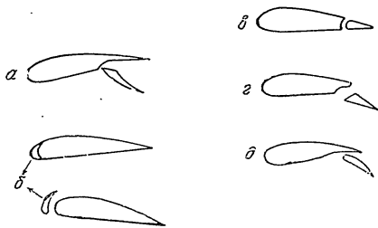
Фиг. 47. Механизация на крилото: а — клапани, б — предкрилки; в — задкрилка без междинна, г — задкрилка с междинна; д — подкрилка
