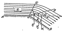
Фиг. 17. Обтичане на външен тъл ъгъл от въздушен поток със свръхзвукова скорост
