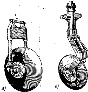
Фиг. 67. Самолетни колела. а — основно колело; б — резервно колело.
