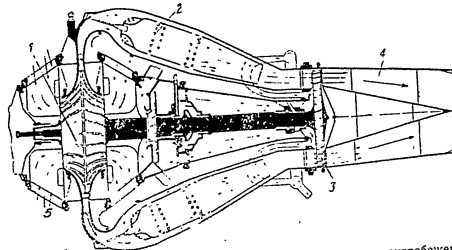
Фиг. 94. Принципа схема на турбо-реактивен двигател с центробежен компресор: 1 — центробежен компресор; 2 — горивна камера; 3 — турбина; 4 — реактивно сопло; 5 — входящо устройство
