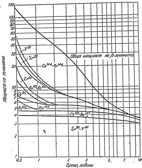
Фиг. 5. Изменение по време на мощността на потока от β-частици, изпускани от продуктите на деление и от отделни най-важни изотопи, влизащи в състава им: Мощността на лъчението се определя като произведение от броя на изпускваните β-частици и тяхната енергия. Времето се изчислява от момента на излизане на продуктите на деление от реактора
