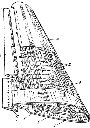
Фиг. 37. Моноблоково крило: 1 — надлъжник; 2 — стрингер; 3 — ребро; 4 — обшивка; 5 — крило; 6 — покривка
