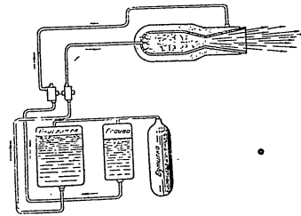
Фиг. 79. Принципа схема на течно-ракетен двигател с бутилково подаване на топливото
