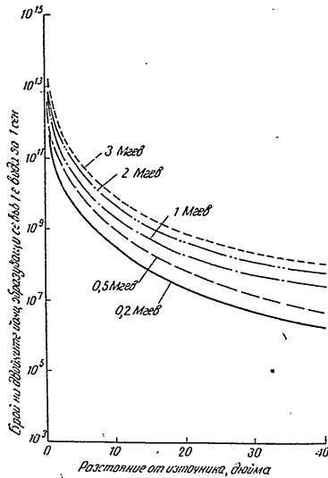
Фиг. 10. Брой на образуваните двойки йони в 1 л вода като функция на разстоянието от източник с активност 1 кюри:
