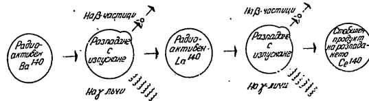
Фиг. 2. Схематично изображение на верига радиоактивни превръщания
