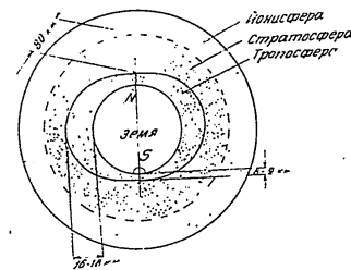
Фиг. 12. Строеж на атмосферата
