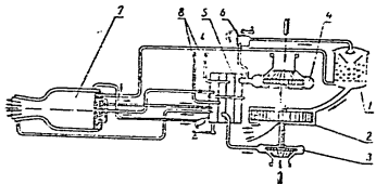
Фиг. 80. Принципа схема на течно-ракетен двигател с помпено подаване на топливото: 1 — парогазгенератор; 2 — турбина, привързана в действителност за гориво и окислител; 3 — помпа за горивото; 4 — помпа за окислителя; 5 — агрегат за разпределение налягането на горивото и окислителя; 6 — регулатор на налягането на парогаса; 7 — горивна камера; 8 — изпускател на горивото и въздуха
