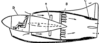
Фиг. 87. Схема на реактивния с моет „Ледюк-010“: А — направлени пламъци; В — форсулки; С — канали за захранване на горивото; D — обвивката кабината
