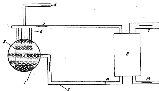
Фиг. 7. Схема, илюстрираща извършваните в реактор с течен топлоносител основни измервания:
