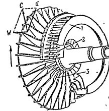
Фиг. 96 Центробежен компресор: 1 — неподвижен направляващ апарат; 2 — направляващи лопатки; 3 — подвижен (въртящ се) направляващ апарат
