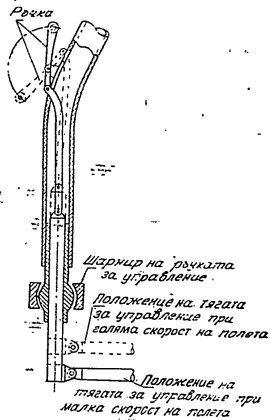
Фиг. 55. Ръчен лост с изменяемо число на предаването
