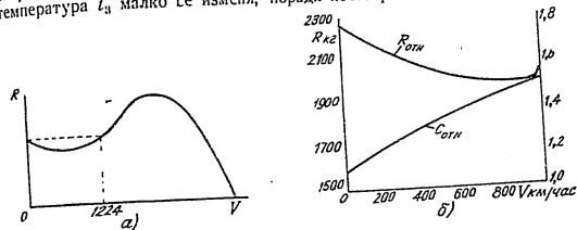
Фиг. 109. Скоростна характеристика на турбо-реактивния двигател
