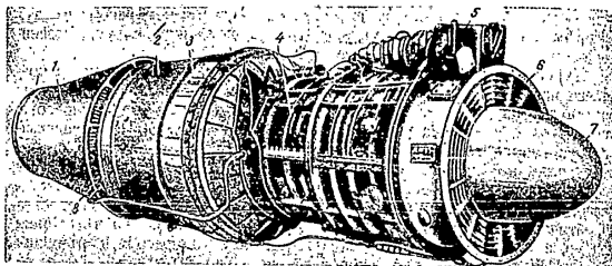
Фиг. 118. Общ вид на двуконтурен турбо-реактивен двигател: 1 — реактивно сопло; 2 — кожух на горивната камера; 3 — форсунка; 4 — кожух на компресора; 5 — квартал на преноса на агрегатите; 6 — вход за въздуха в компресора; 7 — обтикател; 8 — вход на въздуха за компресора във втория контур
