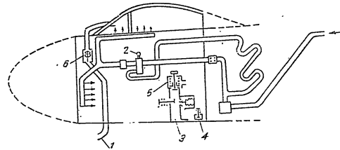
Фиг. 62. Принципно схема на вентилационна кабина: 1 — вентилационна уредба; 2 — кран за подхранване на кабината с въздух; 3 — регулатор на налягането; 4 — предпазителен клапан; 5 — клапан за обратна разлика в налягането
