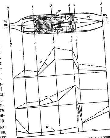
Фиг. 95. Схема на турбо-реактивен двигател с неговите параметри
