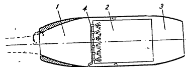
Фиг. 86. Принципа схема на правопоточен въздушно-реактивен двигател: 1 — дифузор, 2 — горивна камера, 3 — сопло, 4 — форсунки за въпръскване на горивото
