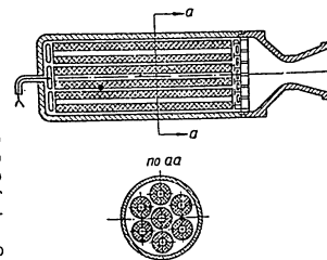
Фиг. 76. Принципа схема на барутен ракетен двигател
