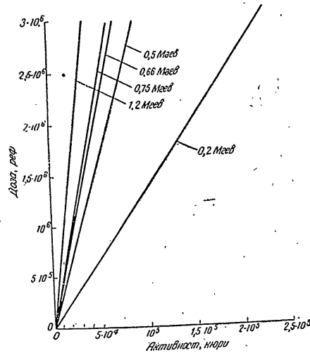
Фиг. 1. Графики за преминаването от активността на източника, изразена в единица кюри, към дозата на \gamma -лъчението в реф за 1000 фунта вещество, облъчвано на ден: Коефициентът на използване енергията на \gamma -лъчите се приема равен на 63% при 20-часов работен ден
