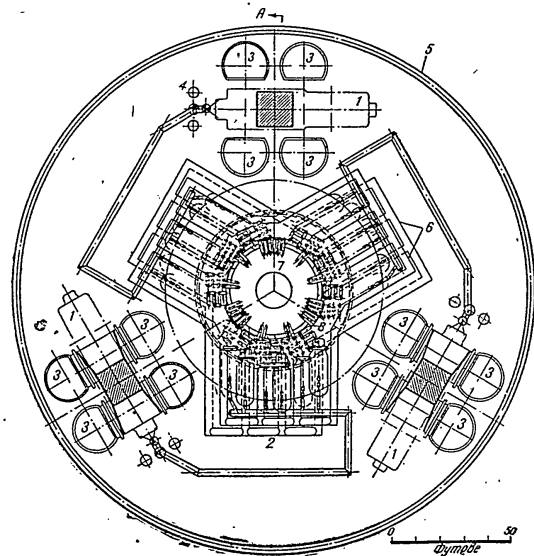
Фиг. 9. План за разположението на реактор с течен топлоносител: 1 — турбина мощност 80 000 кил; 2 — шест парогенератора; 3 — кондензатор; 4 — помпи за кондензата; 5 — стена на сградата с диаметър 217 фута; 6 — бестонна защита; 7 — реактор; 8 — колектори на тежката вода
