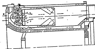
Фиг. 101. Пръстеновидна горивна камера
