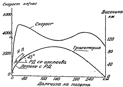
Фиг. 83. Траектория на полета на ракетата V-2
