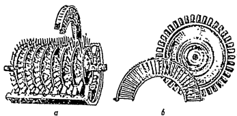
Фиг. 98. Осев компресор
