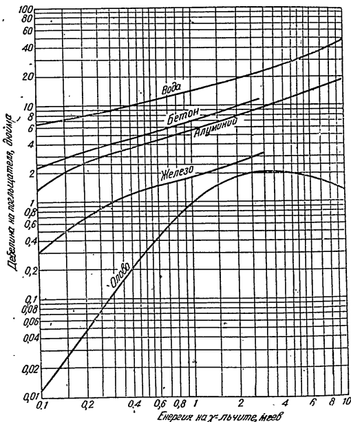
Фиг. 4. Изменение на дебелината на слой с десетократно отслабване за различни вещества в зависимост от енергията на γ-лъчите
