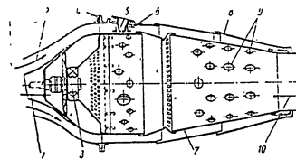
Фиг. 100. Индивидуална горивна камера: 1 — вход на първичния въздух; 2 — вход на вторичния въздух; 3 — форсунка; 4 — фланец; 5 — съединителна тръба; 6 — цилиндричната част на кожуха; 7 — пламъкова тръба; 8 — кожух; 9 — отвори за въздух; 10 — изход на газовете
