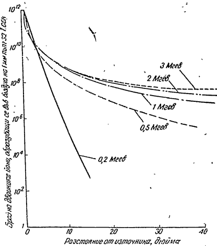
Фиг. 8. Брой на образуваните двойки йони на единица път на \beta -частиците във въздуха за 1 сек. като функция на разстоянието от източник с активност 1 кюри: Взема се под внимание поглъщането на \beta -лъчението във въздуха, намиращ се между източника и обекта
