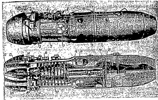
Фиг. 99. Общ вид и разрез на турбо-реактивен двигател с осев компресор:
