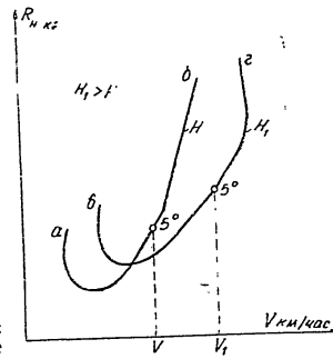
Фиг. 120. Зависимост на R_H от височината H при хоризонтален полет
