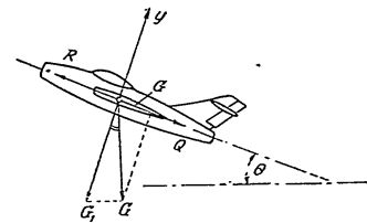
Фиг. 124. Сили, действащи на самолета при изкачване
