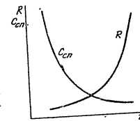
Фиг. 111. Оборотна характеристика на турбо-реактивния двигател
