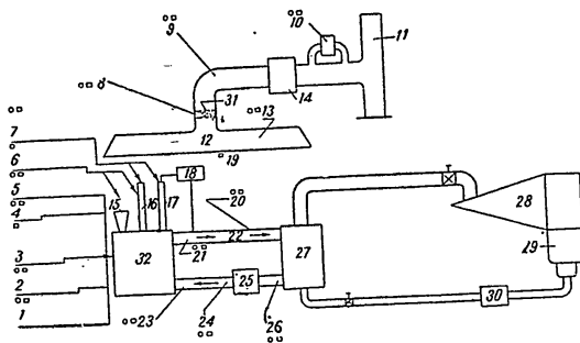
Фиг. 2. Схема за поддръждане на уредите, предназначени за контролиране и аварийно управление на реактор с газово охлаждане.
