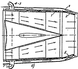
Фиг. 108. Реактивно сопло с неподвижен конус
