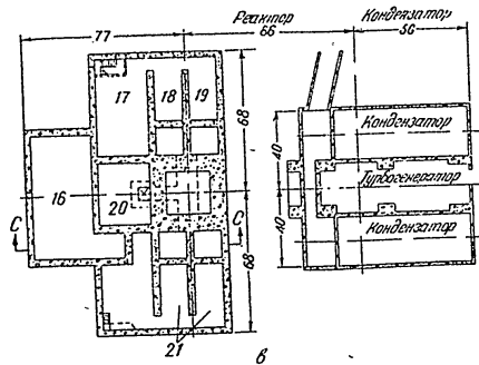
Към фиг. 2. 16 — хранилище за облъчените топлоотдаващи елементи; 17 — помещение за обработване на водата, за пазене на подхранващата вода и за помпите; 18 — въздушни канали и разни съоръжения; 19 — система за климатизиране на въздух и сукателни вентилатори; 20 — съоръжения за охлаждане на забавителя; 21 — хранилище за замърсената вода
