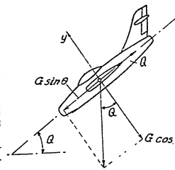
Фиг. 126. Планиране на самолета. Сили, действувачи при планирането
