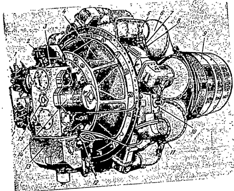
Фиг. 97. Турбо-реактивен двигател с центробежен компресор: 1 — горивни помпи; 2 — барометрически регулатор; 3 — корпус на псеводите за агре- гатите; 4 — защитна мрежа; 5 — филтър за закръване на форсунките; 6 — предпа- зителна мрежа; 7 — горивен тръбопровод за малък газ; 8 — горив- ен тръбопровод за основното гориво; 9 — външен кожух на реактивното сопло; 10 — външен кожух на основното гориво; 11 — прекожна тръба; 12 — газова камера на засло- на; 13 — заслоносборач; 14 — стартер; 15 — отдушник
