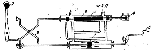
Фиг. 54. Бустерно управление — схема
