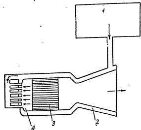
Фиг. 136. Принципа схема за възможен атомни реактивен двигател: 1 — резервоар с работно вещество; 2 — риза за охлаждане; 3 — атомни реактор; 4 — пръскане на работно вещество
