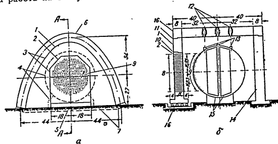
Фиг. 1. Устройство на биологичната и радиационната защита на реактор с газово охлаждане. Сферичният корпус е направен от стомана марка SA204, клас В, дебела 1,67 дюйма, с диаметър 44 фута. Корпусът се монтира след излизане на бетонния свод. Предполага се, че през свода не ще прониква радиоактивно лъчение (всички размери на фигурата са дадени във фута):
