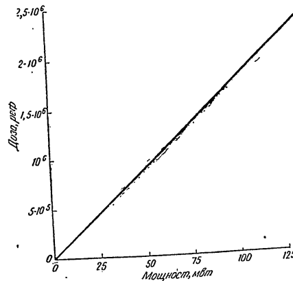
Фиг. 13. Графика за прензчисляване в вт на дозата, изразена в реф за 1 фунт материал, облъчван за 1 работен ден, равен на 20 часа
