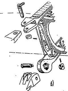
Фиг. 39. Схватки на крилата
