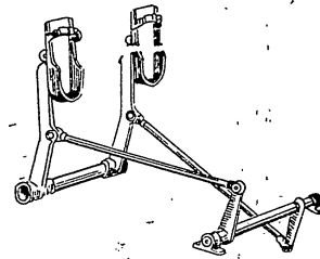
Фиг. 53. Крачно управление
