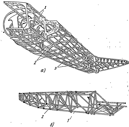
Фиг. 61. Видове тела: а — гредово тяло; б — ферменно тяло; 1 — надлъжници; 2 — стрингери; 3 — рамки
