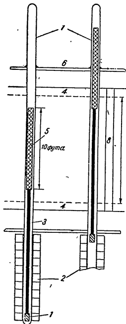
Фиг. 8. Управляващи пръти и соленонден предавател в реактор с течен топлоносител: 1 — магнит; 2 — соленонд; 3 — управляващ прът; 4 — отрязачел; 5 — забавител; 6 — кожух; 7 — изкрайници; 8 — тръби за топлоотделящите елементи; (дължина на топлоотделящите елементи 13 фута).
