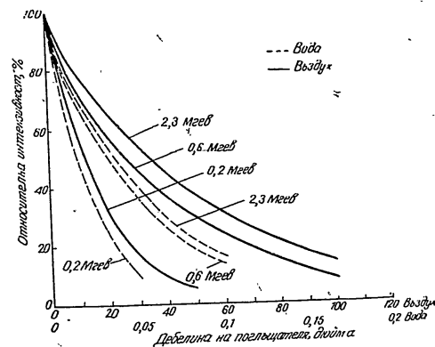
Фиг. 7. Изменение на относителната интензивност на потока от \beta -частици на Sr^{90} (0,6 и 2,3 мгеВ) и Pm^{147} (0,2 мгеВ) в зависимост от дебелината на въздушния и водния слой
