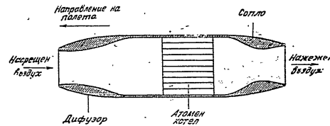
Фиг. 139. Атомен правопоточен въздушно-реактивен двигател (схема)
