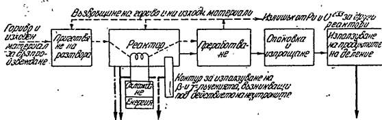
Фиг. 2. Схема на проектирания енергиен реактор с течно гориво, предназначен също за използване като източник на лъчение. Условните знаци са същите както и на фиг. 1
