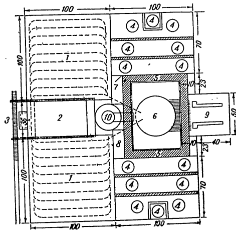
Фиг. 4. План за подреждане на сградите на реактор с газово охлаждане (всички размери на фигурата са дадени във футове): 1 — хранилище за облъчено гориво; 2 — площадка на турбината; 3 — площадка за изтоварване на платформите и на автомобилите; 4 — бойлери и вентилатори; 5 — биологична защита; 6 — реактор; 7 — битови помещения; 8 — помещения на управлението и администрацията; 9 — помещения за пълнене на реактора; 10 — вентилационна тръба
