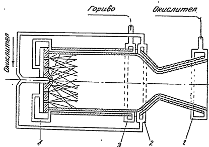
Фиг. 78. Принципа схема на външното охлаждане на горивната камера на течно-ракетен двигател: 1 — входен колектор на окислителя, 2 — изходен колектор на окислителя; 3 — входен колектор на горивото; 4 — изходен колектор на горивото
