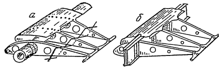
Фиг. 46. Конструкция на крилцата : а — крилце с тръбен надлъжник; б — крилце с двупосен надлъжник
