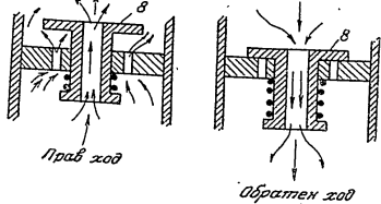
Фиг. 66. Работа на обратния клапан
