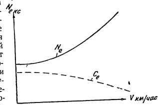
Фиг. 115. Скоростна характеристика на турбовитловия двигател
