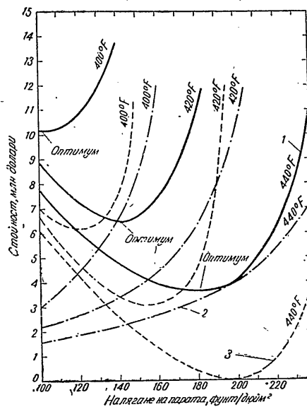
Фиг. 5. График за избрани параметри на парата. Икономически данни, свързани с изменението на температурата и налягането на топлоносителя. Топлинен мощност на реактора 790 мгвт или 2,7·10 6 Б. т. е./час . Данните включват стойността на топлоносителя по външния контур, увеличението на капиталните разходи, стойността на инсталираната мощност, която се изисква за газоуловките, и стойността на инсталираната полезна мощност (375 долара за 1 квт ): 1 — обща стойност; 2 — стойност на топлоносителя във външния контур; 3 — стойност на полезната инсталирана мощност
