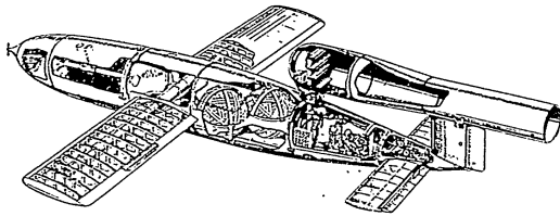
Фиг. 90. Самолет-снаряд „V-1“ с пулсиращ реактивен двигател
