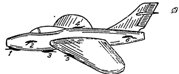
Фиг. 72. Места за възможни разположения по самолета на стрелково-артилерийско въоръжение: 1 — носова установка; 2 — странична; 3 — долна; 4 — горна; 5 — крилна установка; 6 — опашна установка
