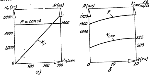
Фиг. 81. Характеристики на течно-ракетен двигател: а — скоростна характеристика; б — височинна характеристика
