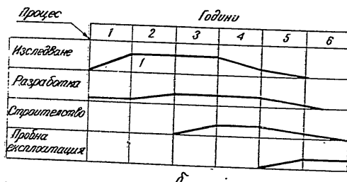
Фиг. 13. Криви, характеризирани времето за изграждане на реактора: а — с газово охлаждане; б — с течно охлаждане
