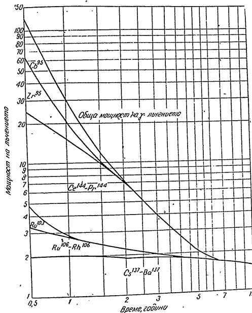
Фиг. 6. Изменение по време на мощността на потока от γ-лъчи, изпускани от продуктите на деление и от най-важните изотопи, влизащи в състава им:
