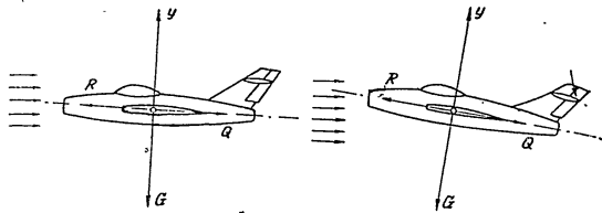
Фиг. 122. Хоризонтален полет
