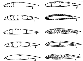
Фиг. 36. Сечение на различни типове крила: 1 — еднонадлъжниково крило с работеща атакуващ ръб; 2 — еднонадлъжниково крило с работеща обшивка; 3 — еднонадлъжниково безстрингерно крило с работеща обшивка; 4 — двуннадлъжниково крило с работеща обшивка; 5 — многоблоково крило с няколко стени; 6 — несечно крило; 7 — крило с многослоева обшивка; 8 — пълно крило; 9 и 10 — дъги или шапковани крила
