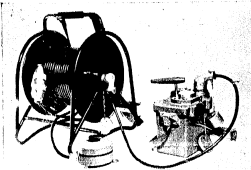
Dělní sestava strojů milisekundový dynamický měřič DMS 25.
