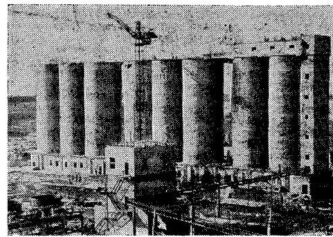
В Липецке на базе богатейших месторождений известняка и глины растет гигант цементной промышленности. Новое предприятие будет одним из самых высококапитализированных в стране. Сейчас на ударной стройке семилетки — горячая предпоследняя пора. Завершается сооружение мощной вращающейся печи, компрессорного цеха, котельной, насосных станций и других важнейших объектов. Полным ходом ведется монтаж теплообменного оборудования сырьевого, цементного и дробильного отделений. Начались малярные работы на цеховой электростанции. С освоением проектной мощности предприятие будет выпускать около миллиона тонн цемента в год. На снимке: строящиеся цементные ежкости. Фото П. Лисенкина. Фотохроника ТАСС.
