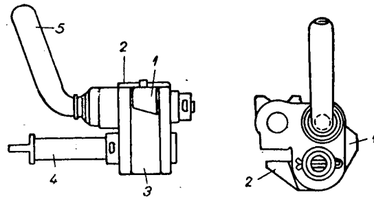
Рис. 28. Страничен механизъм: 1 — затегач; 2 — плъзгач; 3 — съединител; 4 — спиралка; 5 — ръчка
