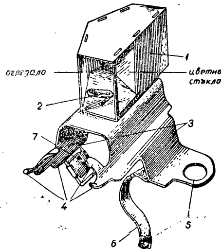
Рис. 4. Универсален ортоскоп: 1 — кутия с цветно стъкло и огледало; 2 — пластинка; 3 — основа; 4 — издатъци за закрепване към пушката и леката картеница; 5 — отворстие за поставяне върху дръжката на ръчника; 6 — лента за закрепване към пушката и леката картеница; 7 — тока за лентата
