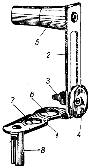
Рис. 2. Универсална диафрагма: 1 — основание; 2 — стойка, 3 — перста ключалка; 4 — подвижен окуляр; 5 — тръбичка за закрепване към пушката; 6, 7 — кръгли отвори за закрепване към картеницата; 8 — шип за закрепване на диафрагмата към старите образци тежки картеници
