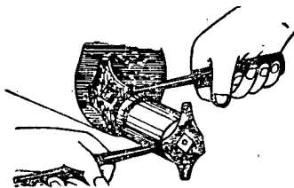
Рис. 10. Отвиване втулката на усилвача на ритането
