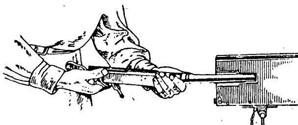
Рис. 9. Изваждане рамката с цевта
