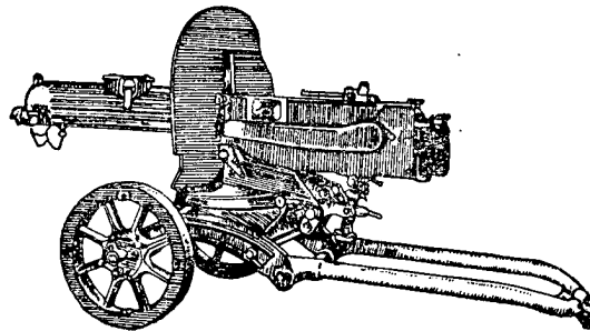
Рис. 5. Общ вид на тежката картечница
