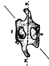
Рис. 5. Силуэтный снимок планетарной туманности NGC 7026. Цифры означают \lg J . Пунктирная линия — магнитная ось туманности, черточки — направление плоскости, параллельной галактическому экватору.
