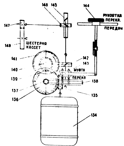
Рис. 28. Кинематическая схема фотопроставки
