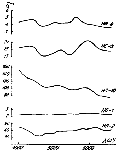
Рис. 2. Пропускания нейтральных фильтров
