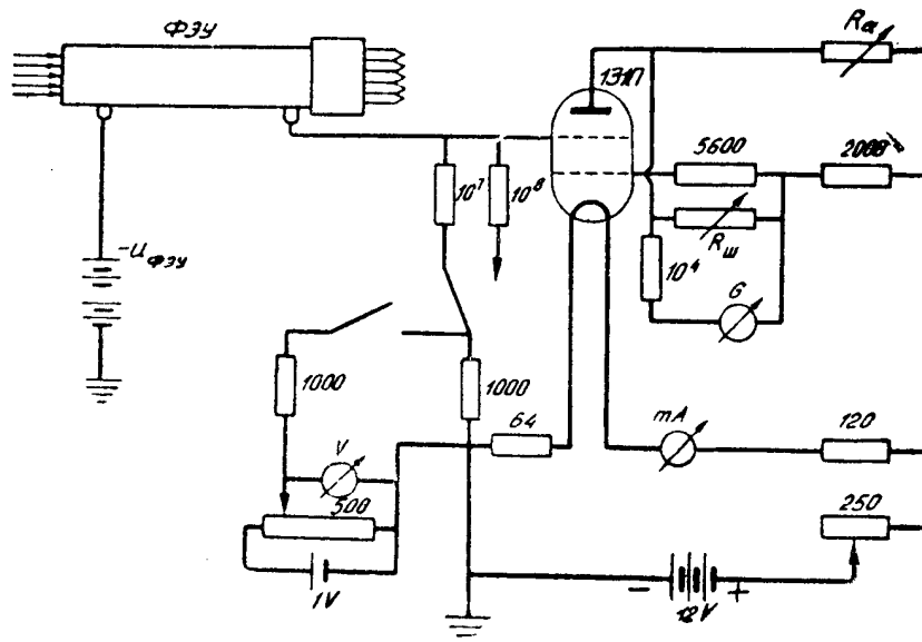
Рис. 8. Схема электрофотометра
