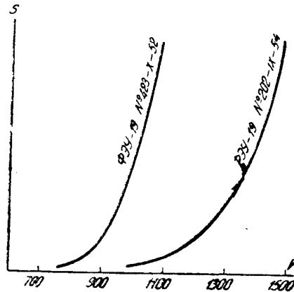
Рис. 3. Вольт-амперные характеристики умножителей
