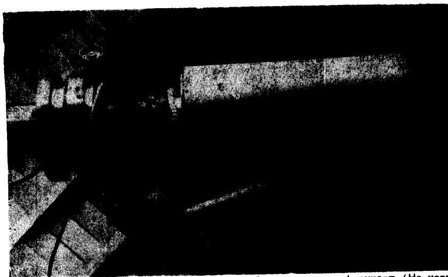
Рис. 5. Корпус с умножителем, прикрепленный к 33-см рефлектору. (На корпус надет металлический цилиндрический футляр, в который насыпался «сухой лед» при пробных охлаждениях умножителя)
