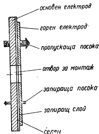
Фиг. 16. Разрез на селенова токоизправителна клетка
