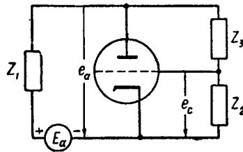
Рис. 1. Автогенератор по обобщенной трехточечной схеме.
