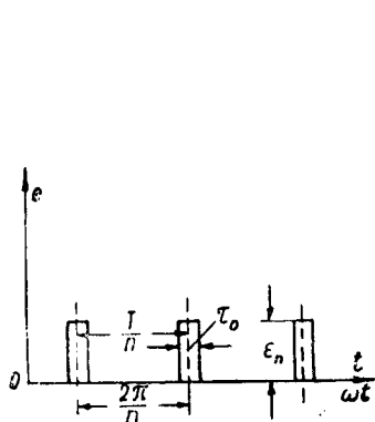
Рис. 4. Временная диаграмма захватывающего напряжения.
