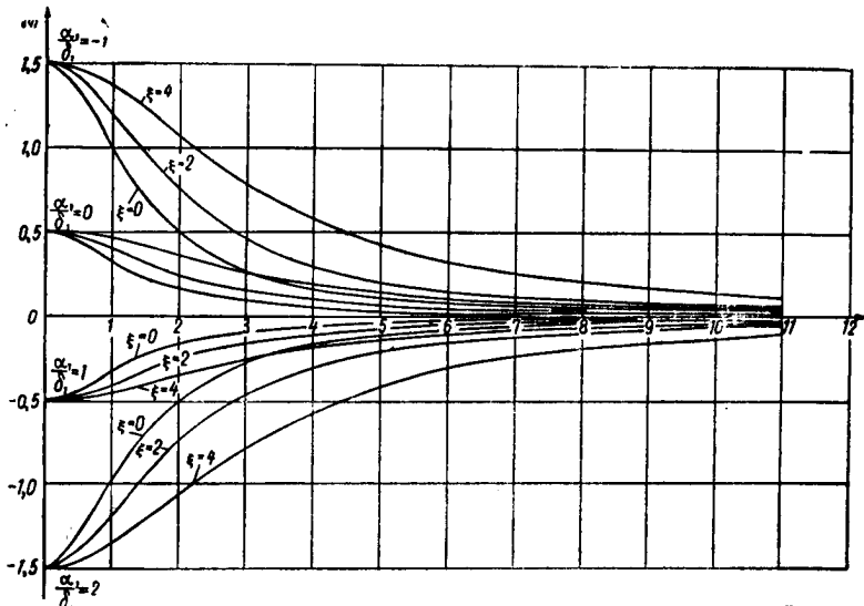
Рис. 7. Зависимость относительной величины временной погрешности \gamma_{ч1} = \frac{\Delta\tau_{лч1}}{\Delta\tau\delta_1} от обобщенного параметра \eta = \frac{\tau\Delta\omega}{\sqrt{2 \ln S_\Delta}} для различных значений \xi = \Delta\Omega\tau и \frac{\alpha_1}{\delta_1} = \frac{\Omega_0}{\Omega} при \beta = 1 .
