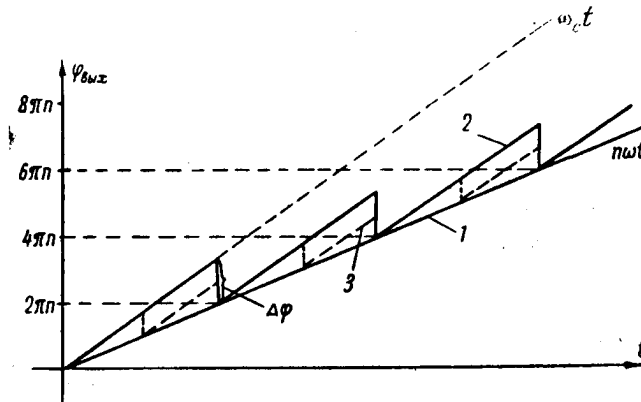
Рис. 4. Изменение фазы на выходе умножителя.
