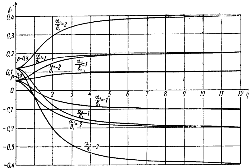
Рис. 5. Зависимость относительной величины временной погрешности \gamma_1 = \frac{\Delta\tau_n}{\Delta\tau\delta_1} от обобщенного параметра \eta = \frac{\tau\Delta\omega}{\sqrt{2 \ln S_\Delta}} для различных значений \beta = \frac{\Delta\omega_2}{\Delta\omega_1} и \frac{\alpha_1}{\delta_1} = \frac{\Omega_0}{\Omega} .
