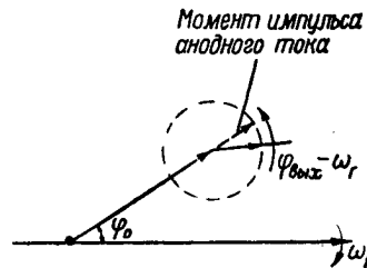
Рис. 12. Векторная диаграмма напряжений на сетке преобразователя.
