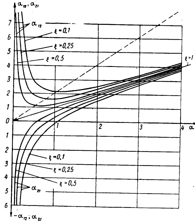
Рис. 1. Зависимость \alpha_{12} и \alpha_{21} от величины \alpha при разных значениях \xi . (Пунктирной линией показано геометрическое место точек минимума \alpha_{12} ).
