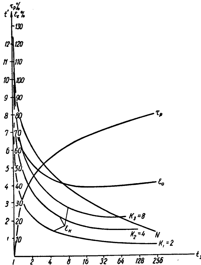
Рис. 6. Зависимость N_i = f(t_s) , \tau_p = f(t_s) , \epsilon_k = f(t_s) и \epsilon_0 = f(t_s) для трубки типа 13ЛЮ37.
