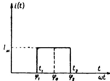
Рис. 4. Временная диаграмма импульса анодного тока.
