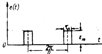
Рис. 7. Временная диаграмма захватывающего напряжения.
