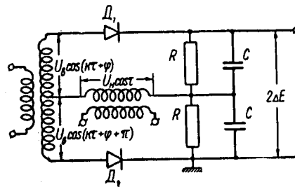
Рис. 1. Схема кратнотазового детектора.
