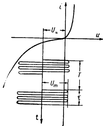
Рис. 9. Диаграмма напряжений пикового детектора в установившемся режиме.
