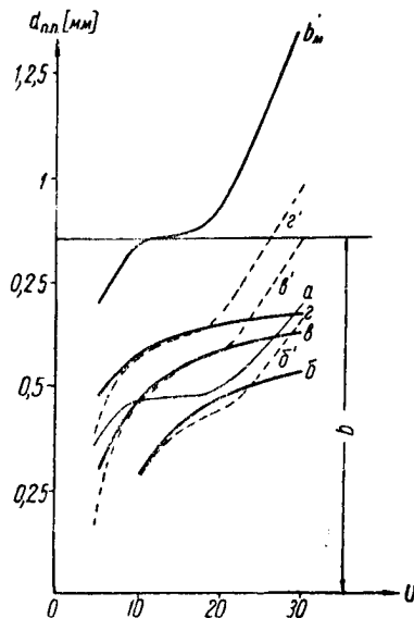
Рис. 3. Зависимость диаметра пишущего пятна от напряжения на модуляторе трубки 13ЛО37 d_{nn} = f(U) : а — диаметр на уровне \frac{1}{e} ; б, в, г — теоретический диаметр пишущего пятна соответственно для B_{2\text{мин}} , B_{2\text{мин}} , B_{1\text{мин}} ; б', в', г' — реальный диаметр пишущего пятна.
