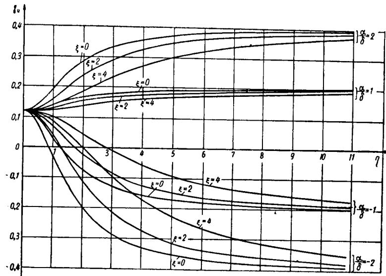
Рис. 6. Зависимость относительной величины временной погрешности \gamma_u = \frac{\Delta\tau_{пч}}{\Delta\tau\delta} от обобщенного параметра \eta = \frac{\tau\Delta\omega}{\sqrt{2 \ln S_\Delta}} для различных значений \xi = \Delta\Omega\tau и \frac{\alpha}{\delta} = \frac{\Omega_0}{\Omega} при \beta = 1 .
