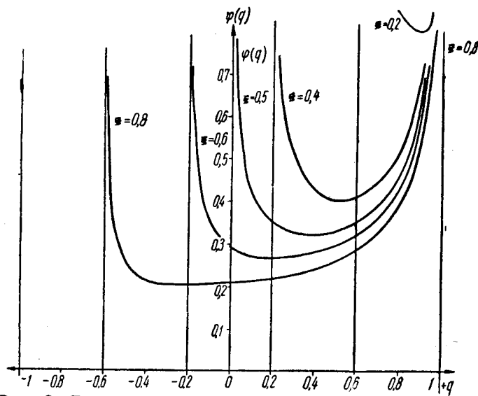
Рис. 3. Плотность вероятностей распределения амплитуд видеоимпульсов на выходе линейного детектора.
