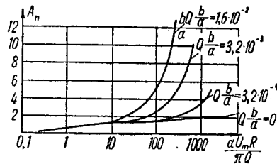
Рис. 12. Функция A_n \left( \frac{a U_m R}{\pi Q} \right) .
