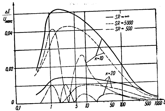
Рис. 13. Зависимость размаха характеристики от b = \frac{U_k}{U_0} и параметра SR .
