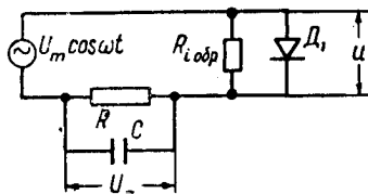
Рис. 10. Эквивалентная схема пикового детектора.
