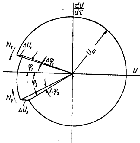
Рис. 12. Фазовая плоскость, изображающая напряжение на контуре.
