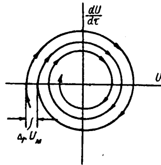
Рис. 2. Изображение затухающих колебаний на фазовой плоскости.
