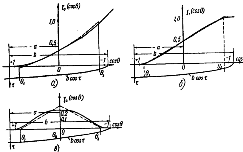
Рис. 3. К определению коэффициентов \gamma_{00} , \gamma_{1K} и \gamma_{22K} .
