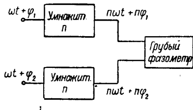
Рис. 1. Блок-схема фазометра.
