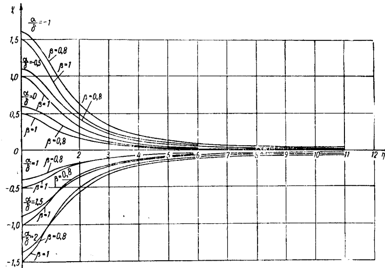
Рис. 4. Зависимость относительной величины временной погрешности \gamma = \frac{\Delta\tau_n}{\Delta\tau\delta} от обобщенного параметра \eta = \frac{\tau\Delta\omega}{\sqrt{2\ln S_\Delta}} для различных значений \beta = \frac{\Delta\omega_2}{\Delta\omega_1} и \frac{\alpha}{\delta} = \frac{\Omega_0}{\Omega} .
