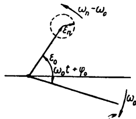
Рис. 1. Векторная диаграмма напряжений сигнала и помехи.
