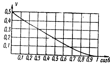
Рис. 7. Функция V(\cos \theta) .
