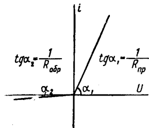
Рис. 5. Идеализированная характеристика вентиля.
