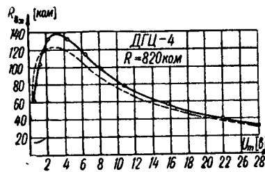
Рис. 8. Экспериментальная (сплошная линия) и расчетная (пунктирная линия) зависимости входного сопротивления детектора R_{вх} от величины амплитуды сигнала U_m .
