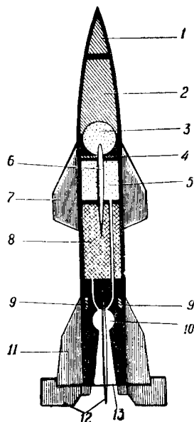
Рис. 12. Снаряд „Васерфаль“:
