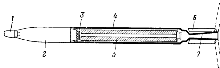
Рис. 17. Снаряд R4M:
