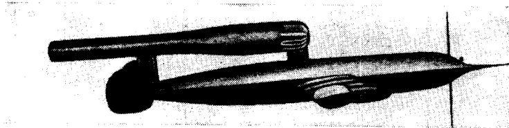
Рис. 65. Французский экспериментальный управляемый реактивный снаряд «Арс-550»
