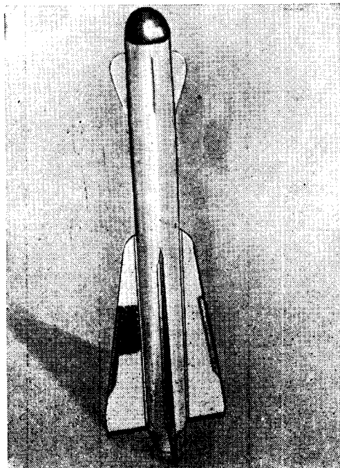
Рис. 55. Авиационный управляемый реактивный снаряд «Фэлкон»
