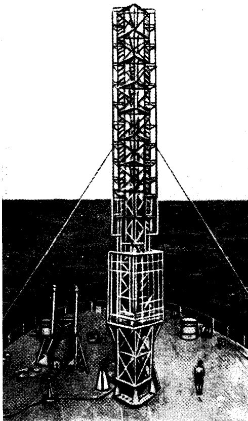
Рис. 60. Снаряд «Аэроб» в пусковой башне на палубе американской плавучей испытательной базы «Нортон Саунд»
