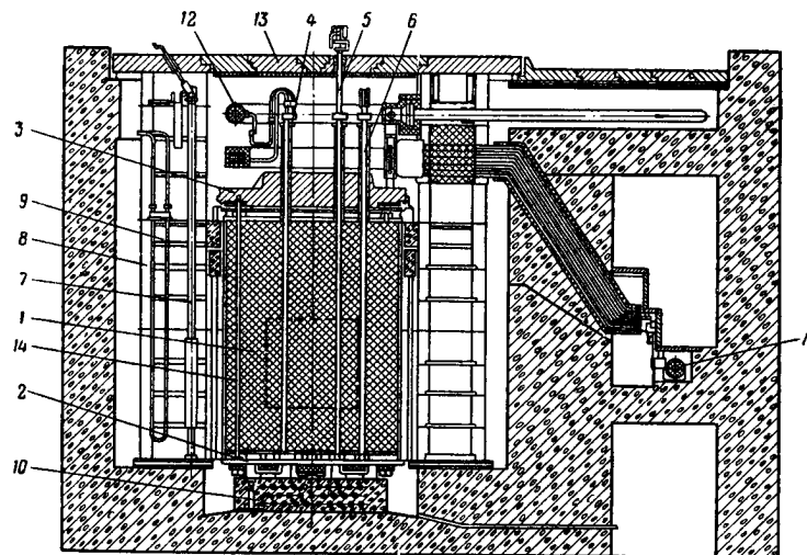
Рис. 51. Реактор атомной электростанции:
