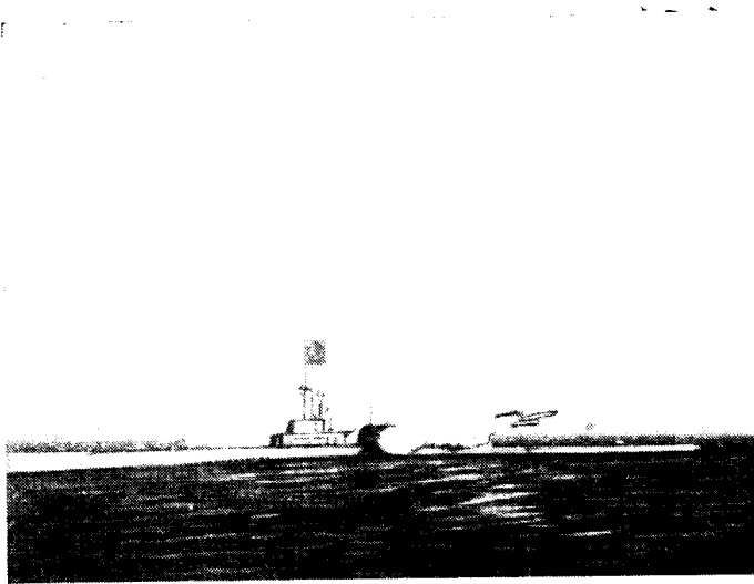
Рис. 20. Запуск снаряда „Лун“ с подводной лодки „Каск“
