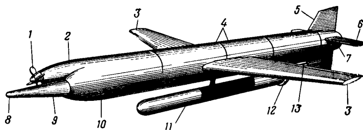
Рис. 13. Снаряд „Шметтерлинг“:
