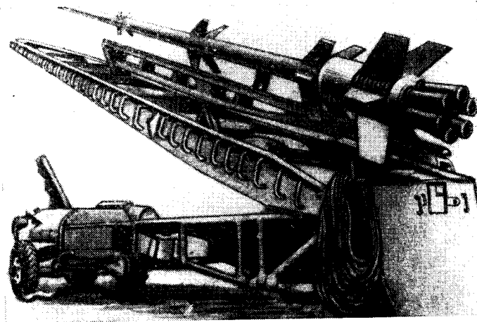
Рис. 11. Многоступенчатый снаряд „Рейботе“ на подвижной стартовой установке
