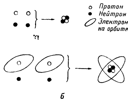
Рис. 29. В обоих случаях а и б убыль массы связана с соединением протонов и нейтронов в ядро. Добавка двух электронов слева и справа в б результата не меняет
