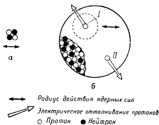
Рис. 38. В ядре а протоны не только отталкиваются электрическими силами, но и притягиваются много большими ядерными силами. В ядре б между протонами I и II действует только электрическое отталкивание
