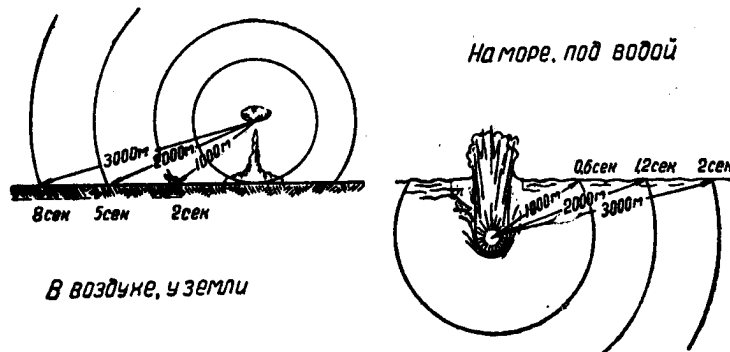
Рис. 23. Скорость распространения ударной волны атомного взрыва в воздухе, у земли и на море, под водой.
