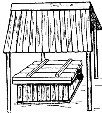
Рис. 24. Шахтный колодец с навесом и герметической крышкой
