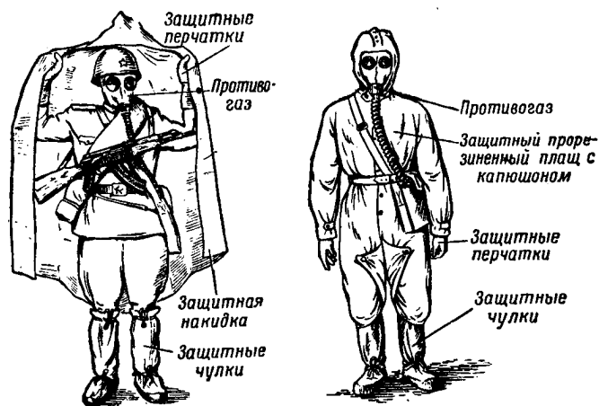
Рис. 25. Индивидуальные средства противохимической защиты солдата (слева) и матроса (справа).
