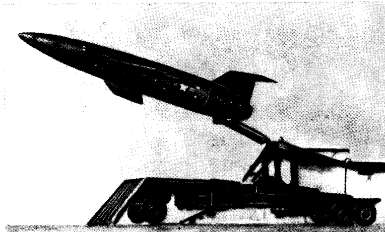
Рис. 23. УРС „Матадор“ в момент запуска с автоприцепа
