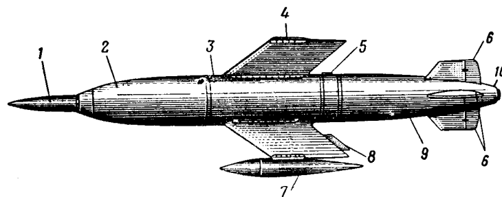
Рис. 18. Снаряд X-4:
