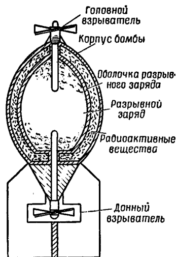
Рис. 42. Принципиальная схема авиабомбы, снаряженной БРВ.
