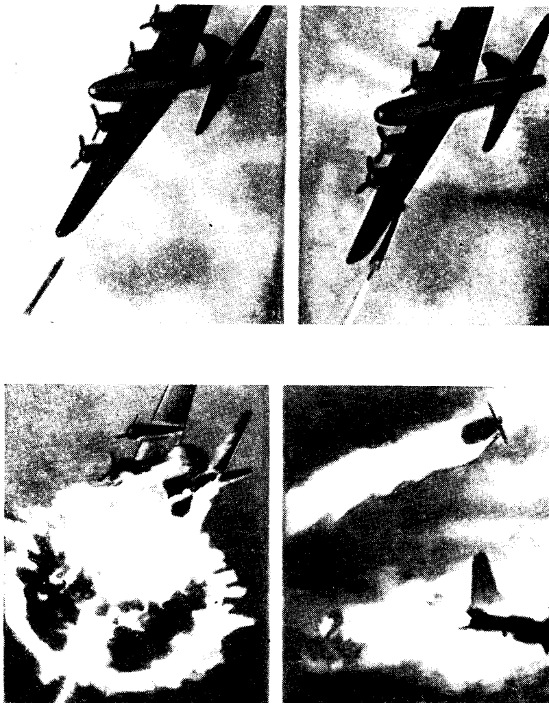
Рис. 44. Поражение воздушной цели зенитным управляемым реактивным снарядом „Найк“; слева направо прибор самонаведения наводит снаряд на цель — бесшляпный бомбардировщик В-17; снаряд приближается к самолету; взрыв снаряда вблизи самолета; гибель самолета
