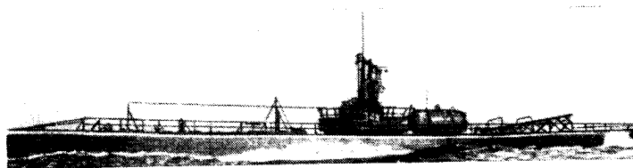
Рис. 21. Подводная лодка с ангаром для хранения УРС и стартовым устройством
