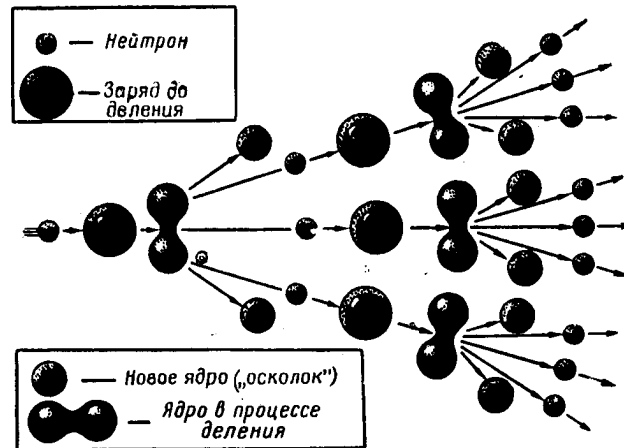
Рис. 11. Схема цепной ядерной реакции в уране. При каждом делении ядра урана образуется 2—3 новых нейтрона, которые вызывают деление последующих ядер.
