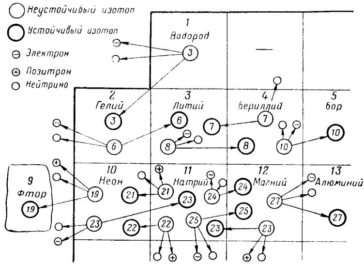
Рис. 33. Левый верхний угол таблицы Менделеева. Показаны искусственные радиоактивные изотопы и их превращение в устойчивые. Изотоп бериллия 7 превращается в литий, не излучая позитрон и нейтрино, а поглощая один из ближайших к ядру электронов (первого слоя) и излучая нейтрино
