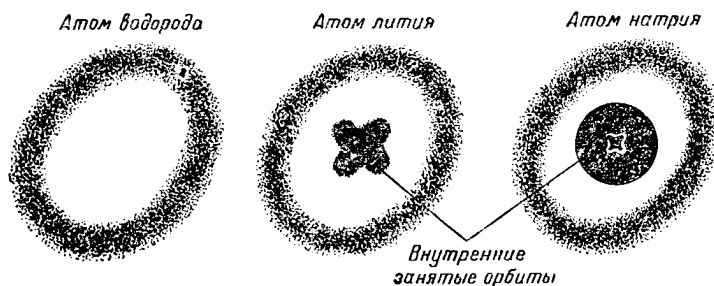
Рис. 18. Схематическое изображение атомов водорода, лития и натрия. Ядра не видны, так как они при этом увеличении слишком малы. У всех этих атомов в наружном слое находится один электрон. Это объясняет их химическое сходство (см. рис. 2)
