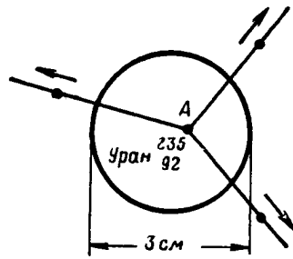
Рис. 44. Нейтроны, возникшие при взрыве ядра (в точке A ), в небольшом кусочке урана ^{235}_{92} разлетаются, не успев попасть в какое-либо другое ядро
