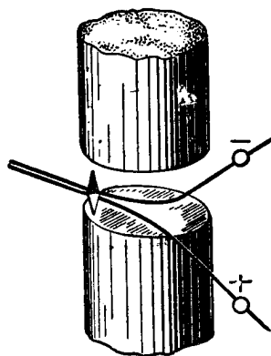
Рис. 7. Действие магнитного поля между полюсами магнитов на движущиеся заряды и магнитную стрелку. Пути заряженных частиц между полюсами магнитов показаны линиями
