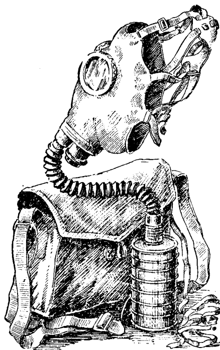
Рис. 15. Общий вид гражданского противогаза ГП-4
