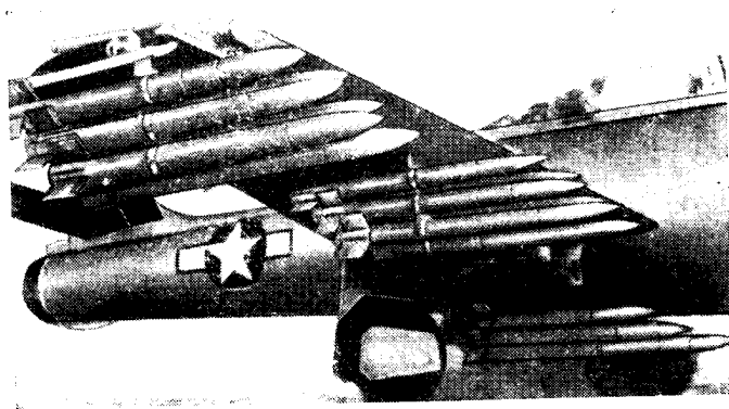
Рис. 30. Подвеска реактивных снарядов «Холи Моусез» под крыльями и фюзеляжем самолета «Тандерджет»
