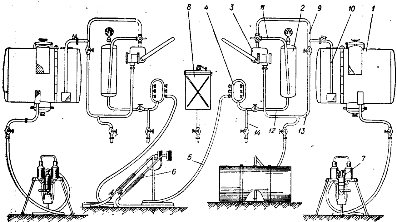
Рис. 11. Схема за устройството на автодегазациялната машина АДМ-48:
