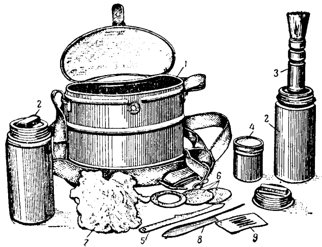
Рис. 3. Картечно-минометен дегазационен комплект: 1 — кутия (калф); 2 — дегазационни туби; 3 — четка; 4 — дървена тубичка; 5 — стъргалка; 6 — уплътнител; 7 — парцали; 8 — дръжка с игла; 9 — запасни иглички
