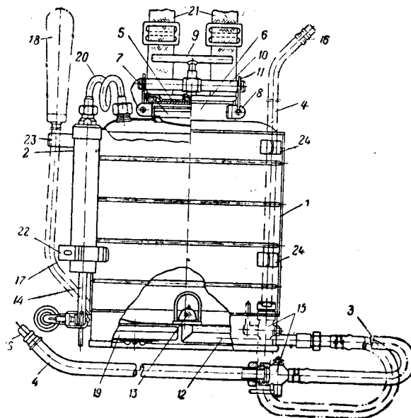
Рис. 6. Ранцев дегазационен прибор РДП-4: 1 — резервоар; 2 — въздушна помпа; 3 — маркуч; 4 — брандспойт; 5 — капак; 6 — отвор; 7 — мрежест филтър; 8 — уши; 9 — опорен винт; 10 — кобилина; 11 — скоба; 12 — изливна тръба; 13 — подвижен филтър; 14 — бутало; 15 — кран на брандспойта; 16 — разпръсквач; 17 — лост в неработно положение; 18 — ръкохватка; 19 — кутийка за запасните части; 20 — въздушна тръба; 21 — презрамни ремъци; 22 — хамуточе за закрепване на въздушната помпа; 23 — ключалка за закрепване на стъблото с ръкохватката; 24 — ключалки за закрепване на брандспойта
