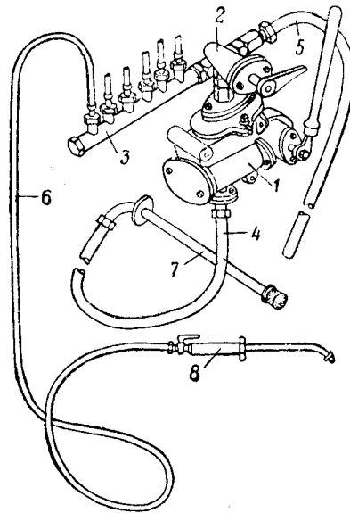
Рис. 14. Хранителна система на автодегазационната машина АДМ-750: 1 — ръчна помпа; 2 — триходов краи; 3 — колектор; 4 — всмукателен маркуч; 5 — нагнетателен маркуч; 6 — раздавателен маркуч; 7 — приемателен сифон; 8 — брандспойт
