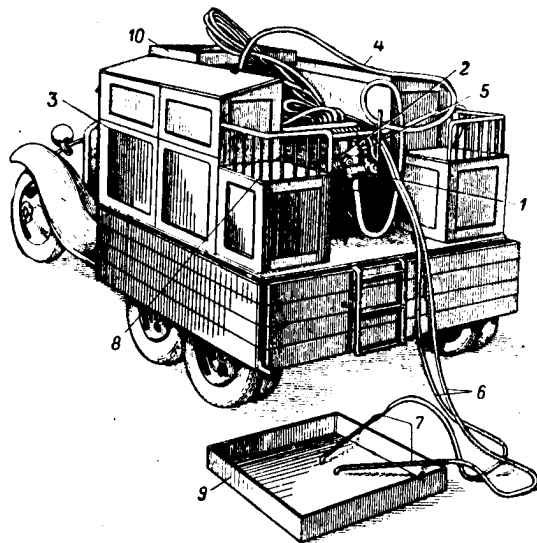
Рис. 13. Автодегазация машина АДМ-750: 1 — ръчна помпа; 2 — варел; 3 — шкаф; 4 — всмукателен маркуч; 5 — нагнетателен маркуч; 6 — разпределителни маркучи; 7 — брандспойти; 8 — седалки; 9 — тава, сне-маема от машината; 10 — тава на машината
