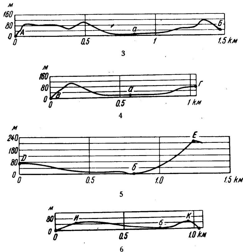
Фиг. 3, 4, 5, 6. Профили кратеров вулкана Малый Семячик
