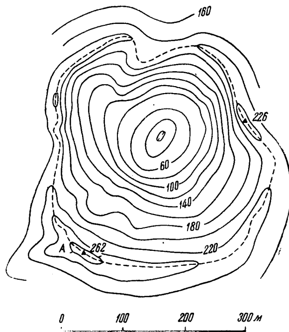
Фиг. 8. План кратера Авачинского вулкана
