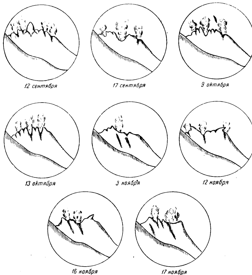
Табл. 1. Изменение формы вершины Суелича в процессе его извержения в 1946 г.
