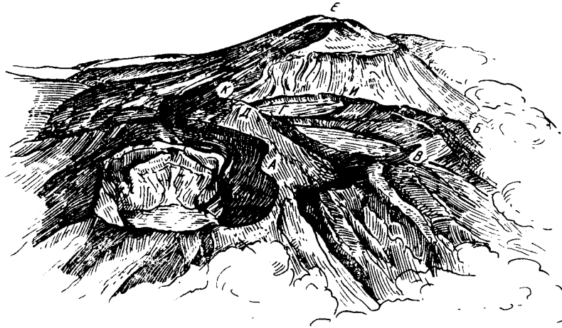
Фиг. 1. Общий вид вулкана Малый Семячик
