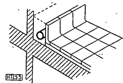
Bild 5: Schemaskizze für die Anordnung der liegenden Sammelabflußleitung oberhalb der Rohdecke hinter der Fliesenscheuerleiste
