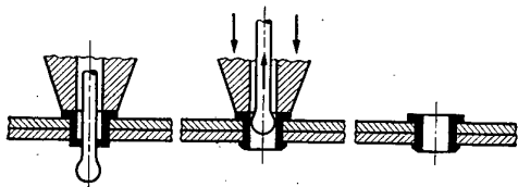
Abb. 26. Durchzieh-Hohlnietung (Chobert-Verfahren).
