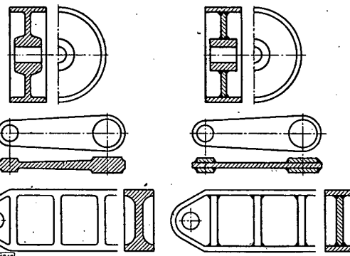
Bild 17 und 18. Gegossene und geschmiedete Leichtmetallteile (links) verglichen mit geschweißten Stahlblechteilen (rechts).
