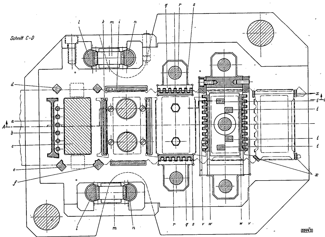
Bild 2. Folgerwerkzeug für Werkstück nach Bild 1 im Senkrecht- und Waagerechtschnitt
