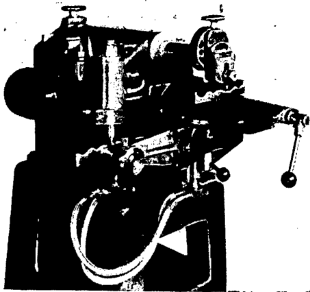
Bild 2. Hydraulischer Kurzhobler mit Kopiereinrichtung (Walter Bartsch, Berlin-Wittenau)
