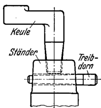
Abb. 41. Nietkeule.
