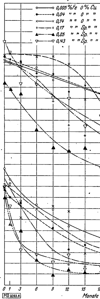
Bild 6. Steigender Fe-Gehalt bei niedrigstem Cu-Gehalt
