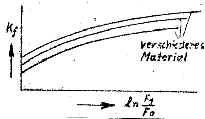
Fließfestigkeit abhängig vom Umformungsgrad
