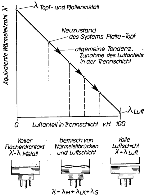
Abb. 13 Schema des Wärmeüberganges in der Trennschicht zwischen Platte und Topf
