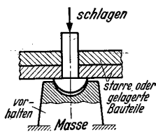
Abb. 37. Direktes Nietten.
