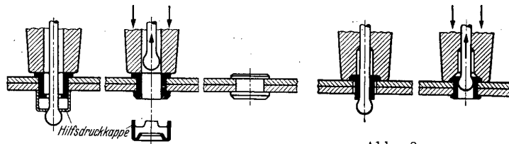
Abb. 28. Schaftstachniet (abgewandeltes Chobert-Verfahren).
