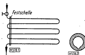
Bild 2 (Mitte): Querschnitt durch ein vom Kondensat angefressenes Rohr
