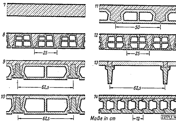
Bild 7. Stahlbewehrte Ziegelsplittbeton-Platte. Bild 8. Stahlsteindecke auf Schalung (DIN 4159). Bild 9. Rippendecke aus Fertigteilen mit Füllkörpern und Aufbeton. Bild 10. Rippendecke aus Fertigteilen mit druckbeanspruchten Füllkörpern. Bild 11. Rippendecke mit Füllkörpern auf Schalung (DIN 4158). Bild 12. Stahlstein-Balkendecke. Bild 13. Rippendecke auf Fertigteilen mit aufgelegten Platten. Bild 14. Vollecke aus dicht verlegten Fertiggliedern.
