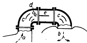
Bild 3. Dampfüberströmrohr zwischen Mitteldruck- u. Niederdruckturbine
