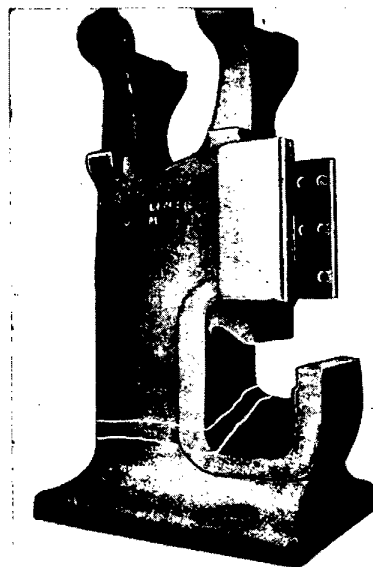
Abb. 16. Exzenterschere-Ständer nach der Warmschweißung.
