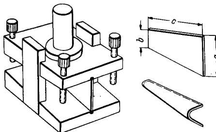
Bild 1. Biegeprüfgerät nach Thompson.
