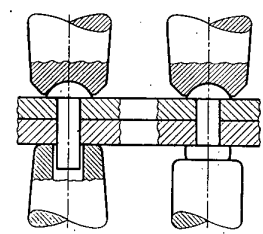
Abb. 9. Anziehen und Schlagen des Flach-Schließkopfes.
