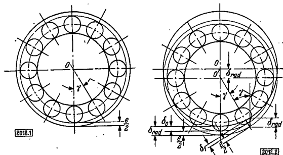
Bild 1. Kugellager mit Spiel. e Lagerluft, \gamma Winkelabstand zweier Kugeln
