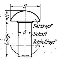
Abb. 7. Bezeichnungen der Nietteile.
