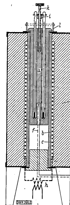
Bild 2. Thermometer-Prüfgerät nach Otte.
