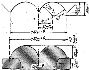
Abb. 5. Kopfform der Nieten für die Arvida-Brücke.
