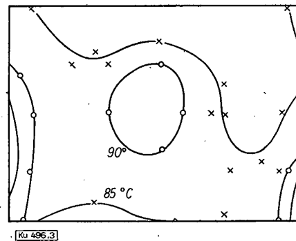
Abb. 3. Siegeldruck 1,36 \text{ kg/cm}^2
