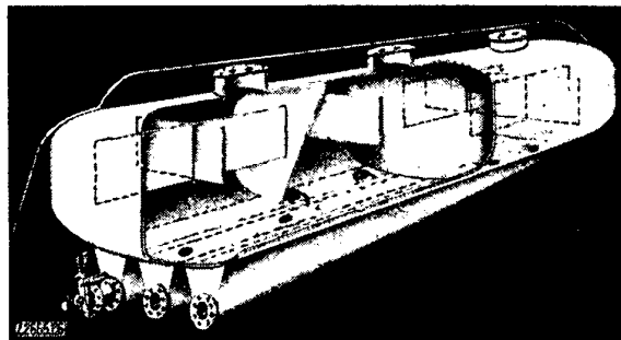
Bild 26. Freitragender Behälter für Tankwagen nach Bild 25. Bauart Haller
