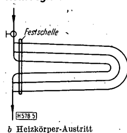
Bild 5: U-förmiges Rohrregister
