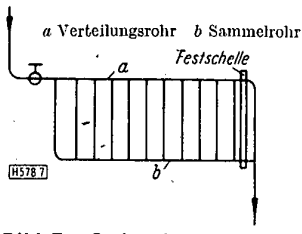
Bild 7: Stehendes ungeteiltes Einzelrohr-Register
