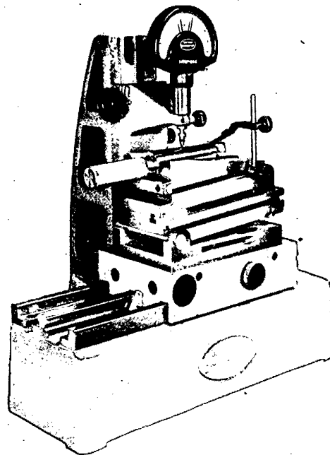
Bild 32. Kegelprüfgerät mit prismatischer Aufnahme (Carl Mahr, Eßlingen|Neckar)
