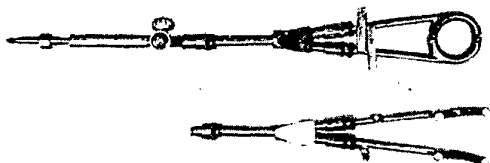
Bild 42. Ringschwenkbrenner (Autogenwerk Sirius GmbH., Düsseldorf)
