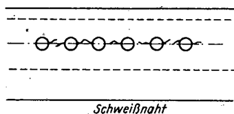
Bild 5. Risse zwischen den Nieten im Flammrohrhals des Kessels nach Bild 4
