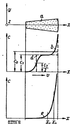
Bild 1. Konzentrationsverhältnisse in einer Zelle der Ultrazentrifuge.
