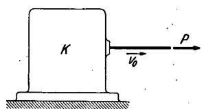
Abb. 22. Kette wird aus einem Behälter herausgezogen.
