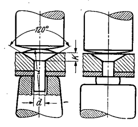
Abb. 12. Flachsenknietung (Flachsen-Setzkopf, Flach-Schließkopf).
