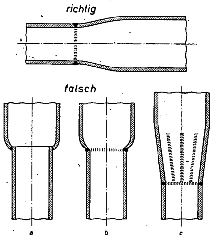
Bild 8. Schweißgerechte Rohrreduktionen
