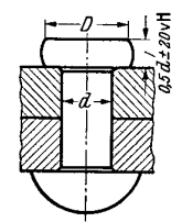
Abb. 8. Flach-Schließkopf.
