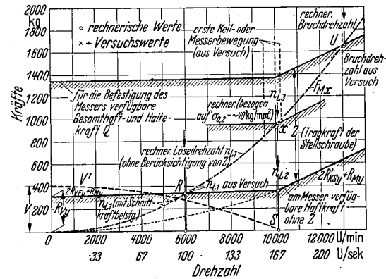
Bild 14. Haft- und Haltekkräfte am Messer einer Schlitzscheibe mit Keilbefestigung in Abhängigkeit von der Drehzahl.
