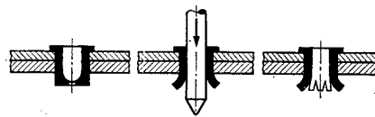
Abb. 29. Klemmniet.
