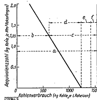
Bild 1. Kohlenverbrauch und -gutschriften bei der Verbundwirtschaft zwischen Hochofen und Kokerei.
