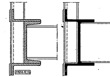
Bild 12. Aus drei Stahlprofilen zusammengesetzter Untergurt. Bild 13. Einteiliger Preßstrang aus Leichtmetall.
