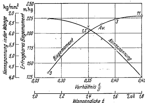
Abb. 2. Einfluß der Kurbelwanddicke auf die Biegedauerfestigkeit.
