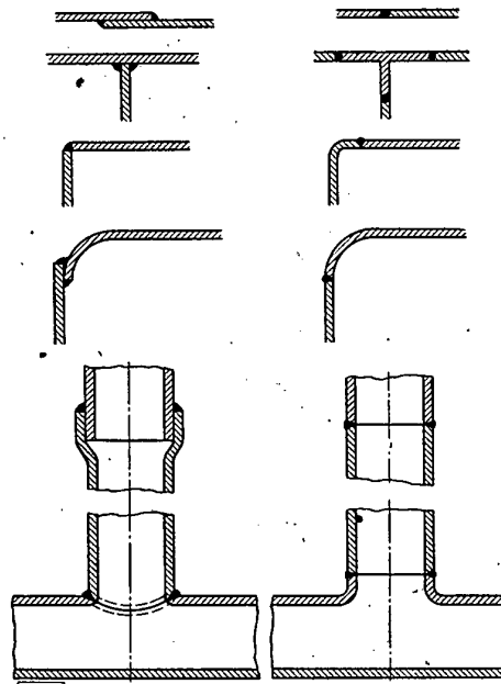
Bild 6. Wegen zusätzlich auftretender Beanspruchungen weniger brauchbare Ausführungen.
