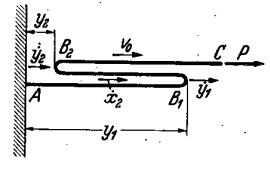
Abb. 23 bis 26. Verschiedene Schemata für die Verhältnisse im Behälter.
