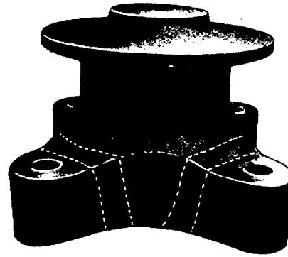
Abb. 9. Hydraulischer Preßzylinder. Zwei Tragpratzen sind durch elektrische Warmmelzschweißung, gleichzeitig verstärkt, wieder angesetzt.
