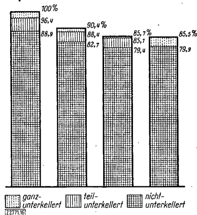
Bild 16. Einfluß der Geschoßzahl auf die Baukosten gleich großer Wohnungen (Wohnungsgröße 50 m 2 ) in beiderseits eingebauten Wohnhäusern mit zwei Wohnungen je Geschoß. von links nach rechts: Haus mit zwei, drei, vier und fünf Wohngeschossen
