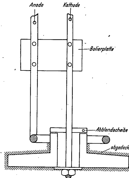
Bild 7. Einhängvorrichtung mit Hilfsanode
