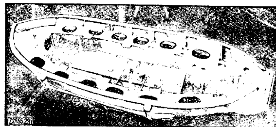
Bild 29. Rettungsboot in Leichtmetall-Schalenkonstruktion. Werkstoff AlMg 3; Argonarc-Schweißung
