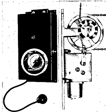
Abb. 3 (rechts): Steuermotor. Abb. 4 (links): Schaltuhr für Tag- und Nachtbetrieb.
