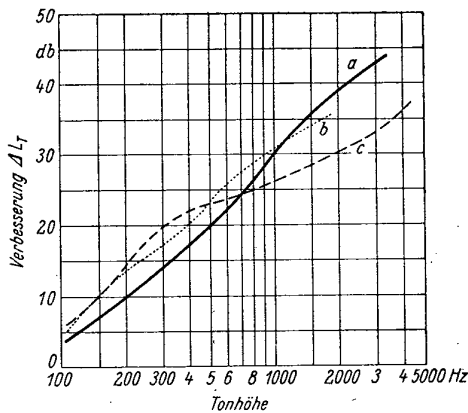
Bild 3. Verbesserung der Trittschalldämmung durch Estriche auf Steinwolleunterlagen.
