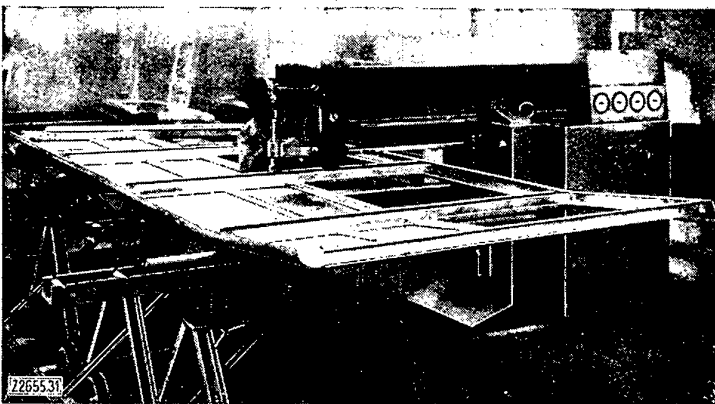
Bild 31. Schweißen von Leichtmetall-Seitenwänden für Eisenbahnwagen auf einer Hochleistungs-Punktschweißmaschine.
