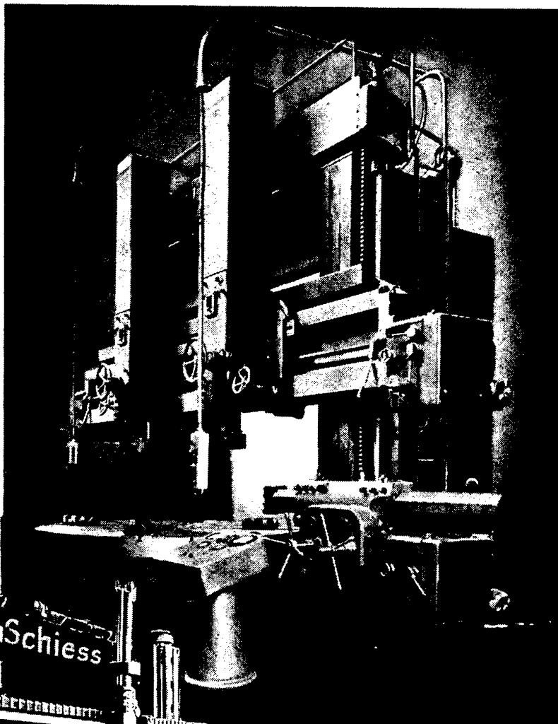
Grosse Karussell-Drehbank m. verschiebbarem Ständer u. Kern-Planscheibe
