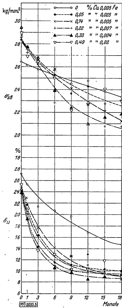
Bild 5. Steigender Cu-Gehalt bei niedrigstem Fe-Gehalt
