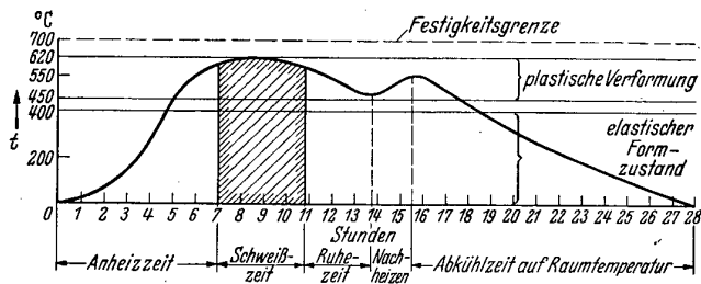
Abb. 4. Temperaturverlauf beim Heizen von gußeisernen Werkstücken bei Warmschweißungen (nach Türcke).
