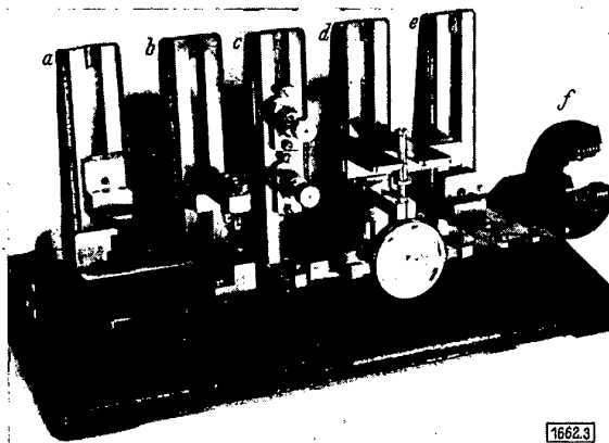
Bild 3. Reihenmeßtisch, eingerichtet für das Messen und Prüfen derjenigen Maße des Werkstückes nach Bild 2, deren Einhaltung erforderlich ist a Außenform und Kleinstmaß der Gesamtlänge mit Formlehre. Größtmaß der Länge mit Höhenmesser, b Außendurchmesser mit Einstelllehre, c Bohrer mit Grenzlehndorn; Gut- und Ausschub-Seite übereinander angeordnet, d Tiefe mit Meßuhr und Auflageplatten, e Sechskant mit Schablone; Gut- und Ausschub-Seite, f Gewinde mit Gewinde-Grenzrachenlehre
