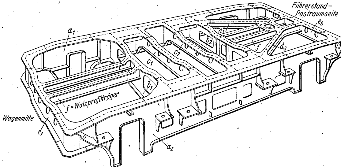
Bild 1. Laufdrehtgestellrahmen für Steuerwagen
