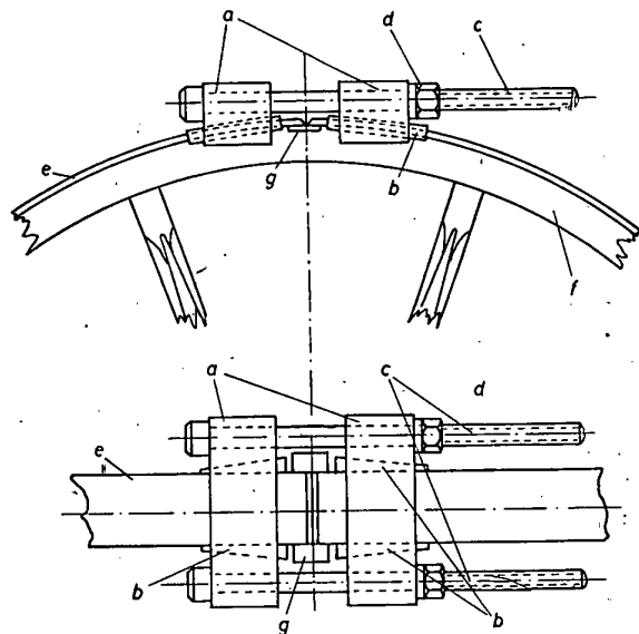
Bild 1. Vorrichtung zum Reifenanziehen auf kaltem Wege a Spannatraverse, b Stahlkeile, c Spannschrauben von 33 mm Durchm. d Spannmutter, e Radreifen, f Holzfelge, g Blechstreifen
