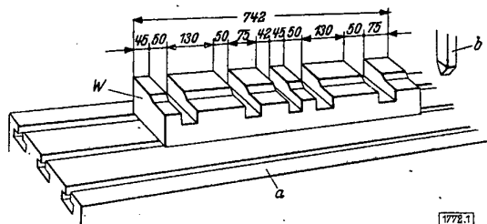
Bild 1. Hobelmaschinentisch mit Versuchs-Werkstück a Maschinentisch, b Hobelstahl, W Werkstück
