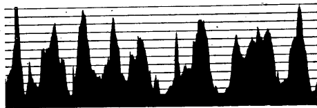
Oberflächenprofilbild einer gedrehten Stahlwelle. Aufgen. mit Leitz-Forster-Gerät. Maßstab: längs 25:1, quer: Teilung \frac{2}{1000} mm, d. h. von Bergspitze zu Bergspitze etwa 0,3 mm, von Tal bis Spitze etwa 0,02 mm
