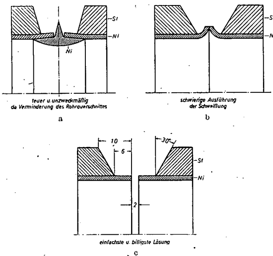
Bild 3. Ausführungsformen einer Stumpfstoßverbindung bei nickelplattierten Röhren
