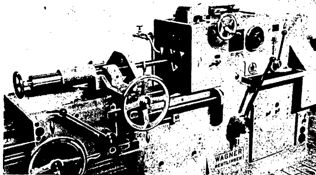
Bild 3. Gewindeschneidmaschine (Gustav Wagner, Reutlingen/Württ.) Arbeitsbereich: Metrische und SI-Gewinde M 8 ... 52, Witworth-Gewinde 3/4 ... 2", Witworth-Rohrgewinde R 1/4 ... 2", Trapez- und Rundgewinde 10 ... 44 mm Dmr. Antriebsleistung rd. 3,5 kW
