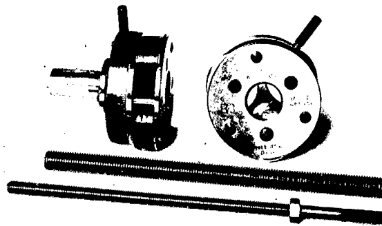
Bild 20. Gewinderollkopf (DP. angem.) (Wilhelm Fette, Hamburg) Darunter: Gewalzte Gewinde
