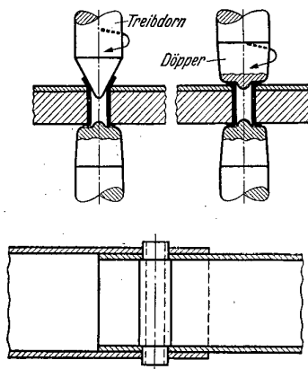
Abb. 21, 22, 23 und 24. Rohrnietungen.
