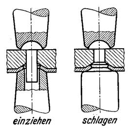
Abb. 11. Einziehnietung.
