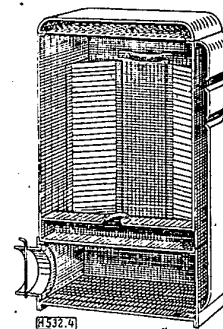
Bild 2 und 3: Sägemehl-Dauerbrandöfen der Göttinger Ofenfabrik Pfeiffer & Sanders
