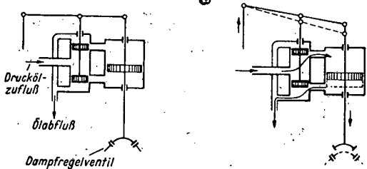
a) Steuerschieber in Mittelstellung, Kraftkolben in beliebiger Stellung in Ruhe.
