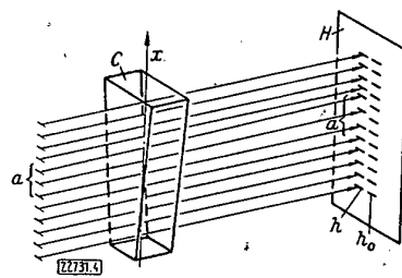
Bild 4. Strahlenverlauf beim Skalenverfahren. Erläuterung s. Text
