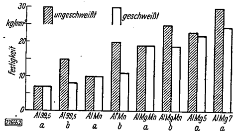
Bild 2. Festigkeitseinbuße durch Schweißen bei nicht aushärtbaren Werkstoffen.
