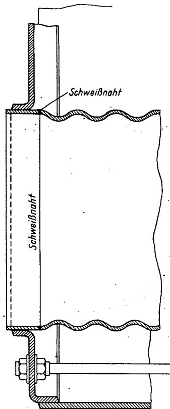
Bild 4. Flammrohr eines Schiffskessels von 245 m 2 Heizfläche
