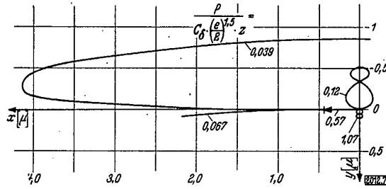
Bild 7. Kugellager mit Spiel.
