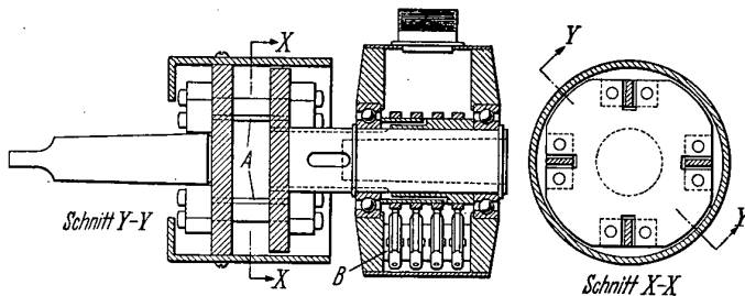
Bild 1. Schnitt durch den Drehmomentenmesser.
