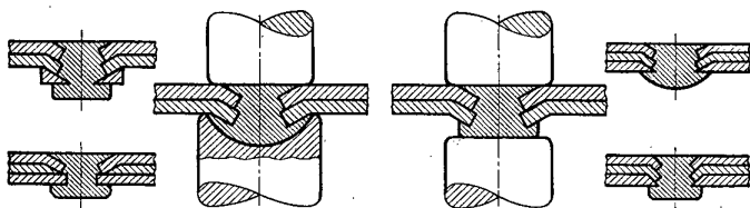
Abb. 17. Glatthautnietungen.
