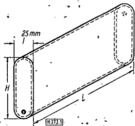
Bild 1: Hagan-Wandplatte
