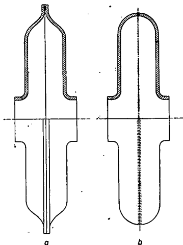
Bild 12. Geschweißte Glieder für Stahlblechradiatoren a widerstandgeschweißt, b autogen geschweißt
