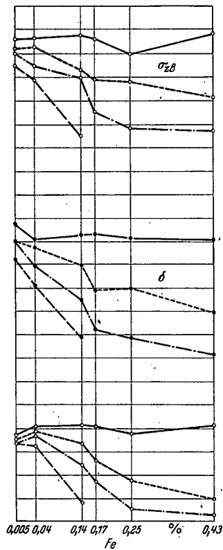
Bild 2. Steigender Eisengehalt bei niedrigstem Kupfergehalt
