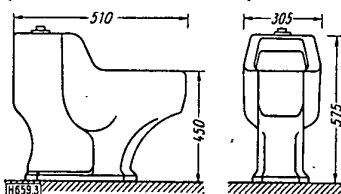
Bild 3: Urinalbecken für Frauen, auch als Klosett benutzbar, zur Benutzung ohne Berührung mit dem Becken (amerikanisches Modell)
