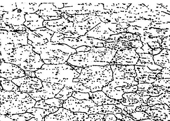
Bild 18. 0,49% Fe; Sp. Cu
