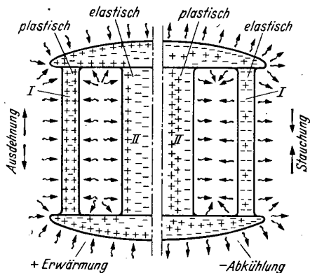
Abb. 5. Schematische Darstellung des Einflusses der Temperaturunterschiede bei gußeisernen Werkstücken mit schwachen außenliegenden und starken innenliegenden Wänden.
