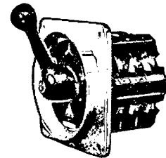
„FANAL“-Nockenschalter (Sterndreieckschalter in Einbauform)
