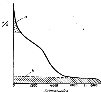
Abb. 1: Geordnete Jahresbelastungslinie eines Heizkraftwerks
