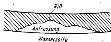
Bild 7. Anfrassungen im Wendekammerboden eines Fährdampferkessels von 50 m² Heizfläche
