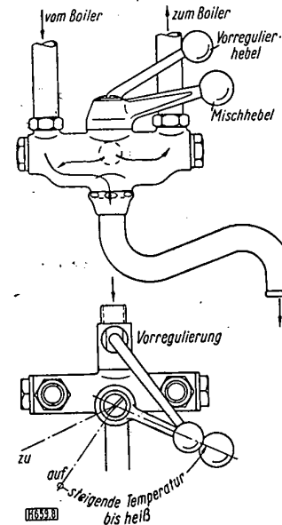
Bild 8: Mischbatterie für Elektrospeicher, Modell Grohe, Hemer, mit Einhebel-Betätigung. Der Betätigungshebel steuert sowohl den Kaltwasser- wie den Warmwasserzulauf.
