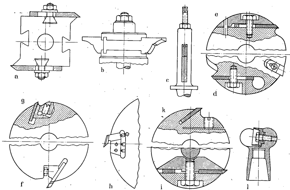
Bild 2a—l. Messerbefestigungen zusammengesetzter Holzfräswerkzeuge.
