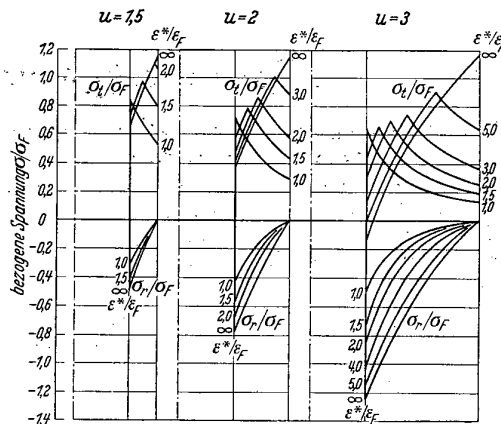
Abb. 4. Spannungsverteilung beim Übergang vom elastischen zum vollplastischen Zustand.
