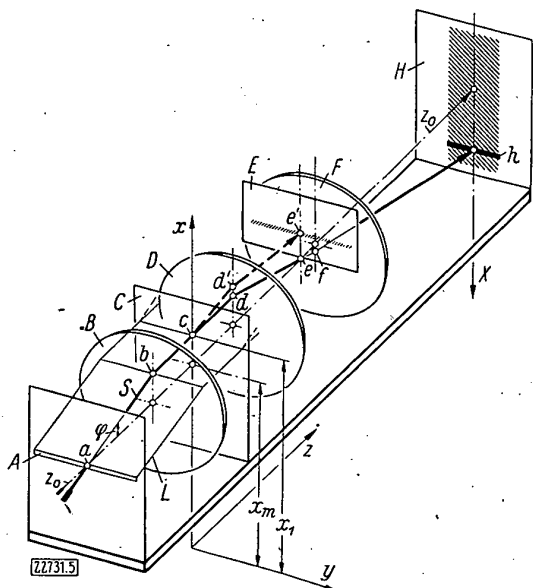
Bild 5. Schema der Töpler-Optik. Erläuterung s. Text
