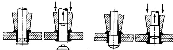
Abb. 30. Hohlriet mit verlorenem Dorn.
