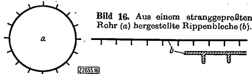
Bild 15 und 16. Punktgeschweißte und stranggepreßte Rippenbleche aus Aluminium.
