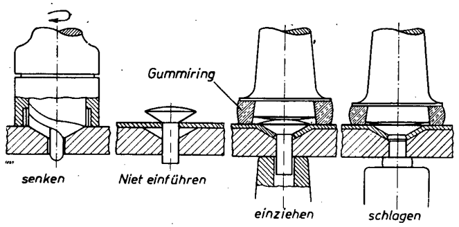
Abb. 13. Flachsenknietung.
