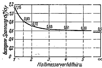
Abb. 2. Einfluß des Halbmesserverhältnisses auf die Zugbeanspruchung bei Fließbeginn.
