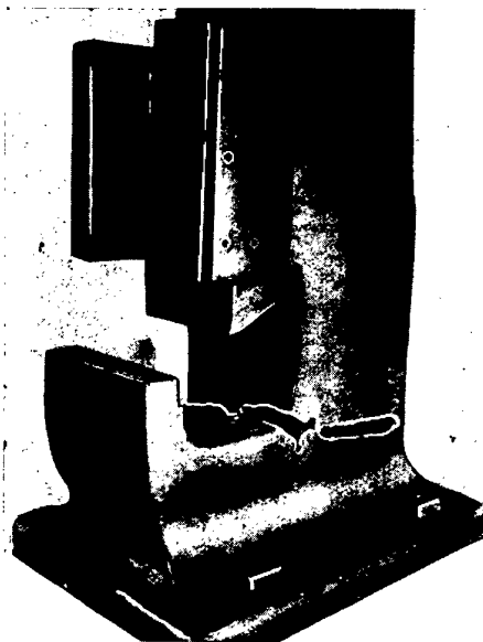
Abb. 12. Exzenterschere-Ständer, 6000 kg Gewicht, mit Rahmenbruch zwischen Fuß und Oberteil, der für die Warmmelzschweißung bereits vorbereitet ist.
