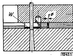
Bild 1. Auswerfer für dünnwandige Werkstücke a Grundplatte, b Einlage, c Führungsplatte, W Werkstück
