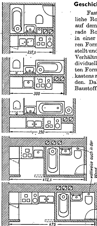
Bild 1: Grundrissarten mit verschiedenen Raumtiefen gemäß DIN 1801 (Normvorschlag nach Mengerlinghausen) (Fenster nach DIN 18050 und Lüftung der Innenbäder nach DIN 18070 nicht dargestellt)
