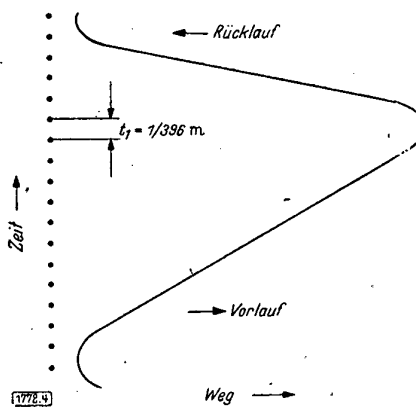
Bild 4. Aufnahme der Tischgeschwindigkeiten im Leerlauf Maschineneinstellung: Vorlauf: v_a = 20 m/min Rücklauf: v_r = 60 m/min Auswertungsergebnisse: Vorlauf: v_a = 24,95 m/min Rücklauf: v_r = 76,6 m/min Umsteuerzeit: t_u = 0,562 s
