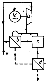
Bild 4. Vereinfachtes Schema der Destillaterzeugung mittels Wärmepumpe.
