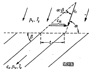
Bild 1. Strömung durch ein ebenes Gitter aus geraden dünnen Schaufeln bei stoßhaftem Eintritt.
