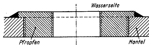
Bild 3. Im Kesselmantel eingeschraubte und verschweißte Gewindescheiben
