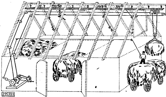
Bild 1. Greiferaufzug für Heu, Getreide und Stroh.
