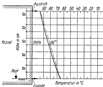
Bild 6. Temperaturverlauf im Kessel.
