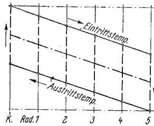
Bild 2. Verlauf der Ein- und Austrittstemperaturen an den Heizkörpern einer Stockwerks-Warmwasserheizung nach der Rietschelschen Berechnung.
