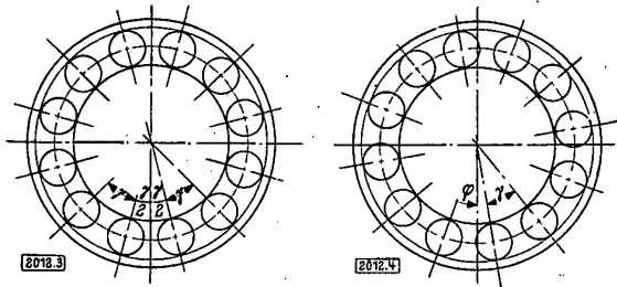
Bild 3. Kugellager mit Spiel. Kugelsatz um \gamma_2 gedreht
