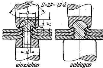
Abb. 16. Pilznietung.
