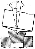
Abb. 2. Schlagen eines Nietkopfes mit Zentrierbohrung mittels Preßlufthammer.
