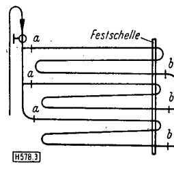
Bild 3: Horizontal unterteilte Rohrschlange
