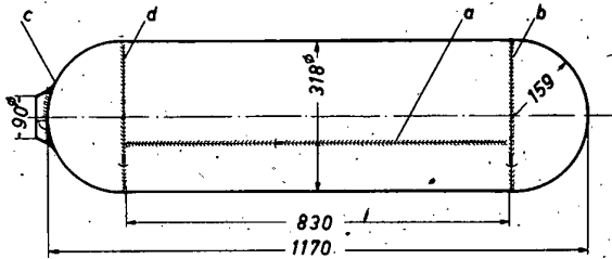
Bild 15. Zweiflammenschweißung von Treibgasflaschen (79 l Inhalt, Werkstoff Kesselblech M II). Schweißnahtanordnung
