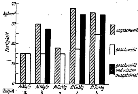
Bild 3. Festigkeitseinbuße durch Schweißen bei aushärtbaren Aluminium-Legierungen.
