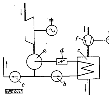
Bild 1. Kondensationsanlage nach Heller.
