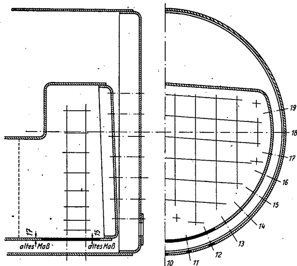
Bild 6. Einschweißen eines verstärkten Wendekammerbodens in einen Fährdampferkessel von 50 m² Heizfläche
