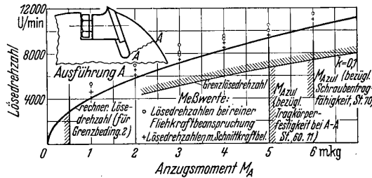
Bild 12. Lösedrehzahlen (bezogen auf Grenzbedingung 2, F_{Mx} < R_{02} ) in Abhängigkeit vom Schraubenanzugsmoment bei einem Universalmesserkopf mit Keilbefestigung.
