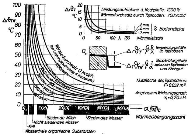
Abb. 14 Temperaturabfall im Topfboden \Delta \vartheta_T und vom Topfboden zum Kochgut \Delta \vartheta_{TW} auf einer Kochplatte 180 \Phi
