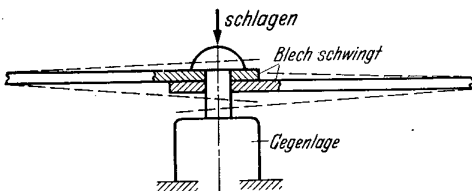
Abb. 38. Indirektes Nietten.
