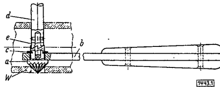
Bild 1. Innensenker
