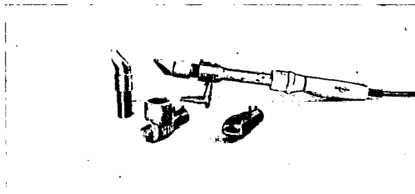
ROTRING-LötKolben „Optimus 2“ mit Universalspitze, schräger Ersatzspitze, Lötbadeinsatz und Brenneinsatz sowie mit schwenkbarem Stützfuß. (Verbrauch 120 Watt)
