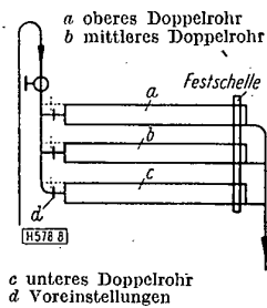
Bild 8 (rechts): Geteiltes Einzelrohr-Register
