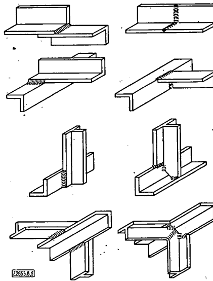
Bild 8. Weniger geeignete Verbindungen.
