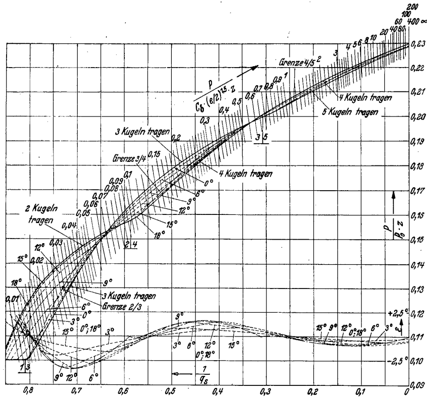
Bild 5. Kugellager mit Spiel Kugelnzahl z = 10 , \frac{P}{P_o \cdot z} = C_\delta \left(\frac{e}{2}\right)^{1,5} z und \epsilon als Funktionen von \frac{1}{q_s}
