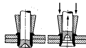
Abb. 32. Hohlrietung nach Loire und Oliver.
