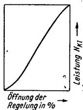
Bild 2. Ideale Leistungskurve einer Kraftwerksturbinen
