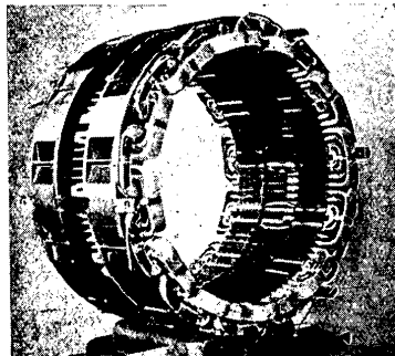
Abb. 4: Ständer eines Motors mit gemeinsamer Feld-Wendepol- und Kompensationswicklung
