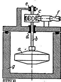
Bild 8. Schema der von Pickels und Beams entwickelten Bauart.
