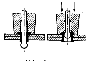
Abb. 28. Schaftstachniet (abgewandeltes Chobert-Verfahren).
