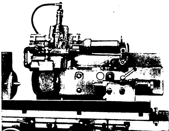
Bild 7. Rundschleifmaschine mit Meß- und Steuereinrichtung zum Einstechschleifen eingerichtet (Hartex GmbH., Berlin-Mariensfelde)
