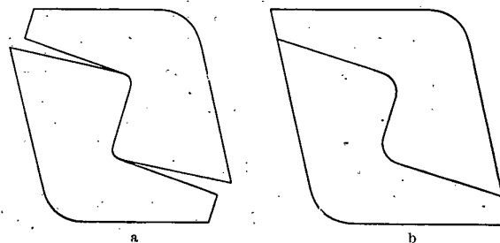
Bild 18. Zweckmäßige Gestaltung von brenngeschnittenen Blechteilen a unzuweckmäßig, b richtig.
