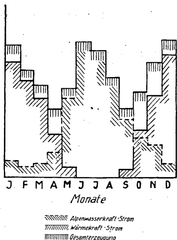
Abb. 3: Ergänzung der Alpenwasserkräfte durch thermische Kraftwerke
