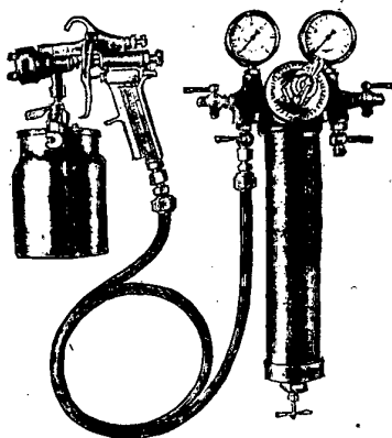
Bild 1. Farbspritzpistole mit Saugfarbgefäß und Luftdruckregler Werkfoto: Defag-DeVilbiss
