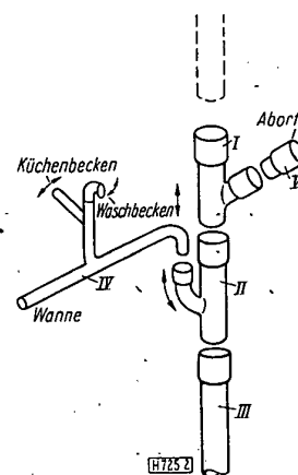
Bild 2: Schema für den Aufbau einer Abflußanlage aus typisierten Fertigbauteilen. Fallrohr Elemente für sämtliche Grundrissarten anwendbar
