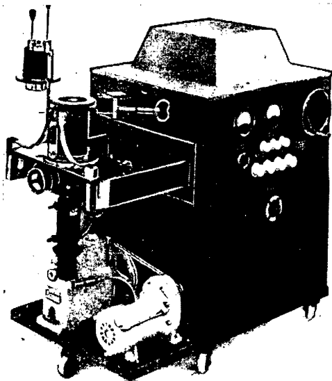
Hochtemperaturofen nach Nernst-Tammann (nutzbarer Tiegelinhalt 30 cm, erreichbare Temperatur bis 2500° C, erreichbares Vakuum bis 1 \times 10^{-4} Torr, Anschlußwert 7,5 kW, 220 V, Ofenhöhe 40 cm, Ofendurchmesser 22 cm)
