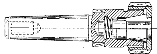
Bild 28. Bohr- und Fräsfutter mit Morsekegel (Eugen Fahrion, Esslingen-Mettingen)
