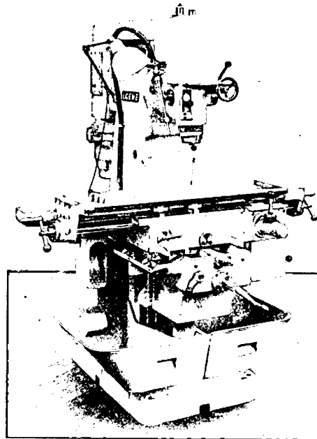
Bild 11. Vertikalfräsmaschine (Ludw. Loewe & Co., Aktiengesellschaft, Berlin)
