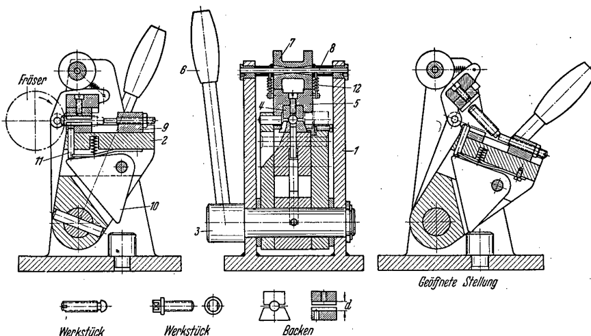
Bild 1. Vorrichtung zum Fräsen von Schlitz- und Schlüsselflächen an Schrauben.
