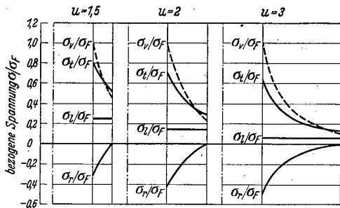
Abb. 1. Spannungverteilung bei Beginn des Fließens.
