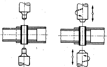
Abb. 21, 22, 23 und 24. Rohrnietungen.
