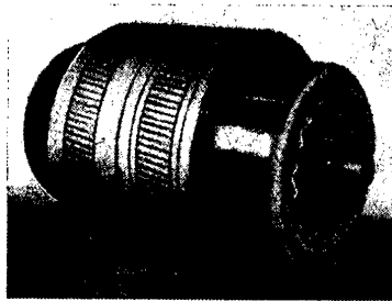
Abb. 3: Welle mit 2 Ankern und 2 Kommutatoren
