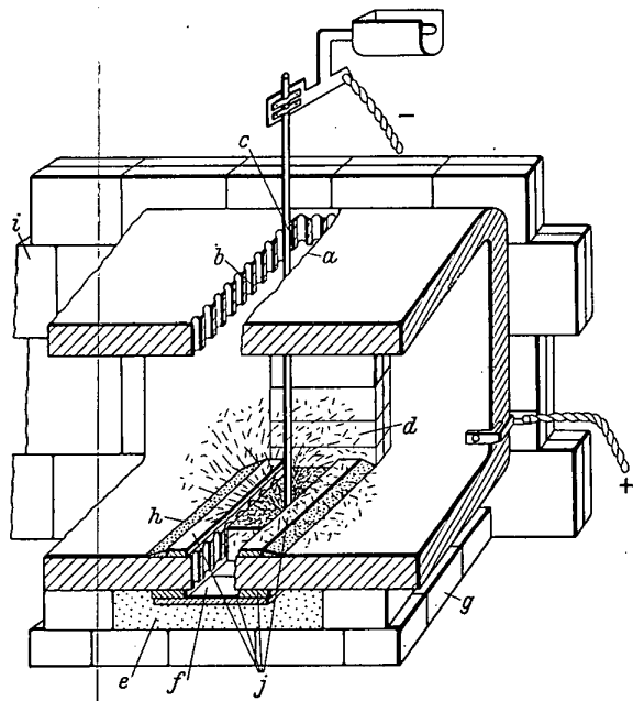
Abb. 14. Schematische Darstellung des ersten Schweißvorganges an dem umgelegten Scherenständer nach Abb. 12. a Bruchverlauf; b Kettenbohrung; c Gußelektrode; d Kohleformwand für senkrechte Bruchwand; e Formsand; f untere Schweißform; g Mauerwerk; h Klebsand; i Ofenwand; j Kohleplatten.
