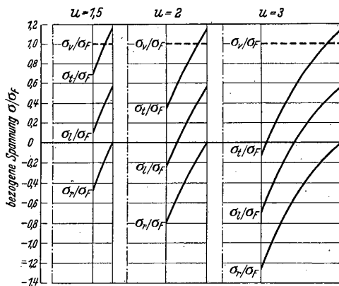
Abb. 3. Spannungsverteilung im vollplastischen Zustand.
