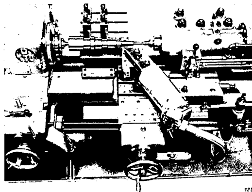
Bild 1. Halbautomatische Vielstahl- und Kopierdrehbank (Gebr. Heinemann AG., St. Georgen i. Schwarzw.)
