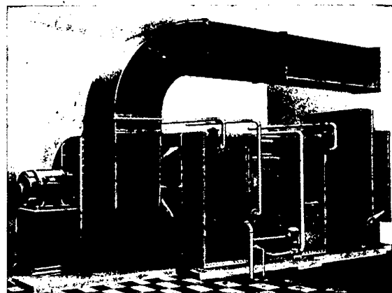
Klimaapparat mit Umlauffilter für Großsenderanlage
