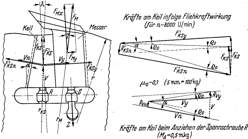
Bild 13. Kräfte in der Keilbefestigung einer Schlitzscheibe.
