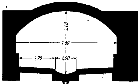
Bild 1. Nesenbach-Profil
