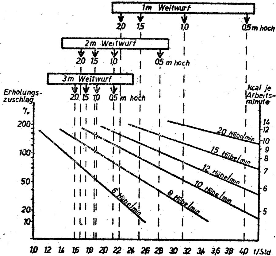
Schaufelleistung und Erholungszuschlag mit 8 kg Schaufellast und 250 Arbeitskatorien je Stunde in Abhängigkeit von Hubzahl, Wurfweite und Wurthöhe.
