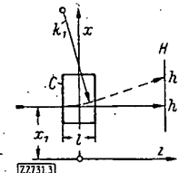
Bild 3. Krümmung eines Lichtstrahls in der Präparatzelle beim Refraktionsverfahren. Erläuterung s. Text
