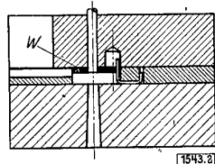
Bild 2. Auswerfer-Stellung kurz vor dem Auswerfen des Werkstückes W Werkstück
