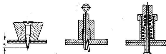
Abb. 46. Holzschrauben-Hefter.
