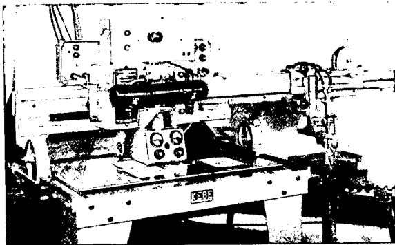
Bild 39. Ultra-Rex-Universalpräzisionsbrennschneidmaschine zum unmittelbaren Abtasten der Striche von Zeichnungsvorlagen (Kjellberg-Eberle GmbH., Frankfurt a. M.)
