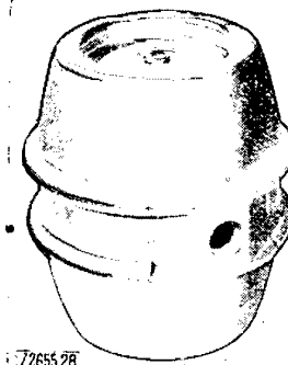
Bild 28 (rechts). Bierfaß aus Leichtmetall. Werkstoff Al-Mg-Si; Argonarc-Schweißung
