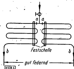
Bild 4: Vertikal unterteilte Rohrschlange
