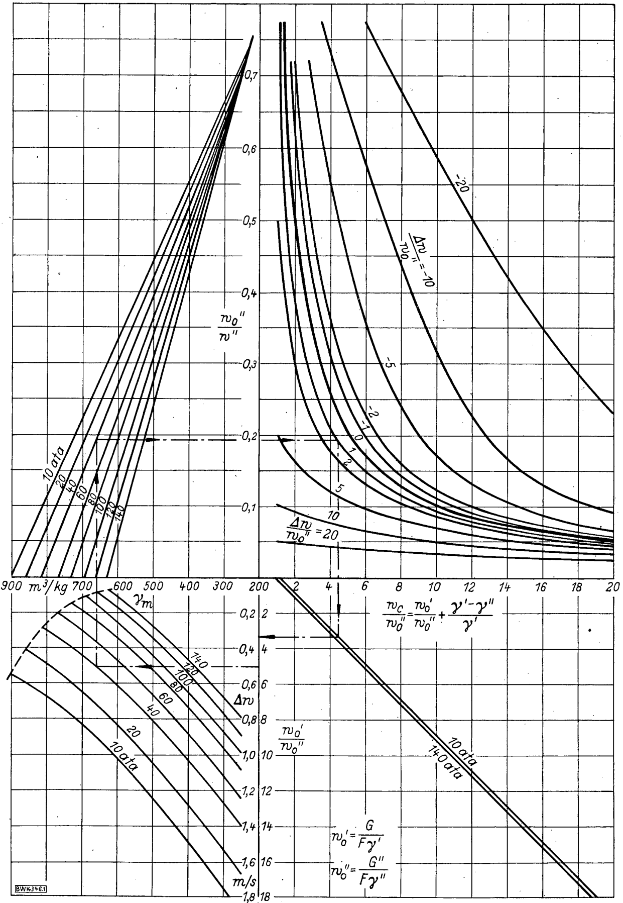
Bild 1. Geschwindigkeiten, Wichte und Dampfvereilung in einem Kesselrohr von 60 mm Dmr.
