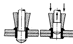
Abb. 31. Hohlrietung nach dem Armstrong-Whitworth-Verfahren.
