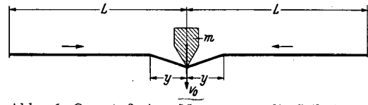
Abb. 16. Querstoß einer Masse gegen die Seilmitte.
