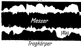
Oberflächenprofil nach betriebsmäßiger Belastung Klappe
