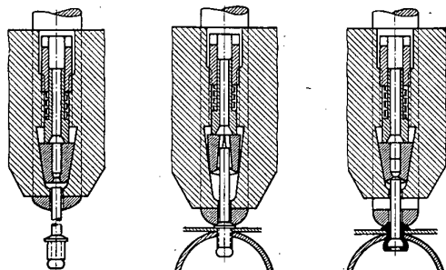
1. Dornniet in die Dornnietzange einführen 2. Dornniet in das Nietloch einführen 3. Niet anziehen bis der Dornschaft anreißt
