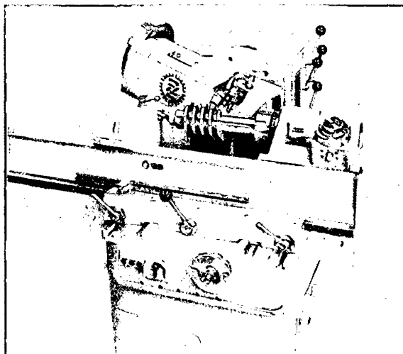
Bild 14. Schneckenfräsmaschine (Zahradfabrik Zuffenhausen) Größter zu fräsender Modul . . . . . 12 Größter Schneckendurchmesser . . . . . 260 mm Größte Fräslänge . . . . . 520 mm Größte Einspannlänge . . . . . 730 mm Antriebsleistung . . . . . 8,3 kW
