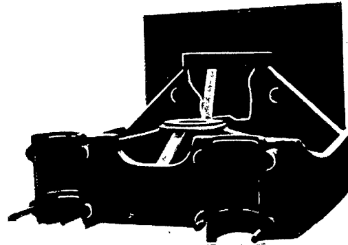
Abb. 11. Die Tischhälfte nach Abb. 10 durch Warmmelzschweißung instandgesetzt. Alte Ausführung durch Rippe verstärkt.
