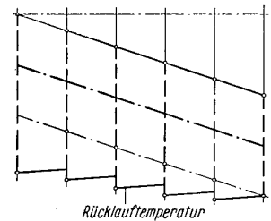
Bild 3. Verlauf der Rücklauftemperaturen nach Rietschel.
