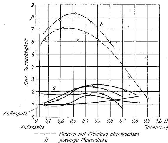
Bild 4. Horizontale Feuchtigkeitsverteilung einiger gut ausgetrockneter Kalksandstein-Außenwände (a), sowie zweier Kalksandsteinwände (b), die infolge Überwachsung mit Weinlaub in ihrer Austrocknung gehemmt waren.
