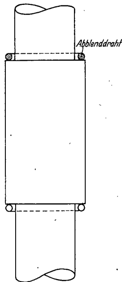
Bild 6. Anordnung der Ablenddrähte bei einer abgesetzten Welle
