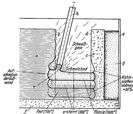
Abb. 6. Der Vorgang einer elektrischen Warmschweißung an einer Bruchwand (links) und einer Formkohlewand (rechts). a Gußeisenwerkstück; b Bruchwand des Gußeisenwerkstückes; c Formkohleplatte; d Formkohlewand; e Formkasten; f untere Formkohleplatte; g Formsand; h Gußeisenelektrode.
