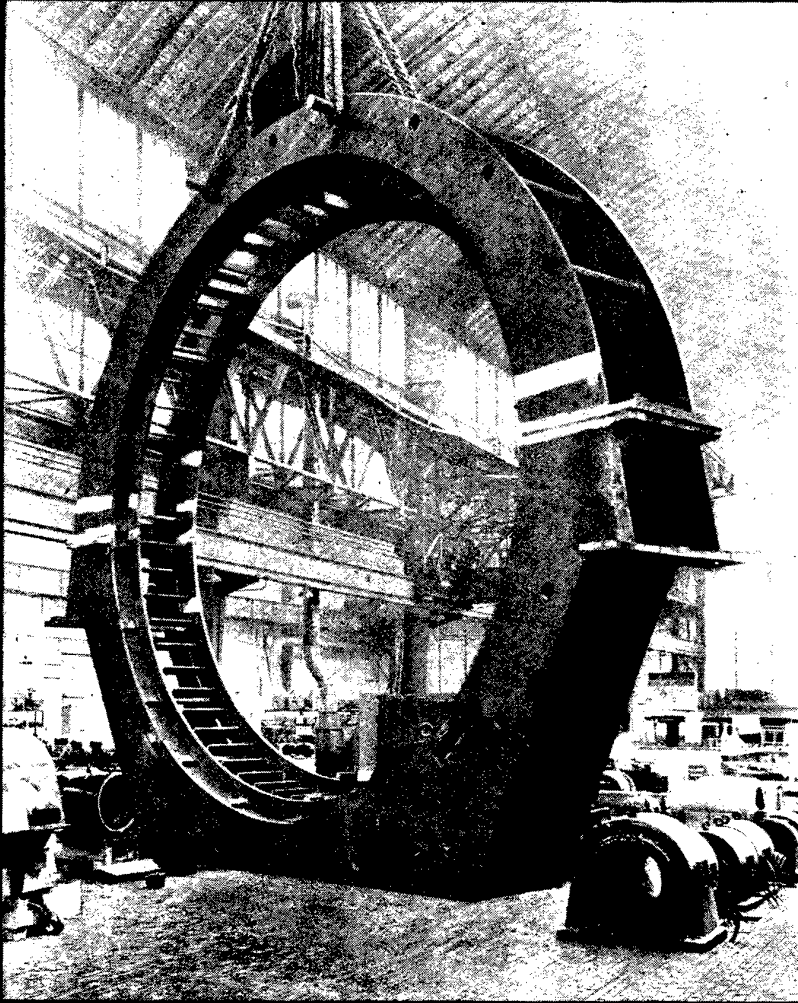
Geteiltes, geschweißtes Gehäuse eines Synchronmotors 2300 kW, 150 U/min
