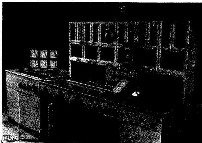
Bild 1. Prüfstand für Elektrizitätszähler.
