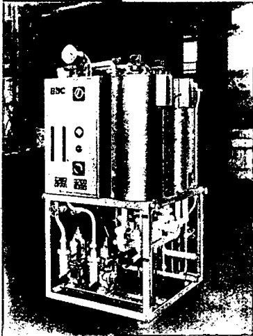
BBC-Schutzgaserzeuger für 10 Nm 3 /h
