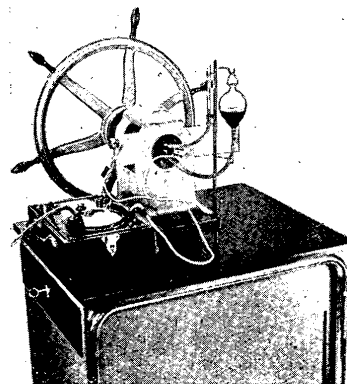
Abb. 2: Elektrische Meßvorrichtung zur Lackprüfmaschine Werkfotos: Erichsen GmbH
