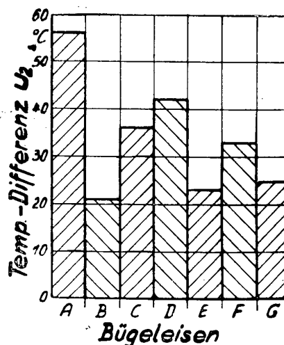
Abb. 13 Unterschied des ermittelten Wirkungsgrades gegenüber den in den NEMA-Vorschriften angegebenen Mindestwerten
