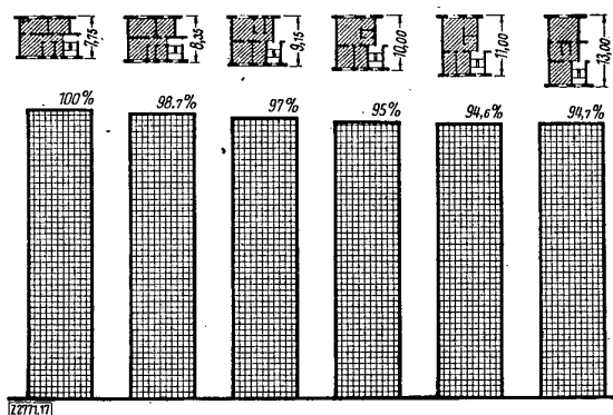
Bild 17. Einfluß der Haustiefe auf die Baukosten gleich großer Wohnungen (Wohnungsgröße 50 m 2 ) in beiderseits eingebautem dreigeschossigen Wohnhause mit zwei Wohnungen je Geschoß.
