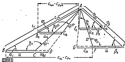
Bild 2. Geschwindigkeitsdreiecke einer Stufe.
