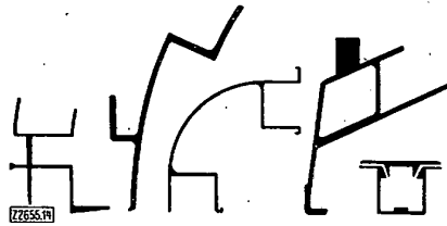
Bild 14 (rechts). Leichtmetall-Sonderprofile für den Fahrzeugbau, entstanden aus der Vereinigung mehrerer Bauelemente zu einem Strangpreß-Querschnitt.
