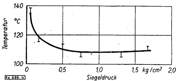
Abb. 4. Abhängigkeit der Temperatur des Heizbandes vom Siegeldruck
