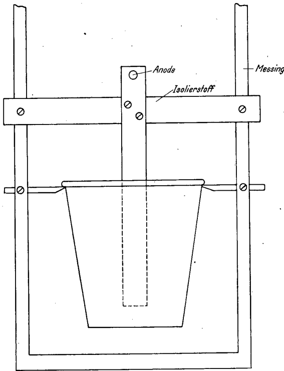
Bild 3. Einhängestell mit Innenanode
