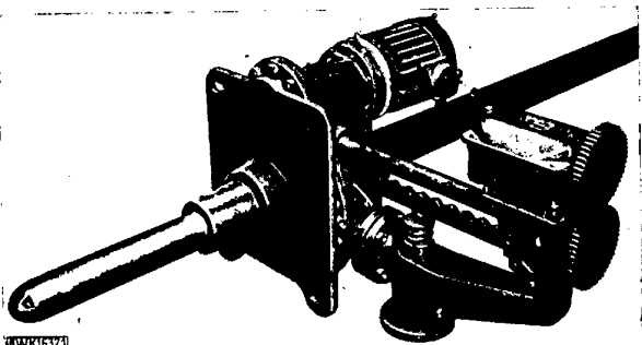
Bild 1. Rußbläser-Automat zur selbsttätigen Steuerung von Blasdüse und Blasdampf bei einem Langvorschubbläser.
