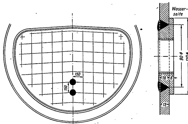
Bild 8 lks., Wendekammerrückwand eines Schiffskessels v. 42 m² Heizfläche; rechts, Eingeschrübte Scheiben zur Aufnahme der Stehbolzen
