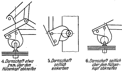
Abb. 25. Dornnietung.
