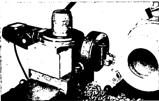
Bild 36. Einkomponentenschnittkraftmesser nach Schallbroch (Schoppe & Faeser GmbH., Minden/Westf.)
