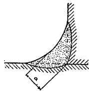
Leichte Kehlnaht
