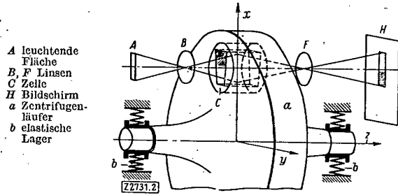
Bild 2. Schema der Optik des Absorptionsverfahrens an einer Zentrifuge der von Tf. Svedberg entwickelten Bauart. Die Bezeichnungsweise (große Buchstaben) ist so gewählt, daß sie mit den entsprechenden Bezeichnungen von Bild 3 bis 6 übereinstimmt.
