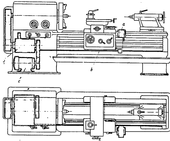
Bild 16. Schematische Darstellung der Universal-Automatik zum Einhalten konstanter Schnittgeschwindigkeiten beim Plandrehen (PIV Antriebe, Werner Reimers KG., Bad-Homburg v. d. H.) a PIV-Universal-Automat, b Übertragungswelle, c Antriebsmotor, d PIV-Getriebe
