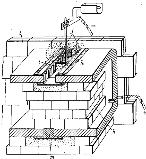
Abb. 15. Schematische Darstellung des letzten Schweißvorganges am Ständer nach Abb. 12. h Klebsand; i Ofenwand; j Kohleplatten; k Mauerwerk; l obere Schweißform; m erste, untere Schweißform
