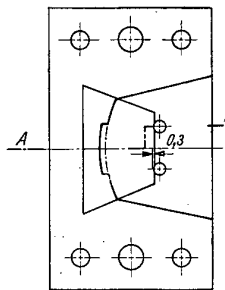
Bild 1 (links) - Lochwerkzeug für maßgenaue Werkstücke a gehärtetes Einsatzstück, b federnde Begrenzungsstifte, c Einlage, d Schnittplatte, e Grundplatte
