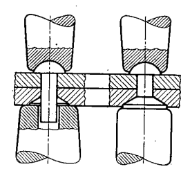
Abb. 10. Anziehen und Schlagen des Flachsenk-Schließkopfes.
