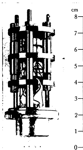
Bild 6 Magnetostriktiver Schwingern für 150 kHz, Gehäuse abgenommen. Die Schwingern sind mit Rimlocksckel ausgerüstet
