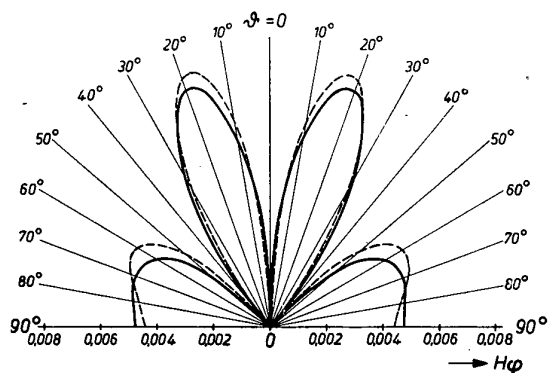
Bild 3 Strahlungsdigramm der magnetischen Feldstärke - - - Spaltbreite \Delta \rho = 0 — Spaltbreite \Delta \rho = 0,1 \rho_0 } \left( \frac{2 \pi \rho_0}{\lambda} = 6 \right)
