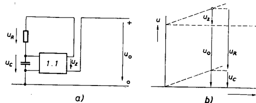
Bild 3 Mittelaufende Ladespannung
