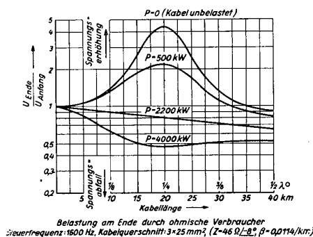
Bild 3 Steuerspannungsabfall an 10 kV-Kabel mit Berücksichtigung der Kabeldämpfung.
