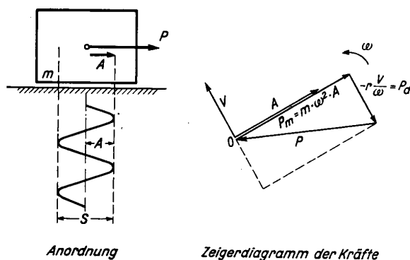
Bild 1 a) Anordnung; b) Zeigerdiagramm der Kräfte
