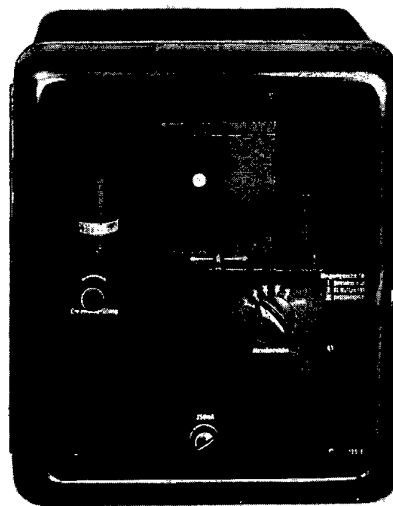
Bild 4 Kompensationsverstärker, Ein- und Aufbaugerät für 220 V Wechselstromnetzanschluß
