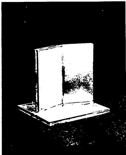
Bild 6 Löt muster — Aluminium, 5 mm — mit Ultraschall und reinem Zinn gelötet
