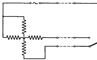
Bild 4 Schaltung des Schrittschaltmotors mit 3 Zuleitungen
