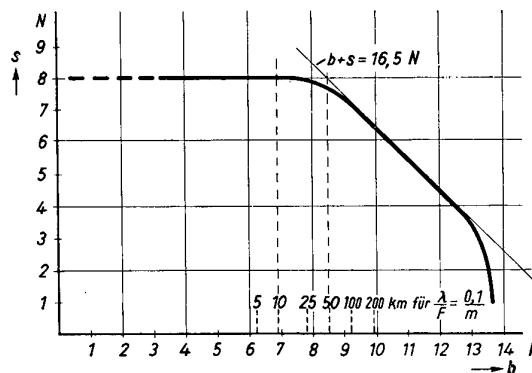
Bild 6 Geräuschabstand s im Sprachkanal über der Streckendämpfung b für eine Richtfunkstrecke
