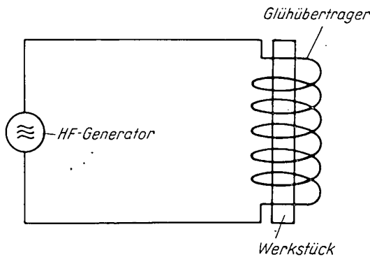
Bild 1 Prinzip einer Hochfrequenzglühanlage
