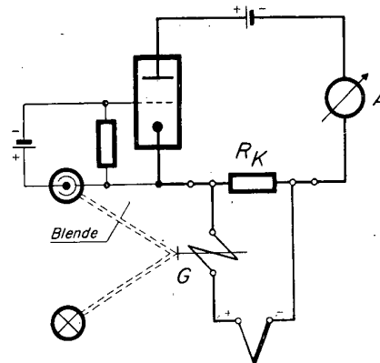
Bild 2 Grundsaltung eines Fotozellenkompensators
