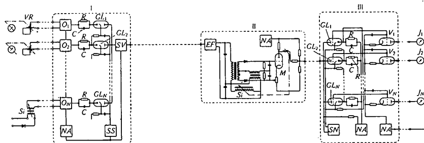
Bild 8 Vereinfachtes Prinzipschaltbild des Frequenz-Variations-Fernmeßkanales kombiniert mit zyklischer Rapidumschaltung
