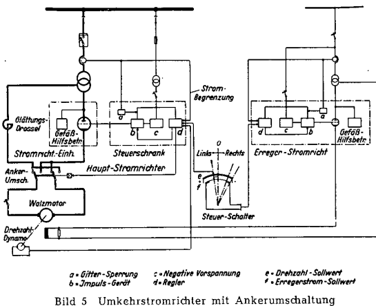
Bild 5 Umkehrstromrichter mit Ankerumschaltung
