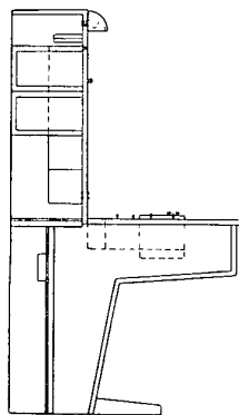
Bild 6 Schrankförmiger Stichleitungs-Fernplatz (Seitenansicht)
