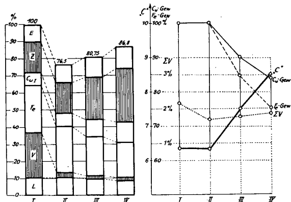
Bild 3 Modellausnutzung und Verluste an einem Turbogenerator 50 MVA ( \cos \varphi = 0,8 )
