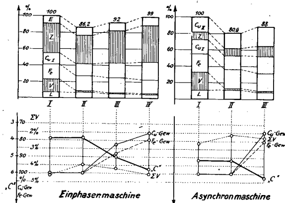
Bild 7 Modellausnutzung und Verluste an einem Netzkupplungs-umformer 24 MVA ( \cos \varphi = 0,75 )
