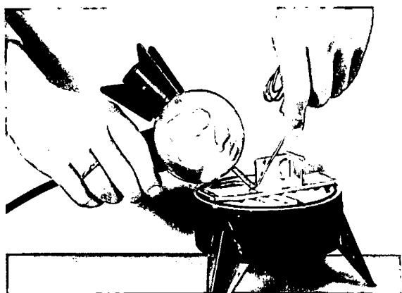
Bild 5 Griffel-Lötverfahren mit Vorwärmplatte
