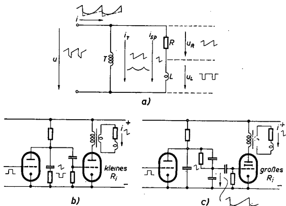
Bild 2 Einfluß des Transformators bei großem und kleinem R_i
