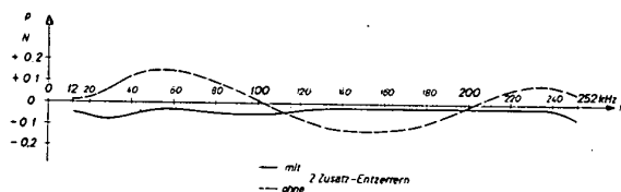
Bild 6 Restverzerrung einer 120 km langen V 60-Strecke (6 Verstärkerfelder)
