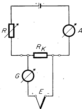
Bild 1 Kompensationsschaltung nach Lindeck-Rothe
