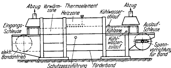
Bild 1 Schutzgas-Durchlaufofen
