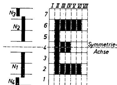
Bild 4 Prinzip der Einzelenschrift
