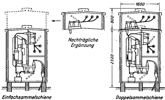
Bild 8 Ergänzung einer Schaltanlage mit einem Sammelschienen-system durch eine zweite Sammelschiene
