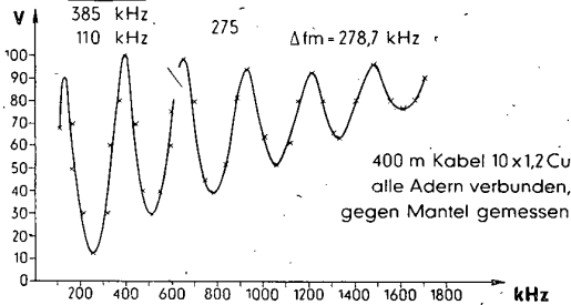
Bild 6 Beispiel einer Kabelmessung
