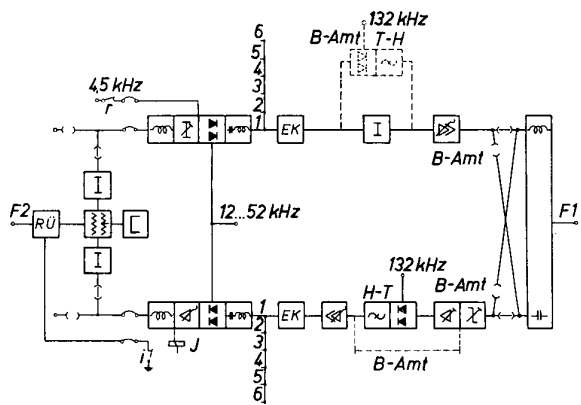
Bild 10 Netzgruppen-Tf-System Z 6 N; Blockschemata der Endstelle A
