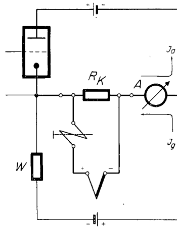
Bild 3 Gegenstromprinzip
