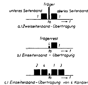
Bild 1 Lage der Seitenbänder zum Träger bei Zwei- und Einseitenband-Übertragung
