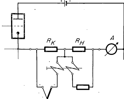
Bild 6 Verminderung des Richtmomentes durch Drehspule mit Hilfswicklung
