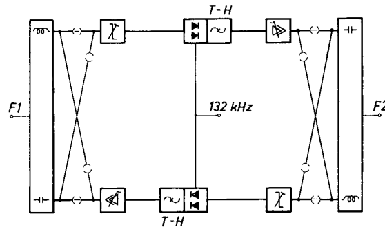
Bild 11 Netzgruppen-Tf-System Z 6 N; Blockschemata eines Zwischenverstärkers (T—H)
