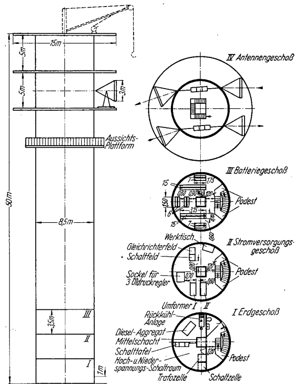
Bild 2 50 m-Dezimeter-Antennenturm
