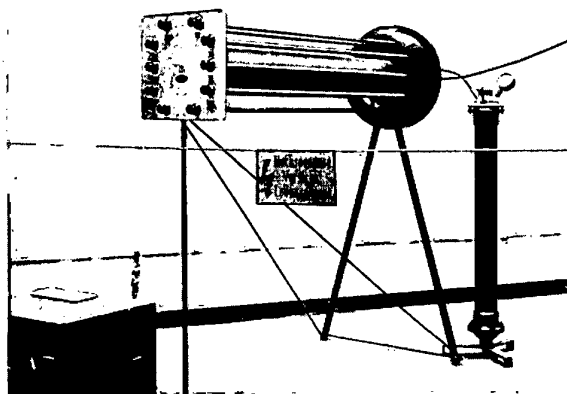
Bild 3 Hochspannungsbrücke für tg \delta -Messung an Kabelanlagen
