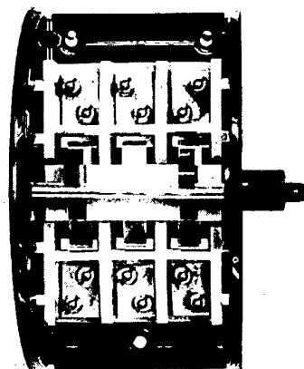
Bild 7: Calor-Emag-Last-Ausschalter auf Steatitkörper in Stahlblechmantel und -abdeckung, Typ LA — 100 A 750 V, Abdeckung abgenommen
