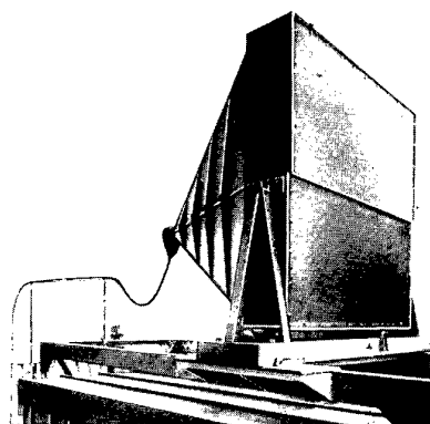
Bild 5 Hornstrahler mit elektrischer Linse für 12 cm-Richtfunk-Verbindungen
