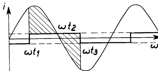
Bild 2 Wirkungweise der Strombegrenzung bei abnehmendem Steuerstrom für den Transduktor nach Bild 1
