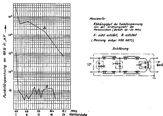
Bild 4 Funk-Entstörung eines Ultraschallgerätes
