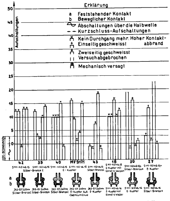
Bild 5 Schaltversuche mit verschiedenen Kontaktmaterialien und -formen
