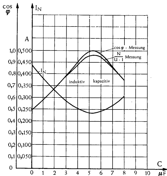
Bild 4 Leistungsfaktormessung an einer 40 W-Leuchtstofflampe mit Drosselspulen-Vorschaltung und verschieden großen netzparallelen Kondensatoren ( C = 0 \dots 8 \mu\text{F} ). Messung mit Leistungsfaktorzeiger und mit Leistungs-, Strom- und Spannungsmesser
