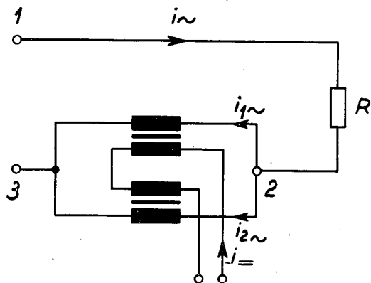
Bild 3 Grundschaltung des Transduktors mit Strombegrenzungssteuerung für wechsellspannungsfreien Steuerkreis
