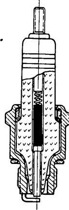
Bild 5 Bosch-Widerstandskerze
