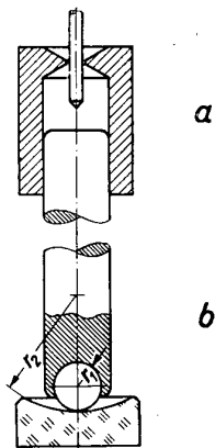
Bild 1 Ober- und Unterlager, a) Halslager, b) Einfachlager
