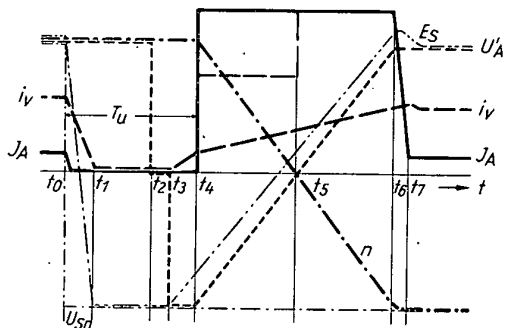
Leerlaufreversiervorgang ohne Feldverstellung
