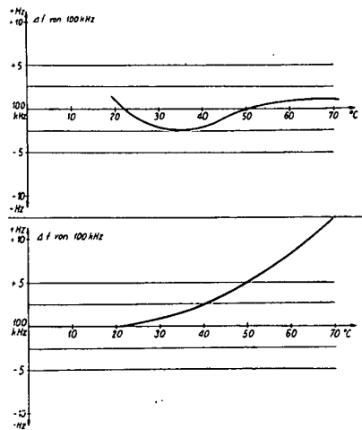
Bild 7 Vergleich des Temperaturganges ohne Thermostat bei 100 kHz für magnetostriktiven Schwingern (oben) und Quarz mittlerer Qualität (unten).
