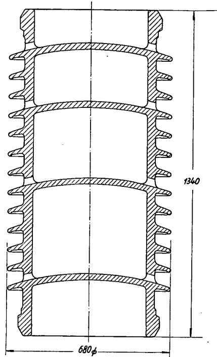
Bild 8 110 kV-Stützer mit belüfteten Zwischenräumen
