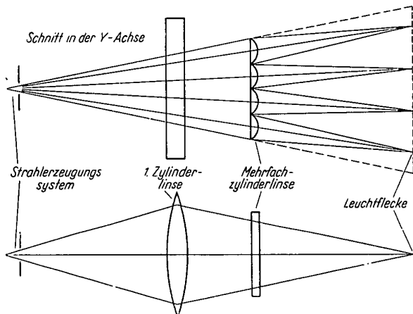
Bild 2 Strahlteilung einer Mehrstrahlröhre mit gekreuzten Zylinderlinsen
