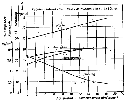
Bild 3 Einfluß des Abziehgrades auf die Werkstoffeigenschaften bei nach dem Herunterziehverfahren hergestellten Aluminiummängeln
