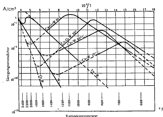
Bild 1 Emissionskennlinien von Wolfram mit einatomarer Cäsium-Schicht
