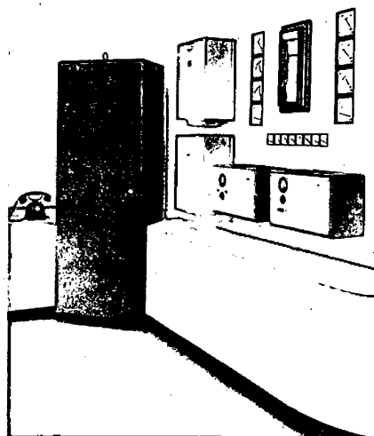
Bild 10 Gesamtaufwand einer Übertragungsanlage nach dem Einseitenbandverfahren für 1 Telephoniekanal mit automatischer Wahl und gleichzeitiger Übertragung von 8 Meßwerten. Links: Trägerschrank, Senkrecht: Hauszentrale für 10 Teilnehmer, sowie Verbindungsgerät für Fernwahl mit Fernkennziffer und Vierdrahtumschaltung. Waagerecht: Fernmeßempfänger und zyklisches Umschaltgerät für 8 Fernmeßkanäle. Anzeigeelemente: je 2 Instrumente in verschiedener Größe pro Wert, ferner eine Summierung registrierend für 2 der Meßwerte
