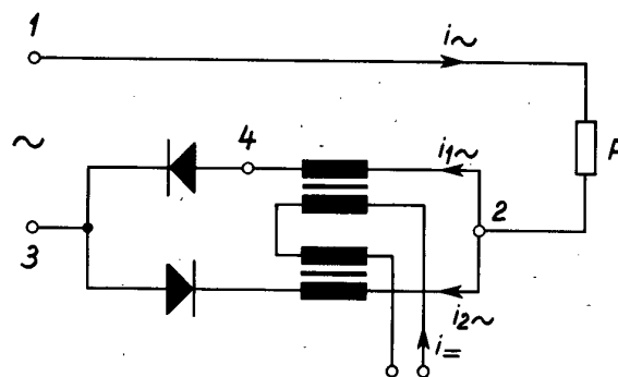
Bild 5 Grundschaltung des Transduktors mit Sättigungswinkelsteuerung für Arbeitswechselstrom
