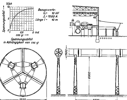
Bild 6 Rohr-Schiene Kanal (10 kV) als fabrikfertige Konstruktionseinheit. Darstellung des Spannungsabfalls in Abhängigkeit vom Leistungsfaktor
