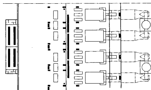
Bild 6 Eigenbedarfsanlage von Kraftwerken, offene und gekapselte Bauform
