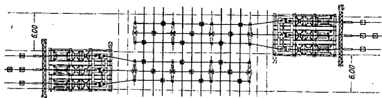
Bild 5 100 kV-Schaltanlage nach der Staffelbauform mit Einpunkt-Scherentrennschaltern und drei Sammelschienensystemen. Anlagenbreite bei vier Sammelschienensystemen beträgt 62 m bei einer Felderteilung F von nur 6 m
