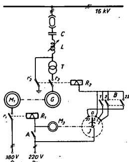
Bild 6 Prinzipschaltbild einer Sendeanlage
