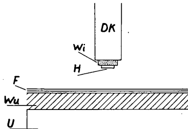
Bild 2 Querschnitt durch einen Wärmeimpulsstempel mit Unterlage bei Wärmeimpulsschweißung
