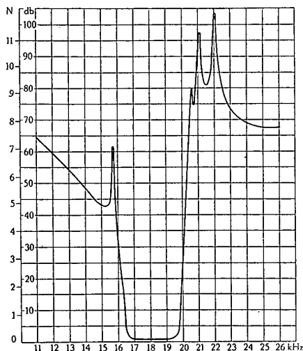
Bild 5 Dämpfungsverlauf eines Filters zur Ausfilterung des 2. Seitenbandes im Zwischenfrequenzkanal eines Einseitenbandsenders. Kernmaterial Ferrox-Cube.
