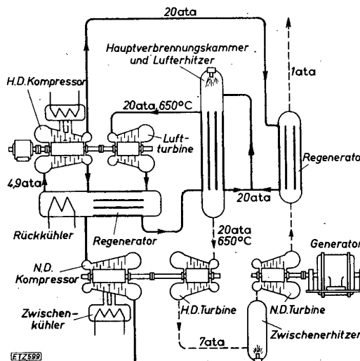
Bild 7. Aufbau des Gasturbinenkraftwerks für 2000 kW in Weinfeldern.
