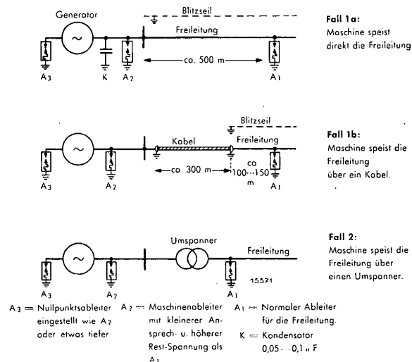
Bild 12 Anordnung von Überspannungsableitern an Generatoren
