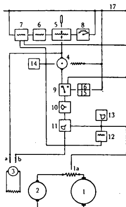
Bild 7 Prinzipschaltbild der Rapid-Exakt-Steuerung für Gleichstrom-Fördermaschinen
