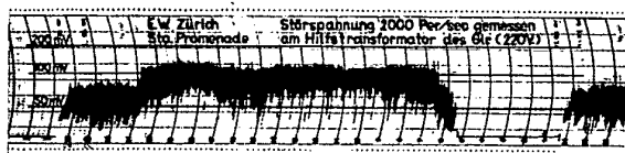
Bild 1 Störspannungsdiagramm für 2000 Hz ± 100 Hz
