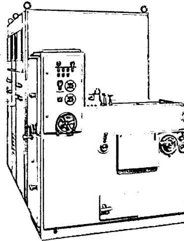
Bild 10 Zahnradhärtemaschine Typ 1031 zur Härtung von Zahnradern nach dem Zahnlückenverfahren. Modul 2-6
