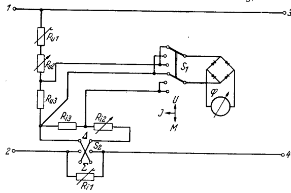
Bild 2 Prinzipschaltung zur Erzeugung der Summen- oder Differenzspannung
