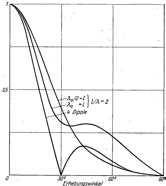
Bild 6 Vertikaldiagramm der Feldstärke einer Rohrschlitzantenne und einer gleich hohen Dipolantenne
