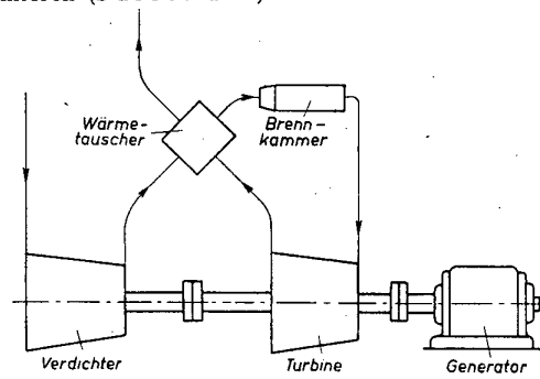
Bild 1. Schema des offenen Arbeitsprozesses.
