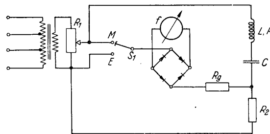
Bild 8 Vereinfachte Schaltung des Frequenzmessers
