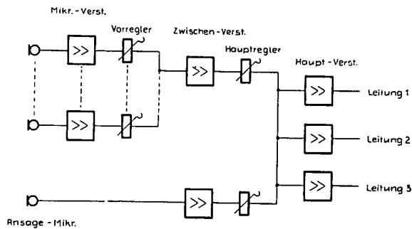
Bild 5 Schema der Studioverstärkung
