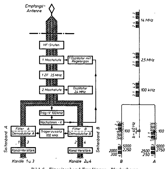
Bild 6 Einseitenband-Empfänger. Blockschema
