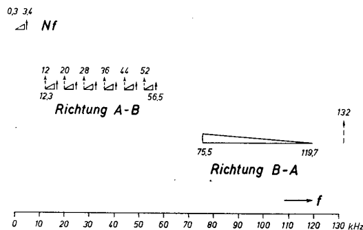
Bild 9 Netzgruppen-Tf-System Z 6 N; Frequenzschema
