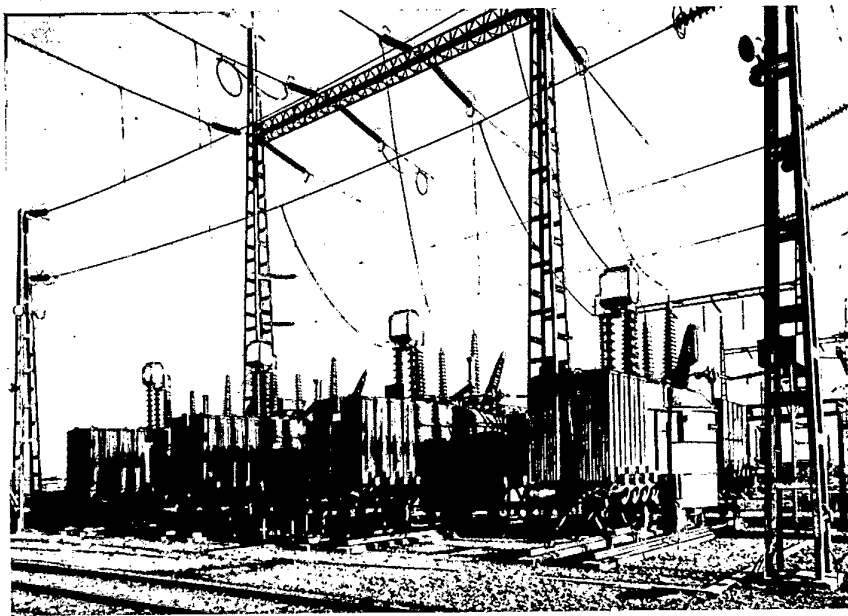
Bild 11 Transformorengruppe von 120 MVA mit drei Einphasentransformatoren je 40 MVA, dazu ein Reservetransformator, 220/112 + 15 x 1,7/10 kV mit eingebautem Stufenlastschalter (BBC)
