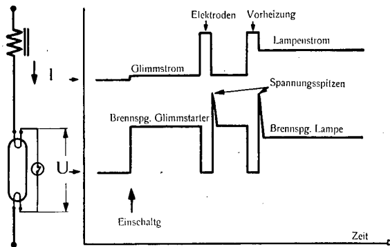
Bild 3 Vorheiz- und Zündvorgang einer Leuchtstofflampe Darstellung der Strom- und Spannungshöhe vom Einschalt Augenblick bis zum Brennen der Lampe (etwa 1 bis 3 Sekunden). (Die Lampe zündet in diesem Beispiel erst nach der zweiten Vorheizung.)
