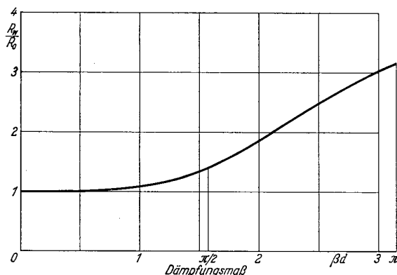
Bild 3 Verhältnis des Wechselstromwiderstandes zum Gleichstromwiderstand eines bandförmigen Leiters bei verschiedenem Dämpfungsmaß. Dämpfungsmaß \beta d ist gleich dem Verhältnis der Bandstärke d zur Eindringtiefe 1/\beta .
