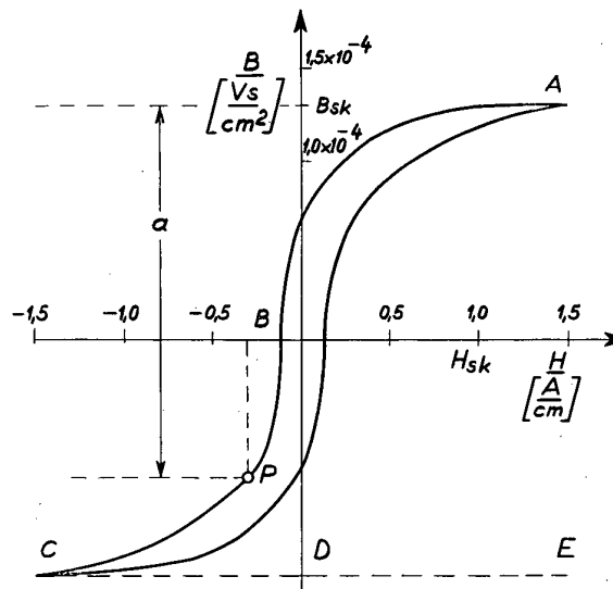
Bild 7 Hystereseschleife eines für Transduktoren verwendeten Spezial Eisens
