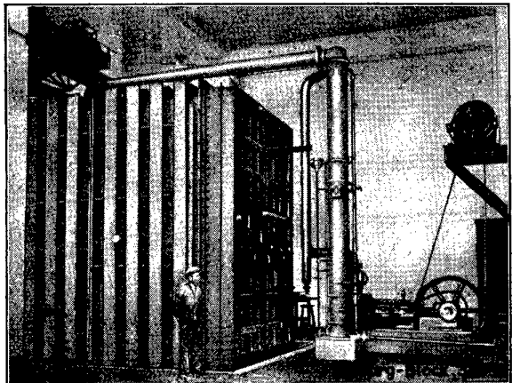
Großer Vakuum - Transformatoren - Trockenschrank
