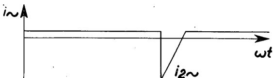
Bild 4 Wirkungsweise der Strombegrenzung bei dem Transduktor nach Bild 3
