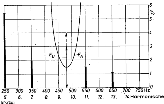
Bild 2. Typisches Oberwellenspektrum eines Dreiphasennetzes und Ansprechbereich der Empfangsgeräte von L & G-Überlagerungs-Fernsteueranlagen.
