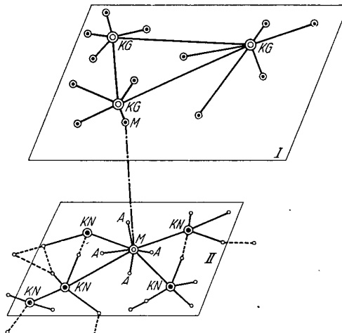
Bild 2 Netzgruppenanordnung im Fernmeldenetz der Bundesbahn (Basa)
