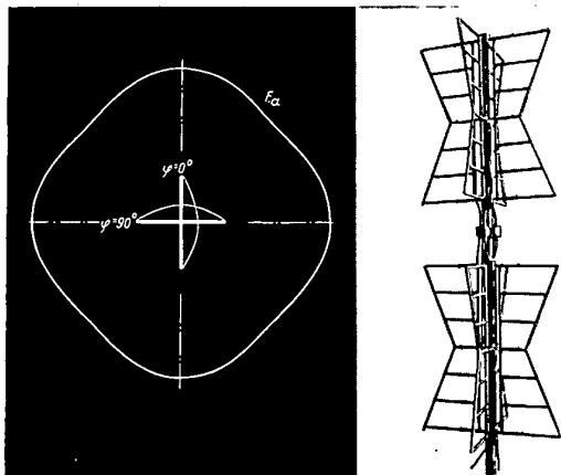
Bild 3 Fernsehantenne (Super-Turnstile)
