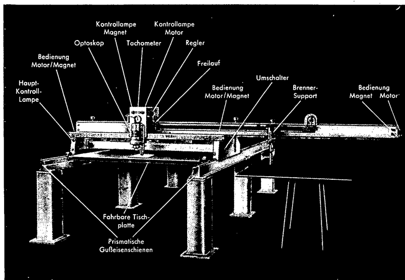
Abb. 5: Universal-Brennschneidmaschine
