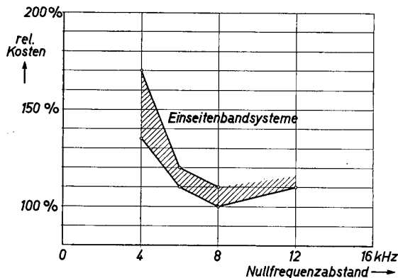
Bild 8 Rel. Investierungskosten für Tf-Endgeräte als Funktion des Nullfrequenzabstandes (50...100 Sprechwege)
