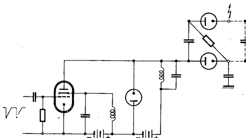
Bild 8 Transformatorfreie Horizontalablenkungsschialtung
