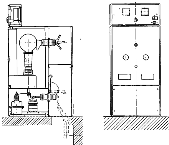
Bild 6 Geschottete Expansionsschaltereinheit, Reihe 10, 600 A, 200 MVA, Leistungsschalter und Wandler ausfahrbar
