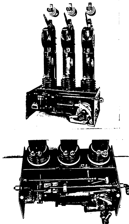
Bild 2 Innenraum-Expansionschalter, 10 kV, 400 A, 100 MVA
