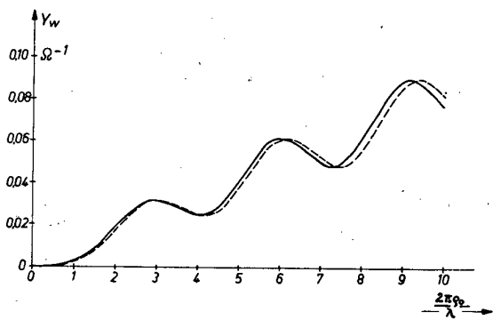
Bild 6 Wirkleitwert am Ringspalt in Abhängigkeit von \frac{2\pi\rho_0}{\lambda}
