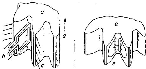
Bild 9 Induktive Zahnlückenhärtung
