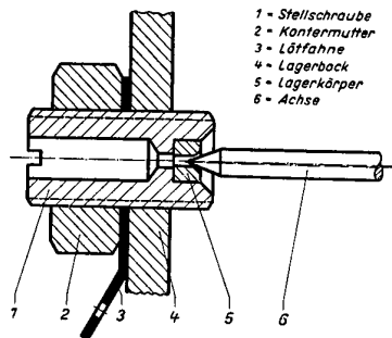
Bild 2 Kontakt-abnahme durch Spitzen-lagerung
