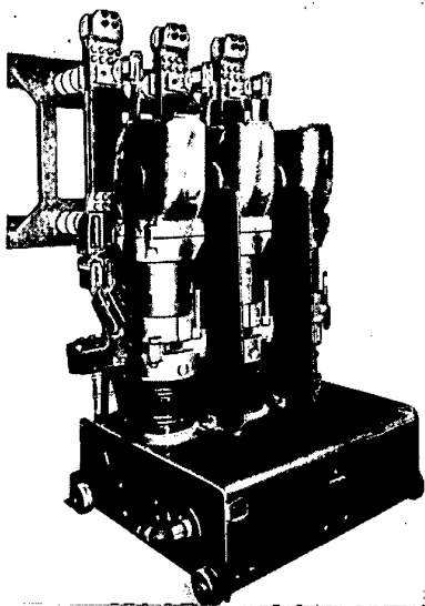
Bild 3 Innenraum-Expansionschalter, 10 kV, 4000 A, 1000 MVA
