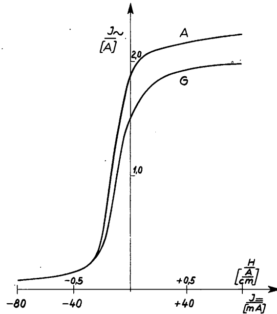
Bild 12 Regelkennlinie des Transduktors nach Bild 11 mit Sättigungswinkelsteuerung für Schaltung nach Bild 5 (Kurve A) und nach Bild 8 (Kurve G).
