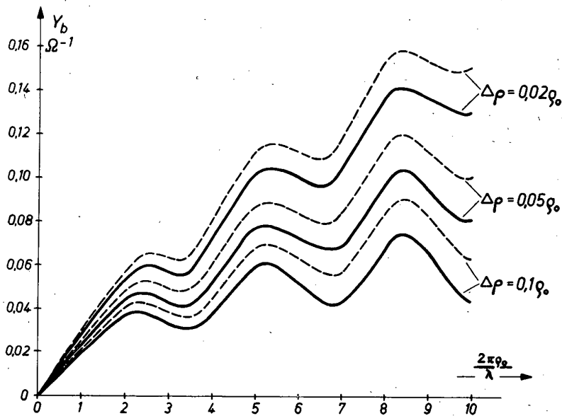
Bild 7 Blindleitwert am Ringspalt in Abhängigkeit von \frac{2\pi\rho_0}{\lambda} für die Spaltbreiten \Delta\rho = 0,1\rho_0 ; \Delta\rho = 0,05\rho_0 ; \Delta\rho = 0,02\rho_0 ; - - - scharfkantige Spaltränder; ..... homogene Feldverteilung im Spalt
