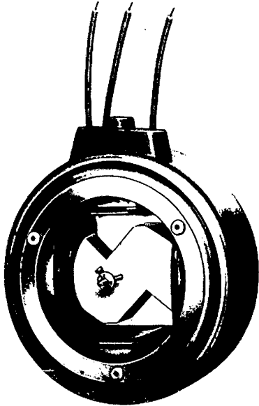
Bild 5 Schrittchaltmotor mit durchbrochener Seitenwand
