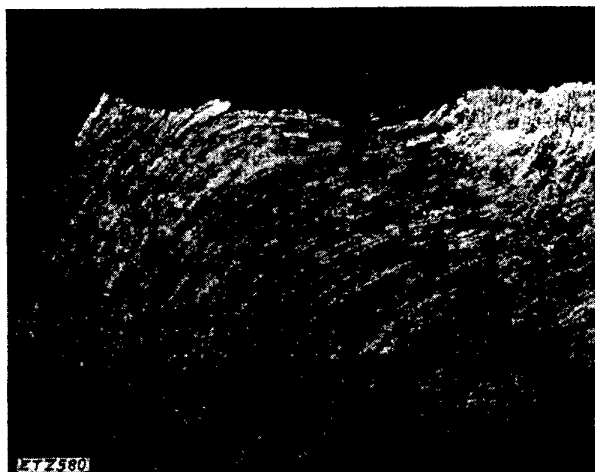
Bild 11. Teilgebiet aus der Kontaktrandzone von Bild 10, geätzt ( V = 75 ).
