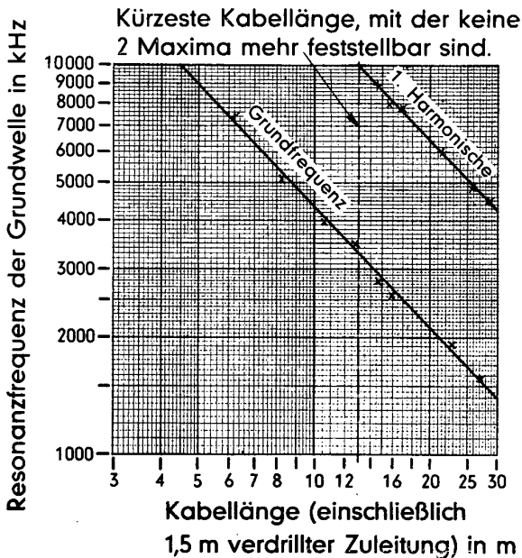
Bild 9 Auswertungs-Nomogramm
