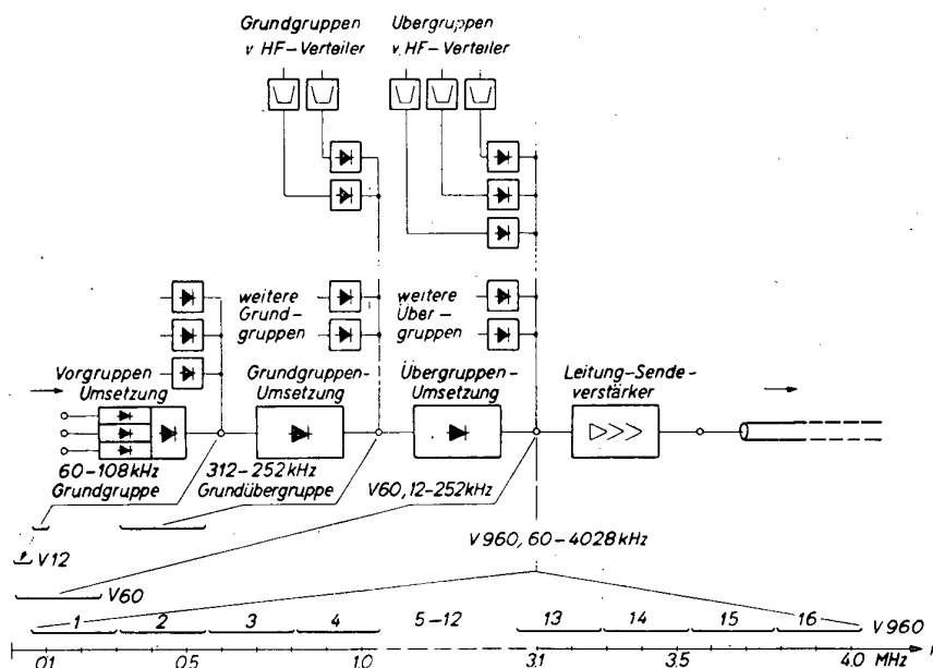
Bild 2 Prinzipstromlauf der Endgeräte und Frequenzschema
