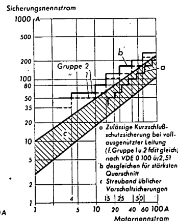
Bild 13 Sicherungen vor Motorschutz
