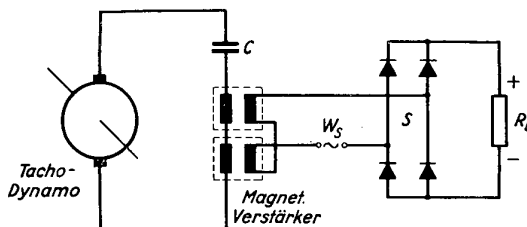
Bild 7 Meßwertumformer für Beschleunigung
