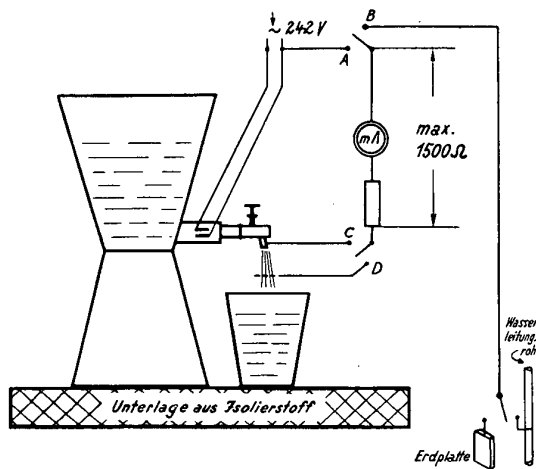
Bild 1 Messung des Übergangstromes gem. VDE 0720 § 22 c Versuchsanordnung
