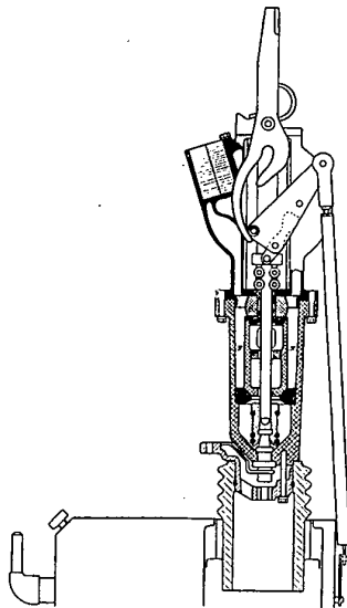
Bild 4 Schnitt durch einen 10 kV-Expansionschalterpol
