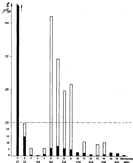
Bild 2 Feldstärken der abgestrahlten Harmonischen eines KW-Therapiegerätes in \mu\text{V}/\text{m} in 300 Abstand vom Gerät (Maximalwerte). Grundfrequenz: f = 27,12 \text{ MHz}
