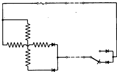
Bild 6 Schaltung des Schrittchaltmotors in Halbwellenschaltung
