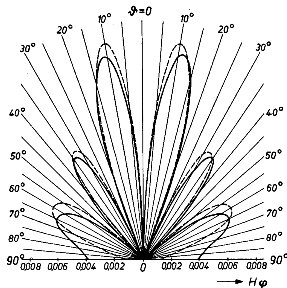
Bild 4 Strahlungsdigramm der magnetischen Feldstärke - - - Spaltbreite \Delta \rho = 0 — Spaltbreite \Delta \rho = 0,1 \rho_0 } \left( \frac{2 \pi \rho_0}{\lambda} = 10 \right)
