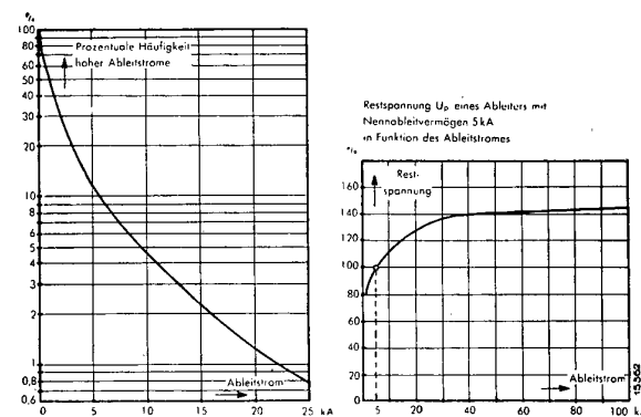
Bild 7 Häufigkeit hoher Ableitströme und Restspannung eines Überspannungsableiters
