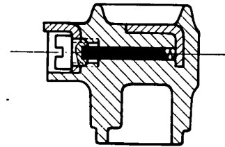
Bild 6 Verteilerfinger mit eingebautem Widerstand
