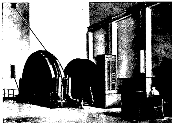
Bild 1 Einhebelssteuerstand und Fördermotor von 3030 kW bei 51 U/min mit Fremdbelüftung, für 680 V, bei 4700 A Nennstrom
