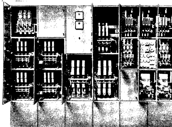
Bild 16 Mehrstöckige Niederspannungs-Schaltanlage in raumsparender Anordnung
