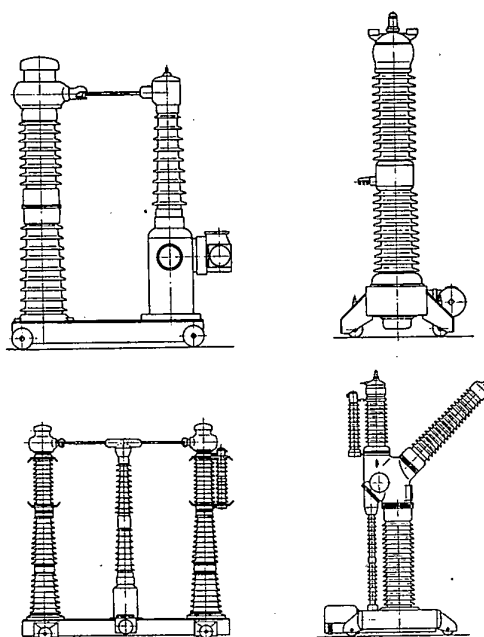
Bild 7 Freiluft-Expansionsschalter, Entwicklung der Bauform oben: Schalter für 60 und 110 kV, unten: Schalter für 220 kV.
