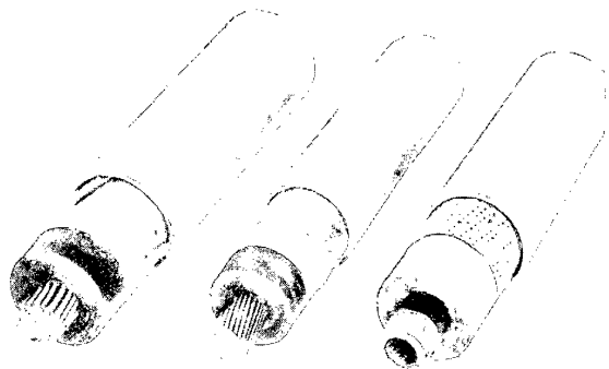
Bild 9 Hochspannungskabel mit Aluminiummantel für Betriebsspannungen bis zu 150 kV
