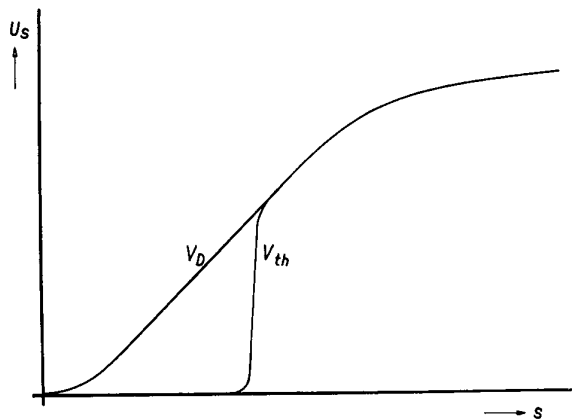
Bild 4 Thermischer und dielektrischer Festigkeitsanstieg bei Leistungsschaltern
