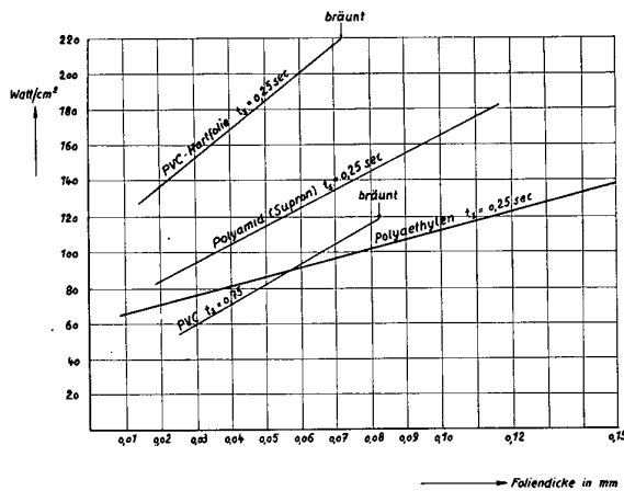
Bild 8 Leistungsbedarf in Watt/cm 2 bei Wärmeimpulsschweißung für verschiedene Thermoplaste und Foliendicken
