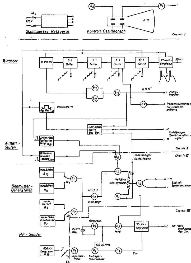
Bild 2 Fernseh-Prüfender GM 2657; Blockschaltbild
