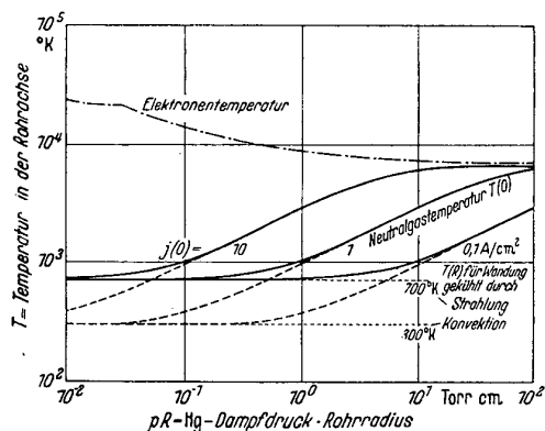
Bild 2 Neutralgastemperatur in der Achse eines Entladungsröhres
