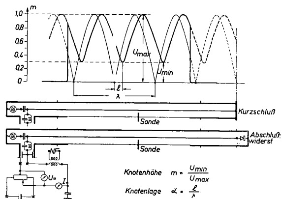
Bild 4 Widerstandsmessung (schematisch)
