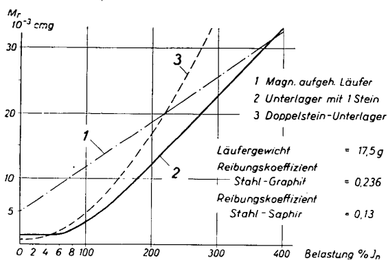
Bild 5 Reibmomente verschiedener Lagerarten in Abhängigkeit von den Radialkräften
