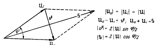
Bild 1 Vektorielle Darstellung von Summen- und Differenzspannung bei amplitudengleichen Vergleichsspannungen
