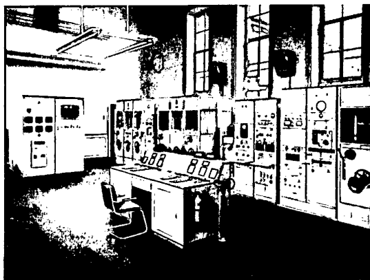
Bild 4 20 kW-Sender mit Schaltpult
