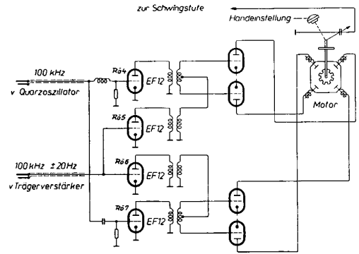
Bild 7 Frequenznachstimmung, Prinzipschaltung
