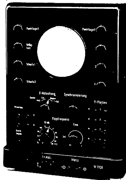
Bild 4 Vierstrahl-Oszillograph
