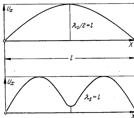
Bild 4 Schlitzspannung U_x über der Schlitzlänge l einer Rohrschlitzantenne (ohne Berücksichtigung der Dämpfung)
