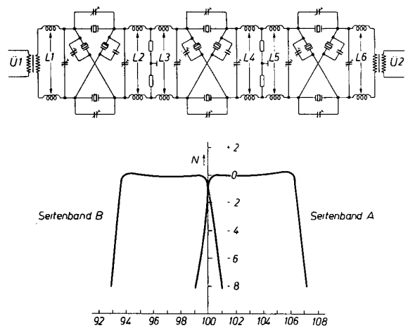
Bild 8 Seitenband-Quarzfilter, Prinzipschaltung
