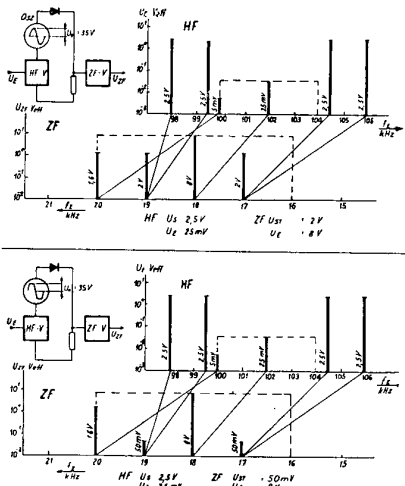
Bild 3 In einem Empfänger bei der 1. Frequenzumsetzung entstehende Störspannungen der Gruppe f_0 \pm (2f_2 - f_1) bei Vorhandensein von 4 benachbart liegenden Sendefrequenzen. Bild 3 oben bei sinusförmiger Umsetzspannung. Bild 3 unten bei trapezförmiger Umsetzspannung. f_0 = Umsetzfrequenz, f_1, f_2 = Störfrequenzen.
