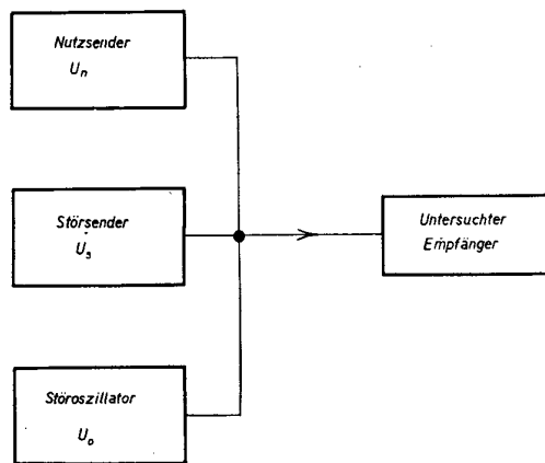
Bild 1 Nachbildung der Modulationsübernahme eines Störsenders durch drei an einen Empfänger angeschaltete Meßsender
