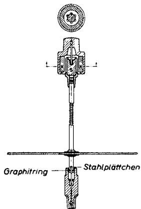
Bild 4 Magnetische Läuferaufhängung
