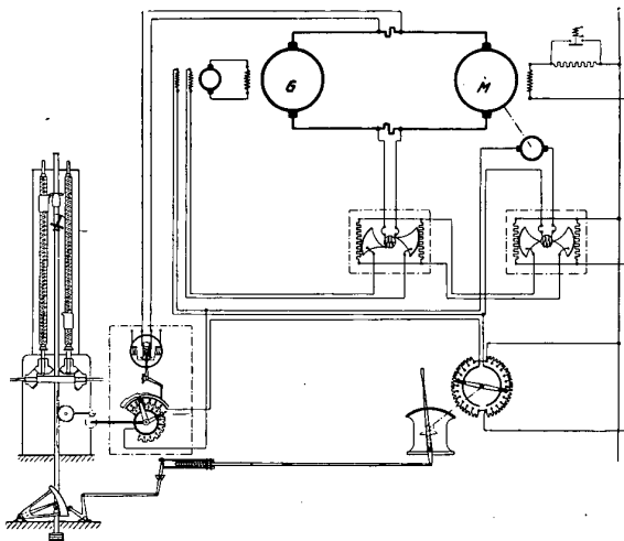
Bild 3 Rapid-Exakt-Steuerung, Prinzip der Drehzahlregelung und Strombegrenzung
