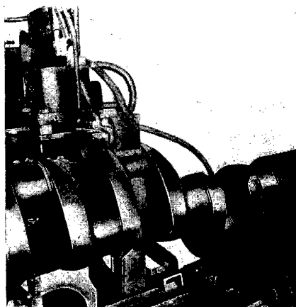
Bild 7 Induktive Kurbelwellenhärtung nach dem Brennlinsenverfahren. Gesamtansicht
