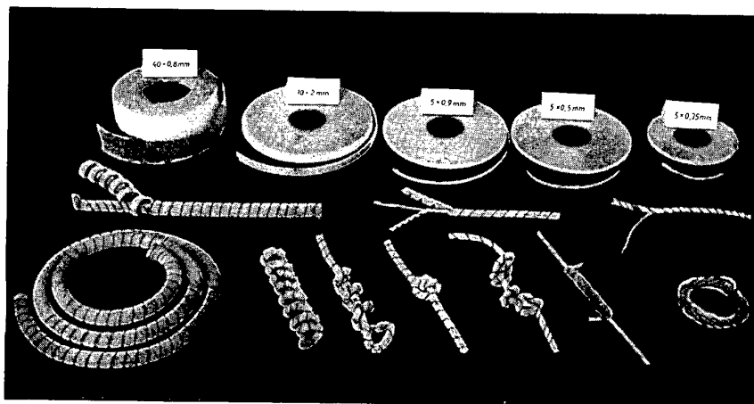
Bild 7 Auswahl von Fäden aus Polystyrolschaumstoff und daraus hergestellte Halbfabrikate von Kabeln und Leitungen
