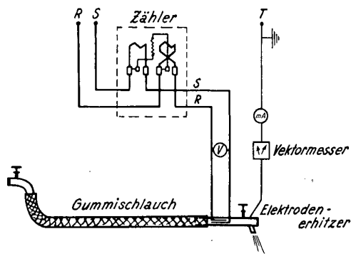
Bild 3 Ermittlung der Phasenlage von Übergangstrom und Spannung im Dreileiternetz ohne Nulleiter, Versuchsanordnung
