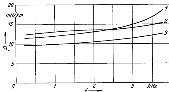
Bild 10 Gegenüberstellung der Dämpfungskurven mit L = 80/40 mH und s = 1,7 km bespulter Kabelleitungen in Sternverteilung:
