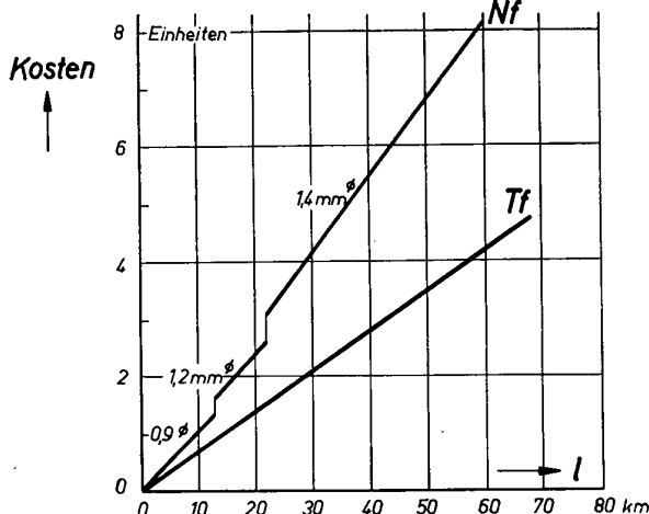
Bild 6 Kosten von Nf- und Tf-Kabeln als Funktion der Kabellänge; 42 Sprechwege
