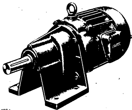
Bild 4: Drehstrom-Stirnräder-Getriebemotor der Eberhard Bauer GmbH. größten von 0,6 ... 160 kW gebaut werden. Außerdem werden Gleichstrommotoren und Spezialmaschinen für verschiedene Zwecke hergestellt.
