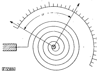
Bild 1. Bimetall-Thermometer.
