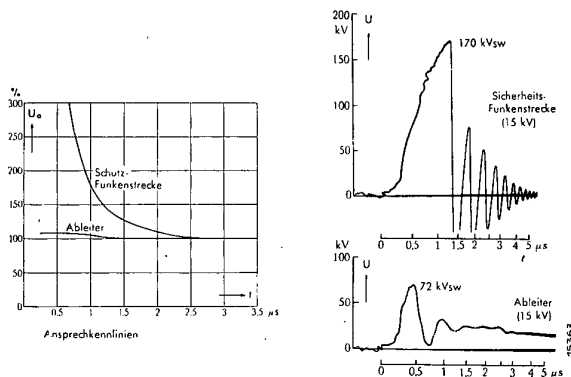
Bild 6 Ansprechkennlinie von Ableiter und Schutzfunkenstrecke
