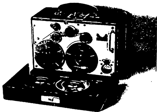
Bild 7 Tragbares Magnetofon
