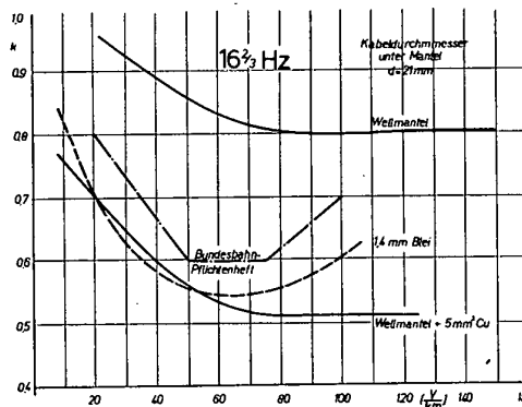
Bild 5 Mantelenschutzfaktor bei Bewehrung mit Spezial-Eisenbändern 30x0,5 mm
