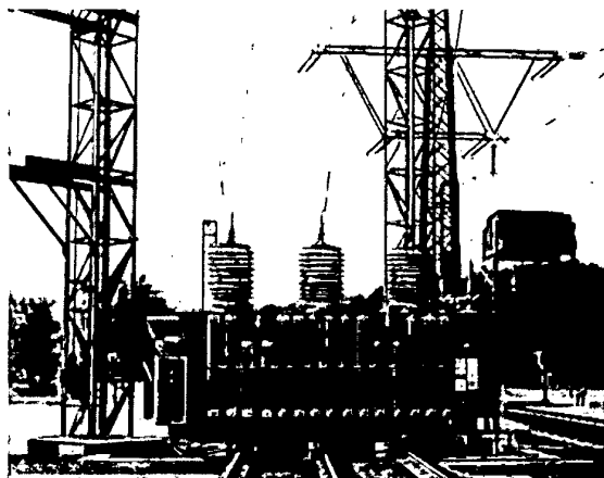
Bild 10 Regeltransformator in Sparschaltung 100 (12,2) MVA, 110/110 ± 8 × 1,5 kV (AEG)
