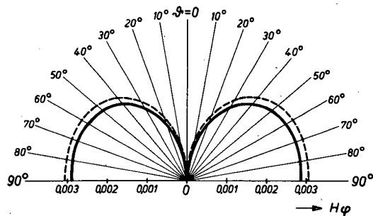
Bild 2 Strahlungsdiagramm der magnetischen Feldstärke - - - Spaltbreite \Delta\rho = 0 — Spaltbreite \Delta\rho = 0,1 \cdot \rho_0 } \left( \frac{2 \pi \rho_0}{\lambda} = 2 \right)
