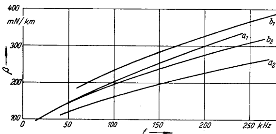
Bild 8 Dämpfung von sternverseilten Tf-Kabelleitungen mit 1,2 mm-Cu-Adern bei 20°C:
