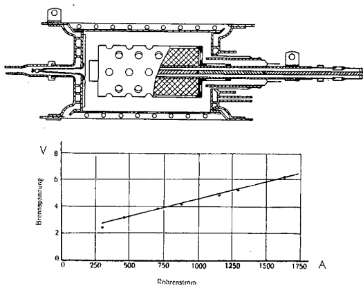
Bild 5 Cäsium-Stromrichter
