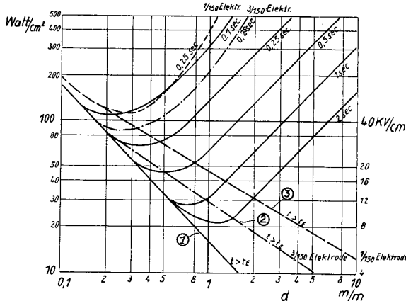
Bild 1 Schweißleistung ( W/cm^2 ) bei HF-Schweißung in Abhängigkeit von Foliendicke, Schweißzeit und Elektrodenbreite. Feldstärkemaßstab gilt für 40 MHz. Elektrodenbreite: ① 20 mm, ② 3 mm, ③ 1 mm
