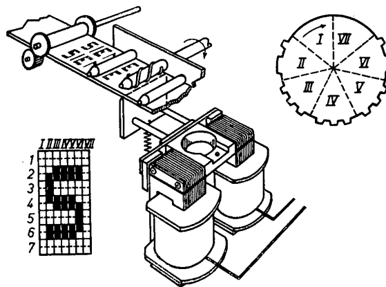
Bild 1 Prinzip des Siemens-Hell-Verfahrens
