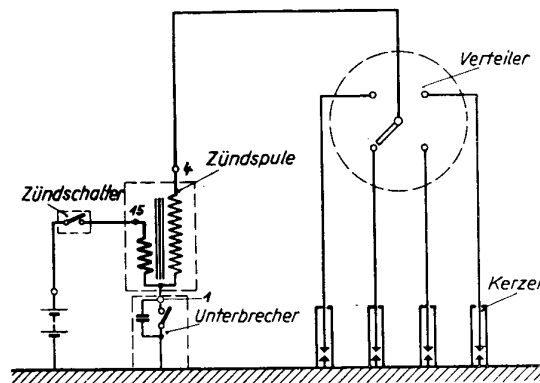
Bild 1 Schema einer Batteriezündanlage
