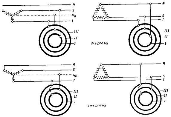
Bild 2 Schema der Elektrodenanschlüsse Elektrodendurchlauferhitzer
