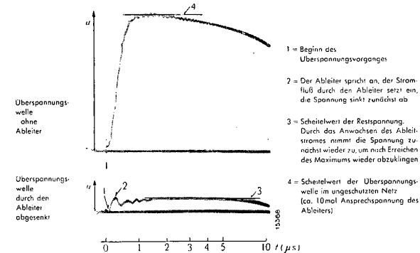
Bild 4 Schutzwirkung des Überspannungsableiters
