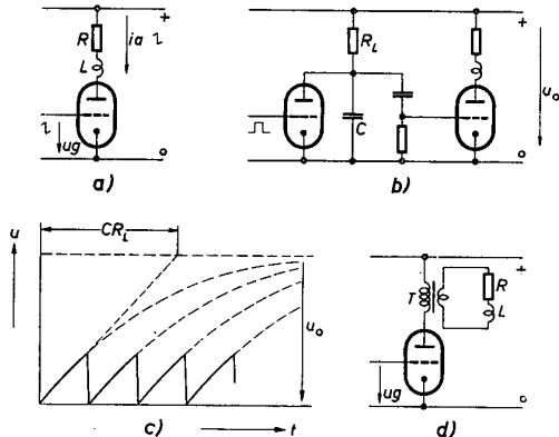
Bild 1 Grundschialtung der Vertikalablenkung
