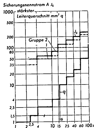
Bild 12 Kurzschlußschutzsicherung für stärksten Anschlußquerschnitt
