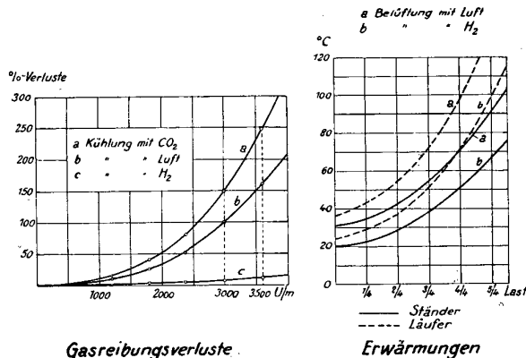
Bild 1 Gasreibungsverlust- und Erwärmungsdiagramme an einem 10 MVA-Versuchsgenerator
