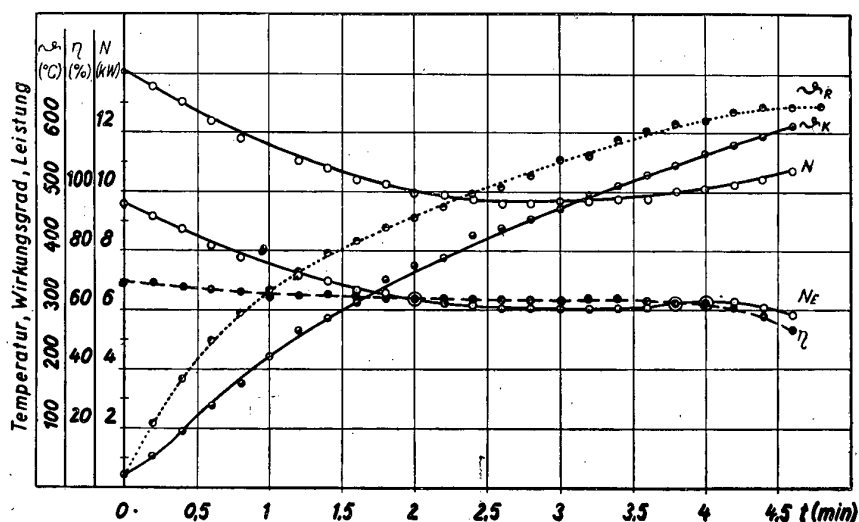
Bild 4 Erwärmungsschaubild eines Einsatzes von 80 mm \phi , 95 mm Länge: \vartheta_R = Randtemperatur, N = aufgenommene Leistung, \vartheta_K = Kerntemperatur, N_E = Einsatzleistung
