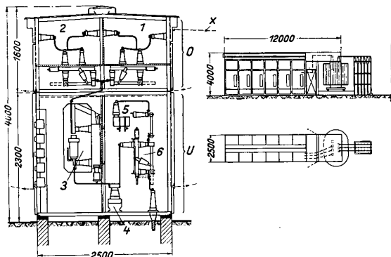
Bild 12 Hochspannung-Schrankanlage Reihe 20 mit Doppelsammelschienen
