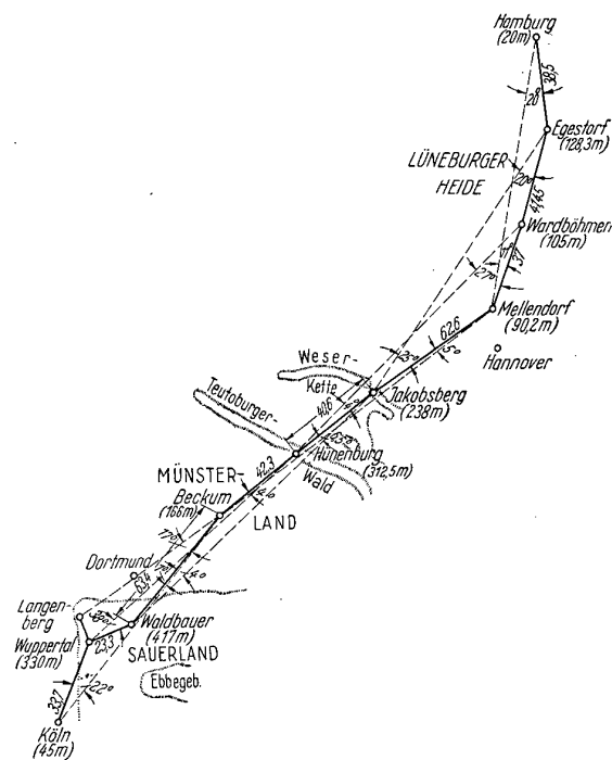
Bild 6 Nordwestdeutsches dm-Fernsprechneitz Kritische Überreichweiten-Winkel
