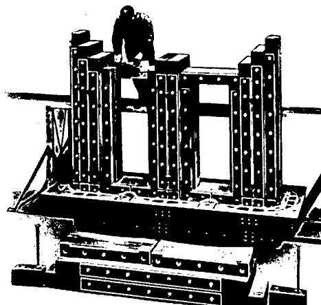
Bild 3 Rahmenkern während des Einschachtelns (SSW)
