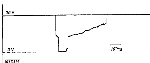
Bild 7. Spannungszoszillogramm (schematisch). Die Spannung fällt durch das Einschalten mit einer leichten Verzögerung durch den schwach markierten Einschaltlichtbogen von 36 auf 0 V. Der Kontakt bleibt \approx 10^{-4} s geschlossen. Beim Öffnen bilden sich eine kleine Schmelzstufe sowie anschließend unregelmäßige Öffnungsfunken von \approx 5 \cdot 10^{-4} s Dauer aus.
