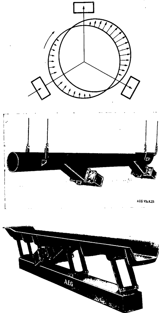
Bild 6 Technische Ausführungsformen von Schwingantrieben: a) Schema eines Bunkerantriebs; b) freischwebende Förderrinne mit Doppelantrieb; c) lenkgeführte Förderrinne mit Leitträger
