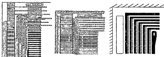
Bild 6 Drei Arten der Hauptisolation von Großtransformatoren: Links: Durch Hülsen und Kappen getrennte Ölstreifen Mitte: Isolierwickel aus ölprägniertem Papier und mit gespreizten Enden (BBC) Rechts: Isolierwickel bei Lagenwicklung mit einfach umgelegten Enden (Gen. Electric)
