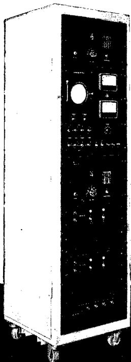
Kathodenstrahl-Oszillograph mit 2 Strahlen und 2 Zeitablenkgeräten für die Registrierung von einmaligen Vorgängen (Stosspannungen). Registriergeschwindigkeit bis 3000 km pro Sekunde.
