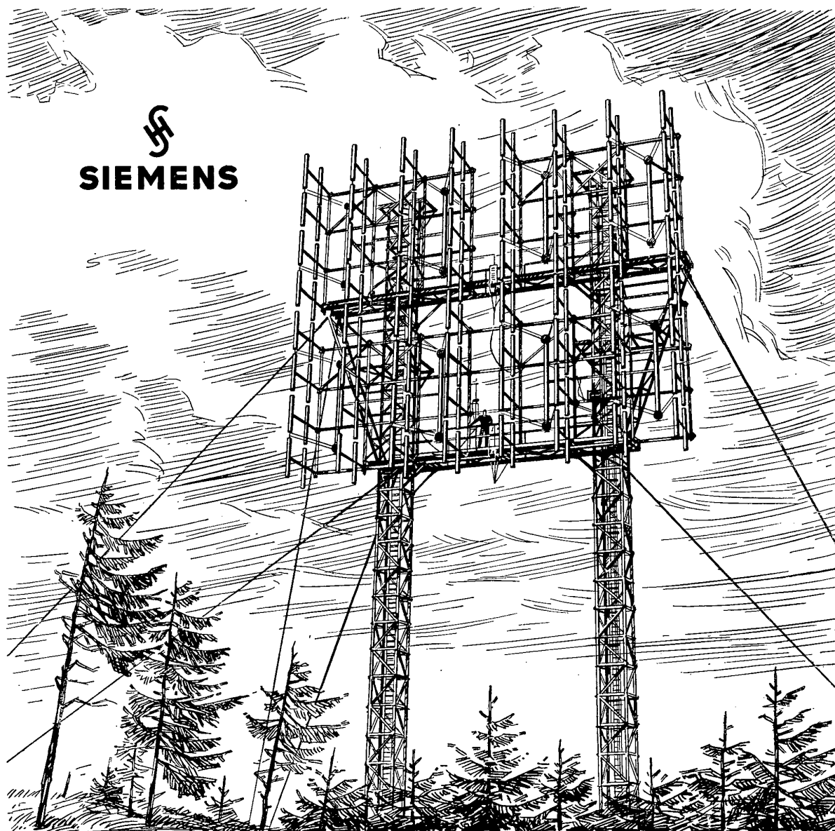
Breitband-Antennenfeld einer Meterwellenfunkbrücke
