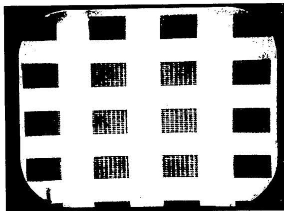
Bild 4 Fernseh-Prüfender CM 2657; gekreuzte Balken und Linien
