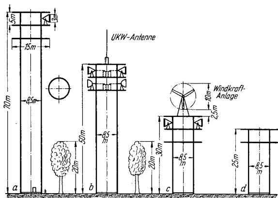
Bild 1 Türme für Richtfunkanlagen a) 70 m-Turm, b) 50 m-Turm, c) 30 m-Turm, d) 25 m-Turm
