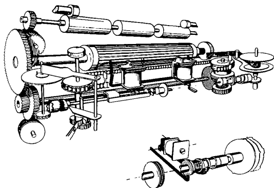
Bild 2 Prinzip der Aufzeichnung beim Blattschreiber SH
