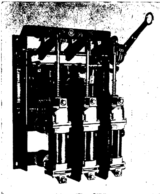
Bild 6: Druckausgleichschalter, Reihe 10, 400 A, 50 MVA von Voigt & Haeffner
