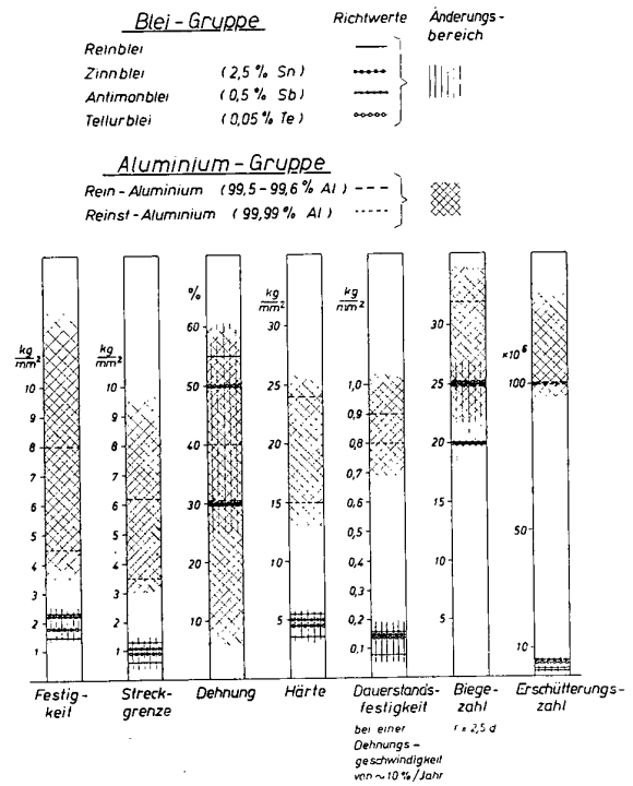
Bild 1 Vergleich der technologischen Eigenschaften von Kabelmantelwerkstoffen auf Blei- und Aluminiumbasis
