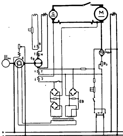
Bild 8 Leonard-Fördermaschine. Prinzipschaltplan
