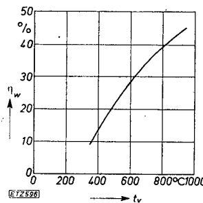
Bild 4. Einfluß der Frischgastemperatur auf den wirtschaftlichen Wirkungsgrad.
