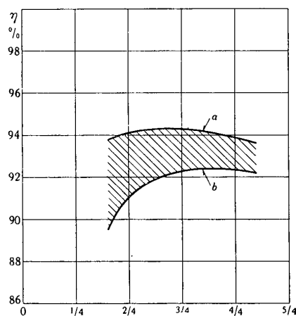
Bild 1 Wirkungsgrade des Frequenzumformers, a) mit Wasserstoffkühlung, H_2 -Überdruck 350 mm WS b) mit Luftkühlung.
