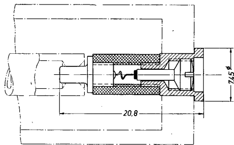
Bild 1 Dezimeterwellendetektor
