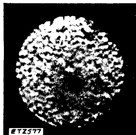
Bild 8. Kontaktoberfläche (Kathode) nach 5,4 \cdot 10^6 Schaltungen, 36 V, 4 A; Wolfram mit gleichmäßiger Faserstruktur, ungeätzt ( V = 9 ).
