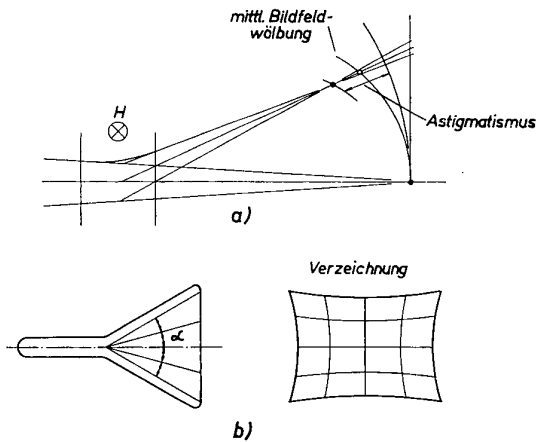
Bild 9 Elektronenoptische Fehler der Ablenkfelder
