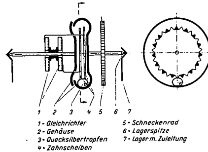
Bild 7 Quecksilber-Kontaktdose als Umschalter mit Gleichrichterplatten
