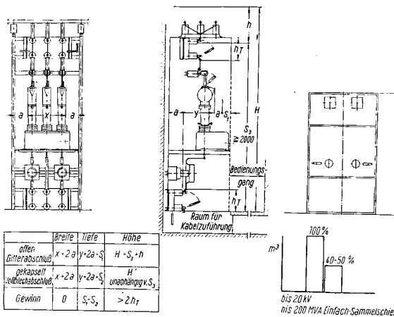
Bild 2 Raumbedarf von Schaltanlagen, offene und gekapselte Bauform
