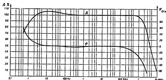
Bild 8 Elektronenstrahl-Oszillograph GM 5653; Verstärkung und Phasenwinkel zwischen 1 Hz und 7 MHz
