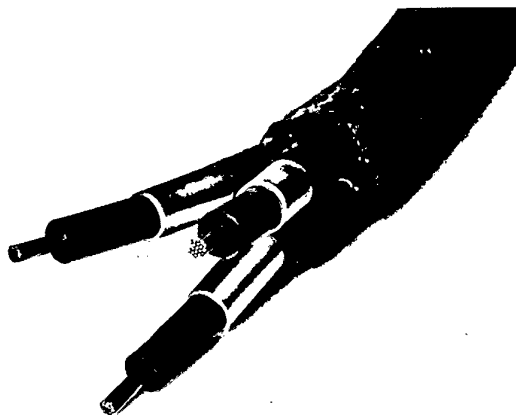
Bild 5 Dreimantelkabel mit Aluminiummantel, 30 kV, 3 × 50 mm 2 Cu
