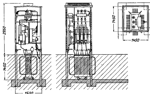
Bild 11 Netztransformatorenstation als Hochspannung-Schrankanlage ausgebildet mit im Erdreich eingebettetem Trafo
