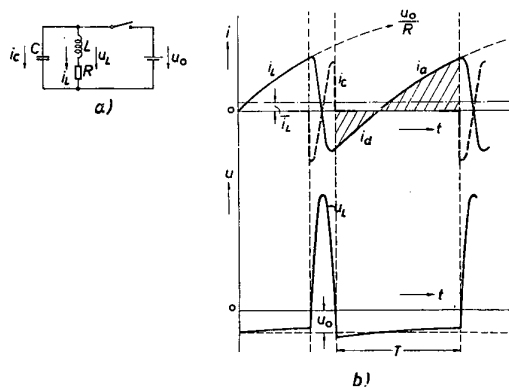
Bild 5 Grundschialtung für die Horizontalablenkung
