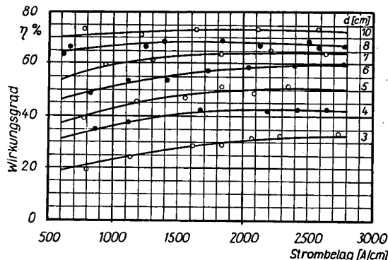
Bild 2 Abhängigkeit des Wirkungsgrades vom Strombelag A bei verschiedenen Einsatzdurchmessern. Einsatz: Werkzeugstahl mit 0,61 % C-Gehalt, \alpha = 30 \dots 100 mm \phi , Länge l = 1,066 d + 10 [mm]
