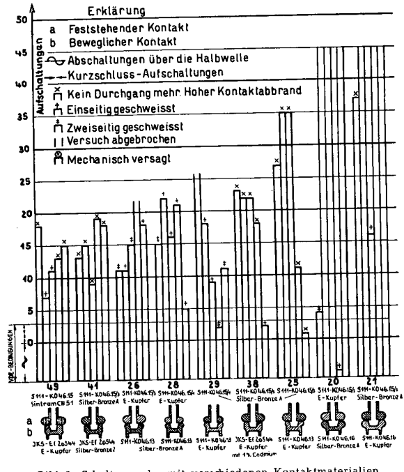
Bild 6 Schaltversuche mit verschiedenen Kontaktmaterialien und -formen
