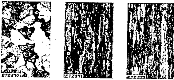
Bild 1. Rekristallisiertes Wolfram, anodisch geätzt ( V = 70 ). Bild 2. Gehämmertes Wolfram, anodisch geätzt ( V = 70 ). Bild 3. Gezogenes Wolfram, anodisch geätzt ( V = 70 ).
