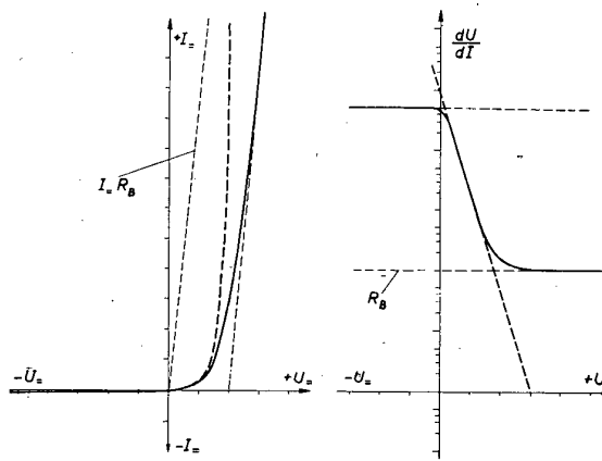
Bild 2 Detektor-kennlinien
