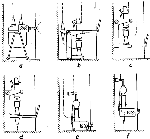
Bild 1 Innenraum-Expansionschalter, Entwicklung der Bauform
