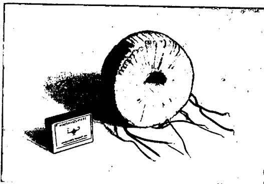
Bild 11 Bewickelter Doppelkern eines Transduktors für 75 W
