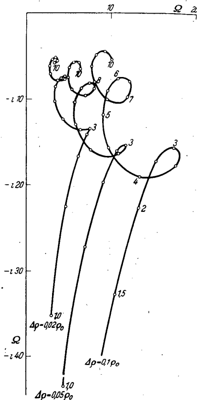
Bild 8 Ortskurve des Speisespalt-Scheinwiderstandes der Ringspaltantenne. Spaltbreite \Delta\rho = 0,1\rho_0 rechte Kurve, Spaltbreite \Delta\rho = 0,05\rho_0 mittlere Kurve, Spaltbreite \Delta\rho = 0,02\rho_0 linke Kurve; ..... homogene Feldverteilung
