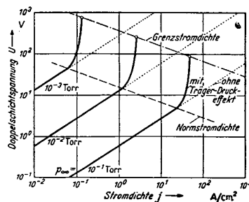
Bild 4 Doppelschichtkennlinien mit und ohne Druckeffekt der Ladungsträger
