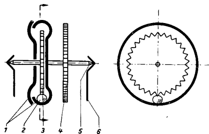
Bild 1 Grundform der Quecksilber-Kontakt-dose
