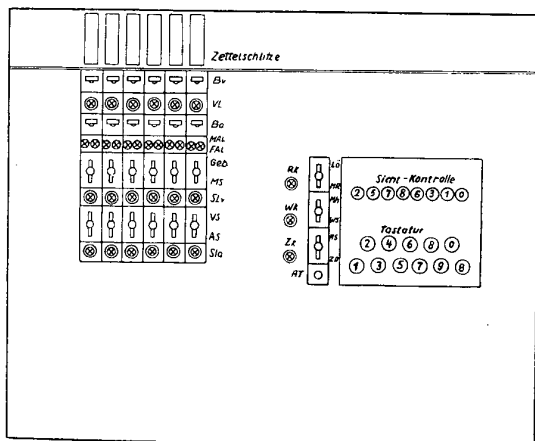
Bild 8 Schrankförmiger Stichleitungs-Fernplatz (Draufsicht)
