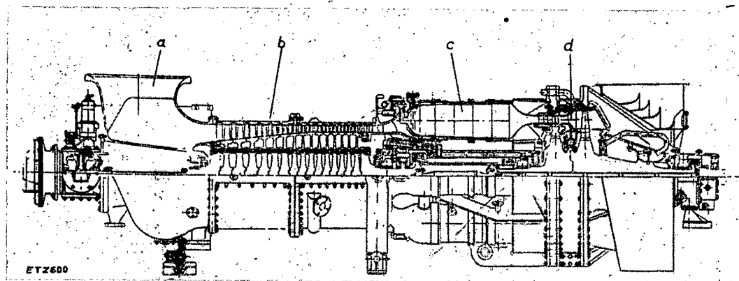
a) Kompressoransaugstutzen b) Kompressor c) Brennkammern d) zweistufige Gasturbine Bild 8. Längsschnitt durch eine 3500 kW-Gasturbinenanlage der General Electric Co.
