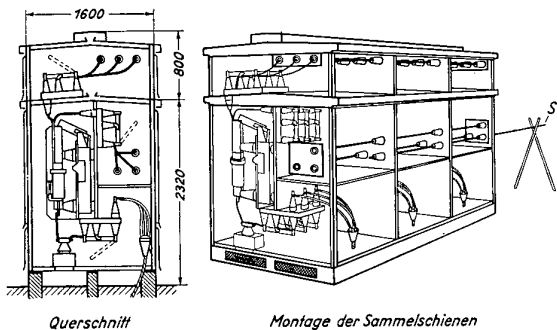
Bild 9 Nachträgliches Einschieben der Sammelschienenleiter nach Zusammenbau der einzelnen Schränke am Montageort
