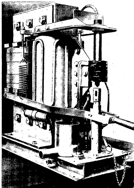
Bild 5 Industrielle Netzfrequenz-Induktionsglühanlage zur Erwärmung von Schließringen. Schließringmaße: 25,7 x 34 mm \phi , 57 mm Länge
