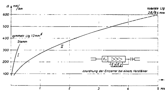
Bild 5 Dämpfungsverlauf von symmetrischen und koaxialen Kabeln
