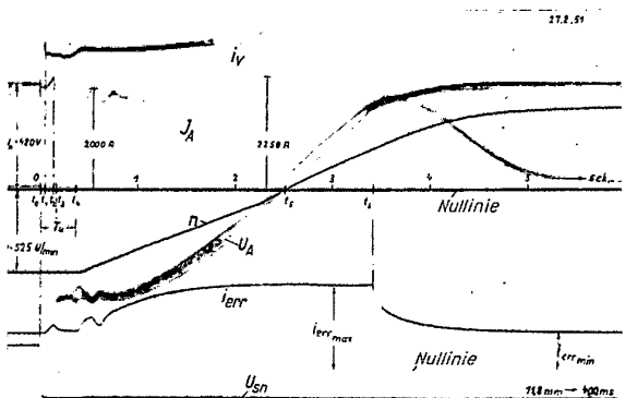
Bild 10 Umkehrvorgang mit Feldänderung bei einer 1000 kW-Großversuchsanlage
