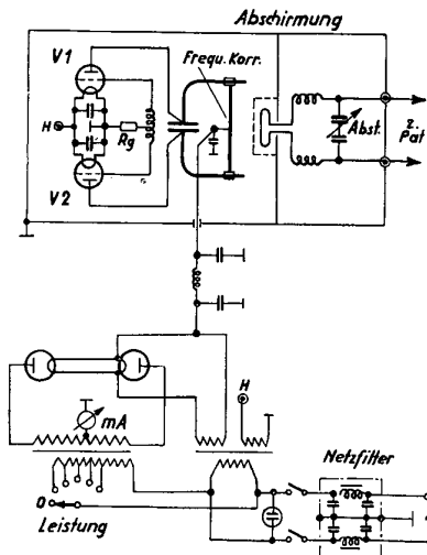
Bild 3 KW-Therapiegerät für 27,12 MHz \pm 0,6 % (funk-entstört und frequenzstabil)
