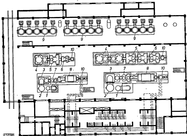
Bild 6. Grundriß des thermischen Kraftwerks in Beznau (Schweiz).
