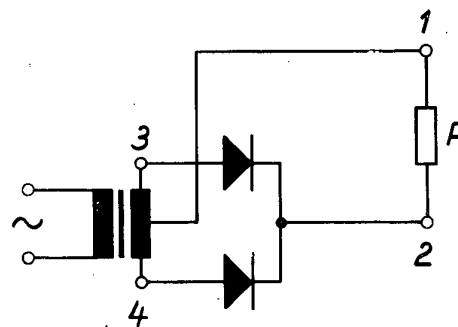
Bild 8 Grundschialtung des Transduktors mit Sättigungswinkelsteuerung für gleichgerichteten Arbeitsstrom
