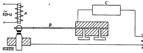
A Magnet B Blattfeder auf 100 Hz abgestimmt C Induktionsfreier Vorwiderstand Bild 6. Kontaktprüfgerät (schematisch).
