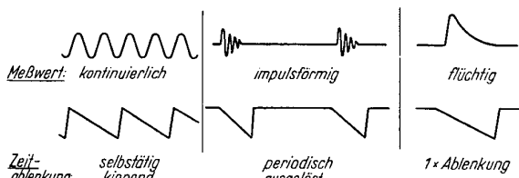
Bild 5 Verschiedene Betriebsarten des Zeitkreises
